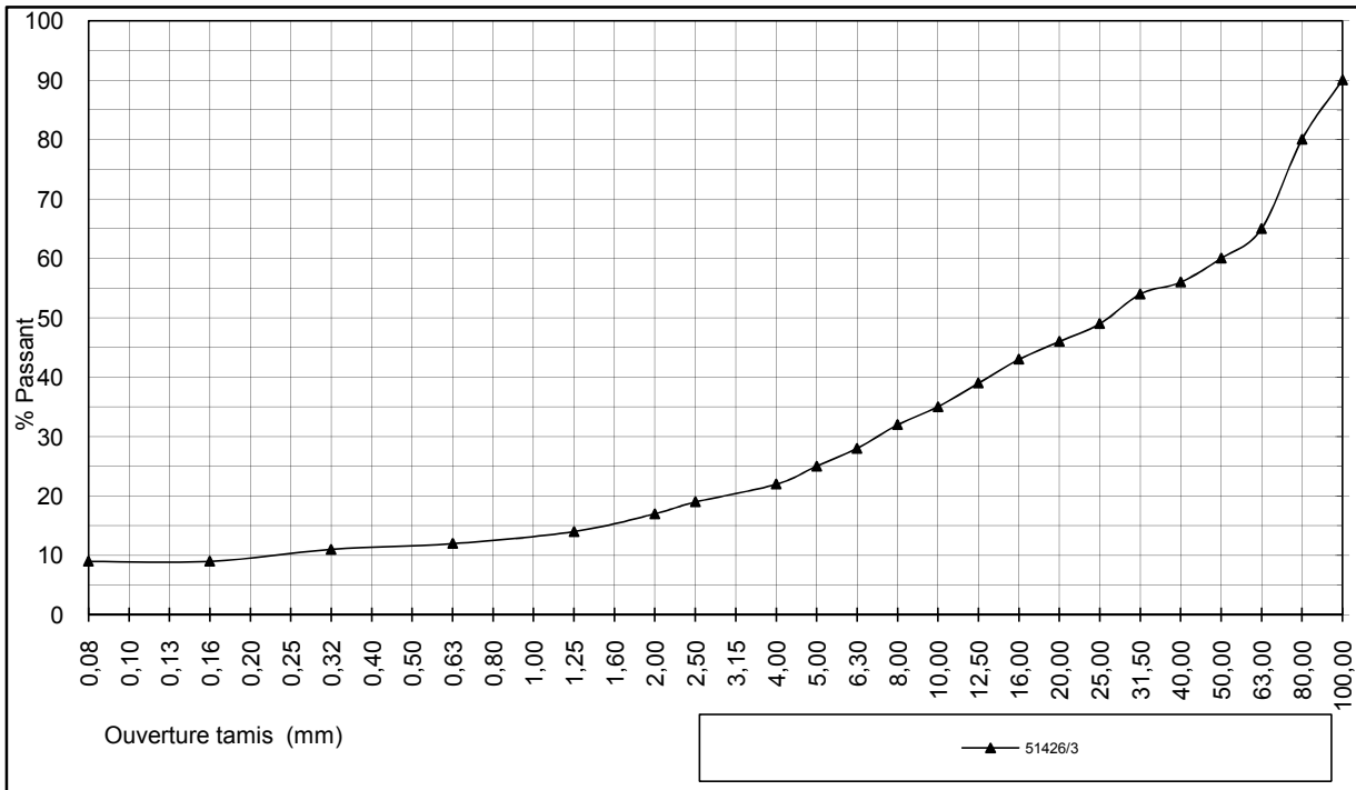
Figure 15 : Courbe cumulative de l'analyse granulométrique
