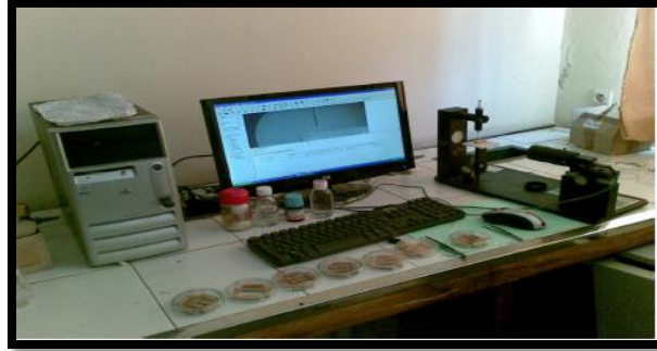
Figure. 4: Appareil d'angle de contact
