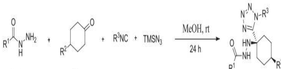
Schéma 13 * : Préparation de tétrazole par réaction « multi composants ».
