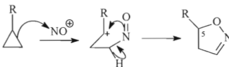
Schéma 19 : Formation de 2-isoxazolines par nitrosation du cyclopropane.
