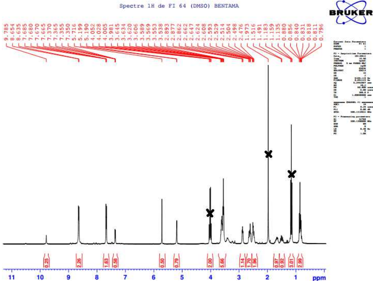
Figure 5 : Spectre de RMN 1 H du produit K.
