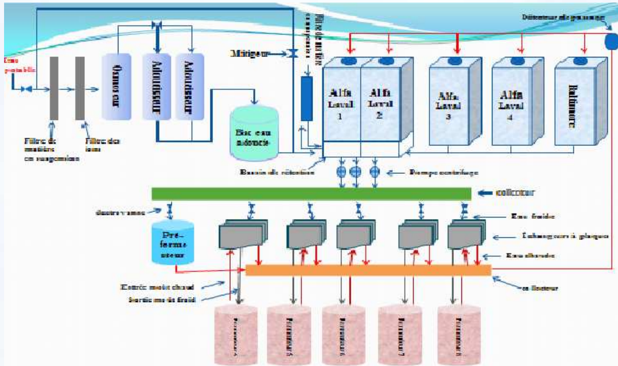
Figure 13: schéma du procédé de refroidissement.
