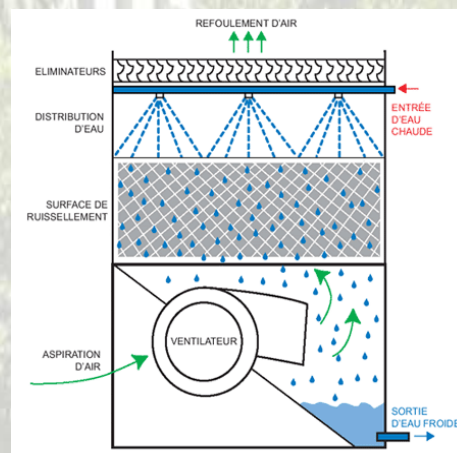
Figure 8 : tour à circuit ouvert.
