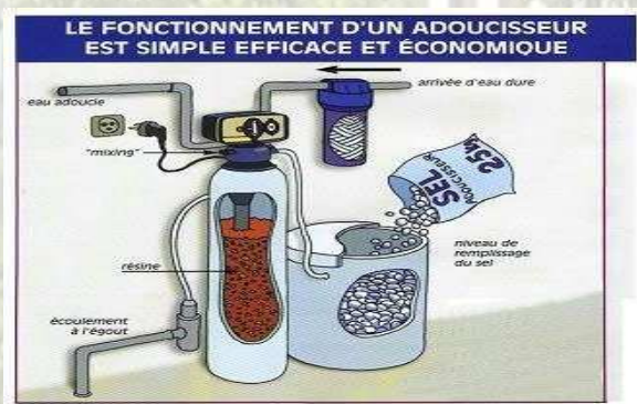
Figure 9: principe et fonctionnement d'un adoucisseur
