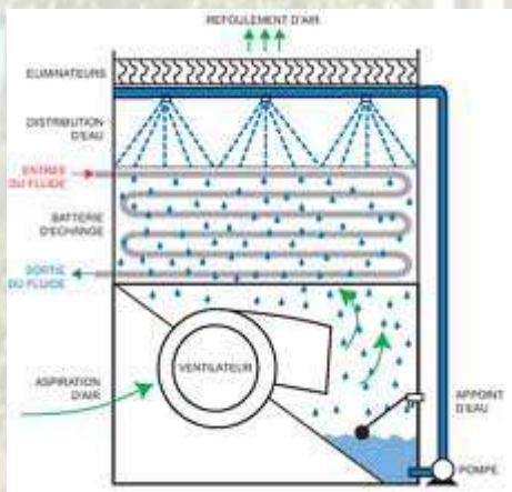
Figure 7 : tour à circuit fermé.
