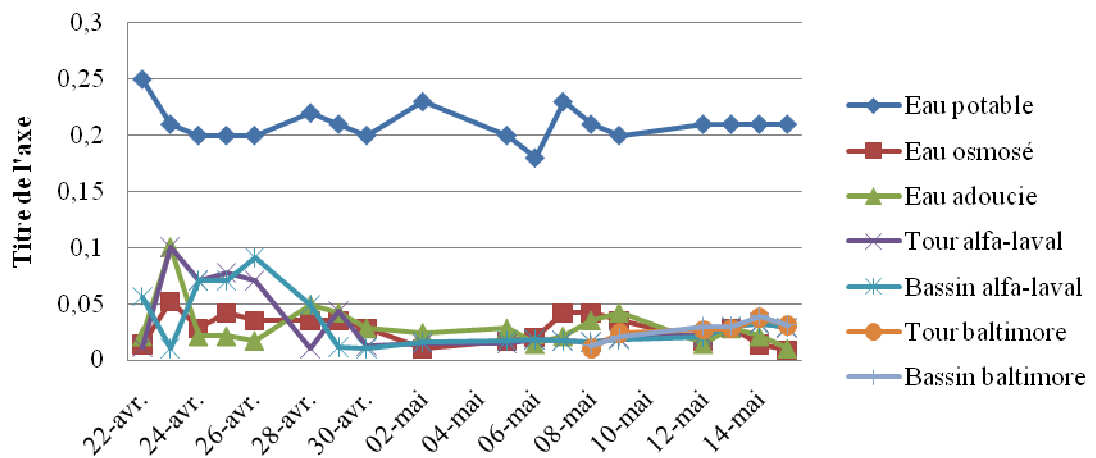
figure 20: [Cl - ] g/l des eaux en fonction des jours de prélèvements
