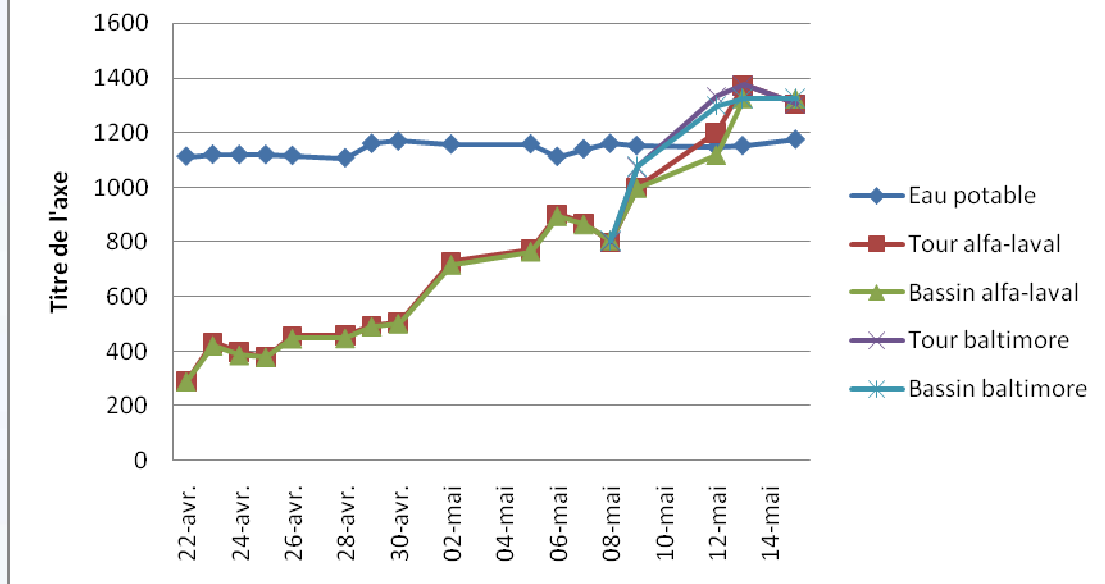
figure 14: conductivité de l'eau potable et des tours de refroidissement en fonction des jours de prélèvements
