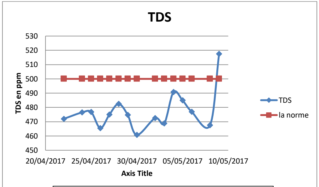
Figure 14 : variation de TDS au cours du temps
