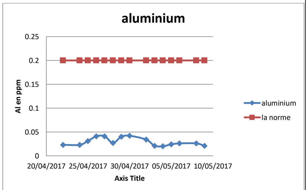
Figure 15 : variation d'aluminium au cours du temps
