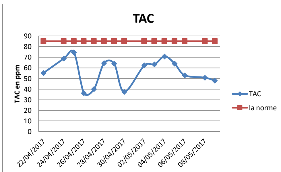
Figure 12 : variation de TAC au cours du temps
