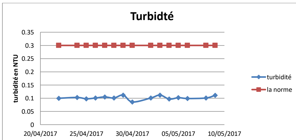
Figure 13 : variation de turbidité au cours du temps
