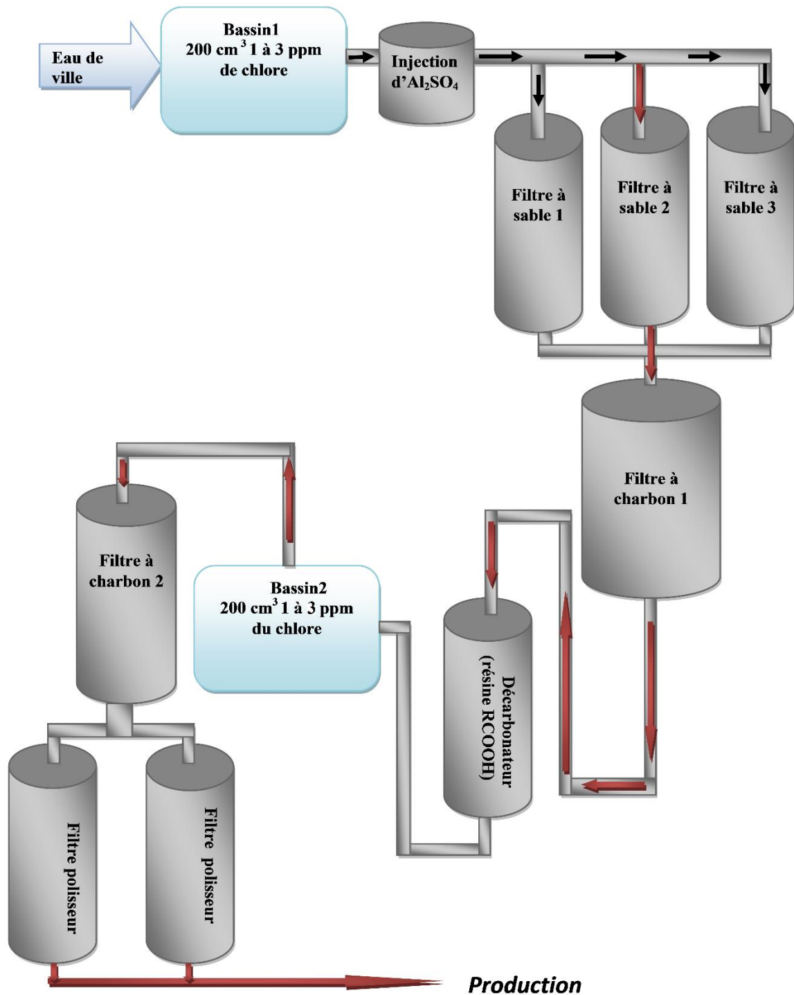
Figure 5 : Schéma de principe du traitement des eaux
