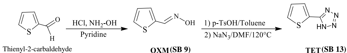
Figure 15 : Etapes de synthèse des produits OXM (SB9) et TET (SB13)
