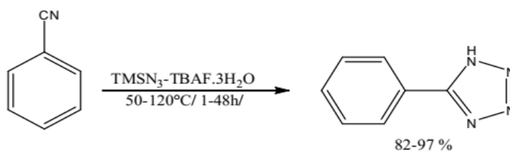
Figure 14 : Préparation de tétrazoles par l'azoture de triméthylsilyle sans solvant.
