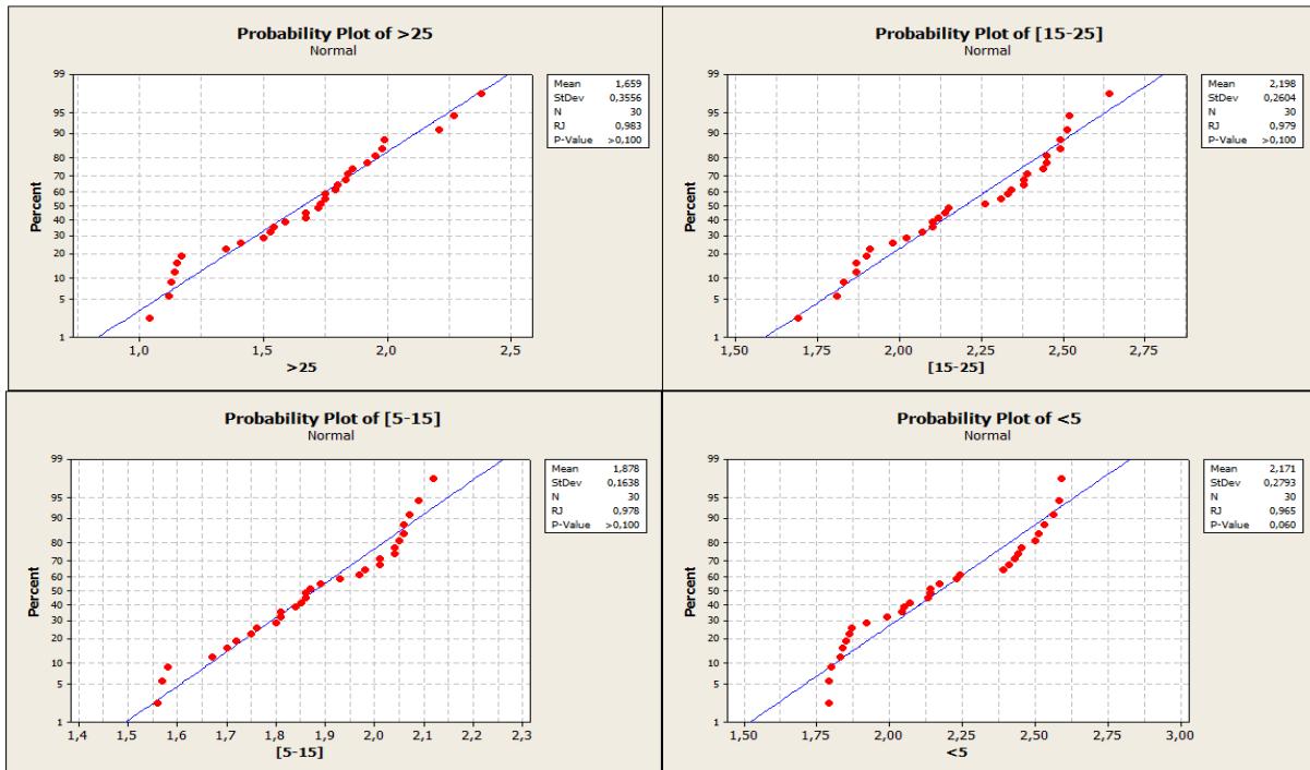
Figure20 : Représentation graphique de la normalité des résultats de CaO libre pour les différentes tranches du clinker : >25, [15-25], [5-15], <5
