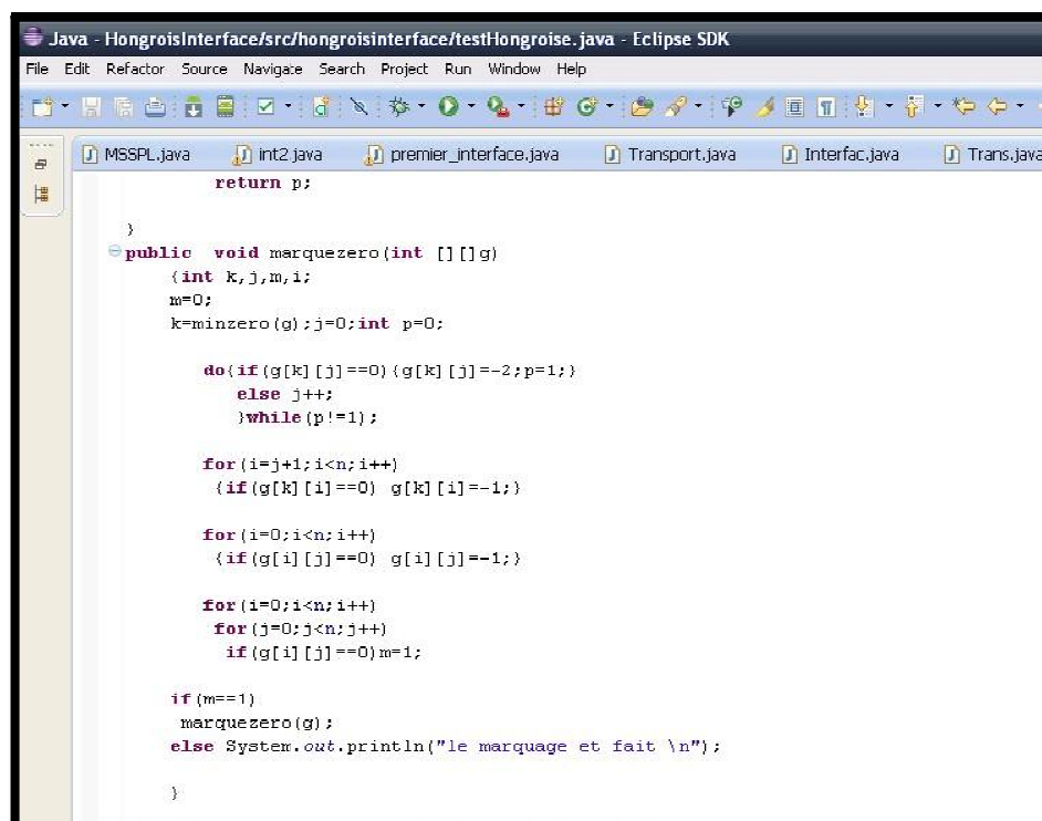
Figure 28 : La méthode marquezero.
