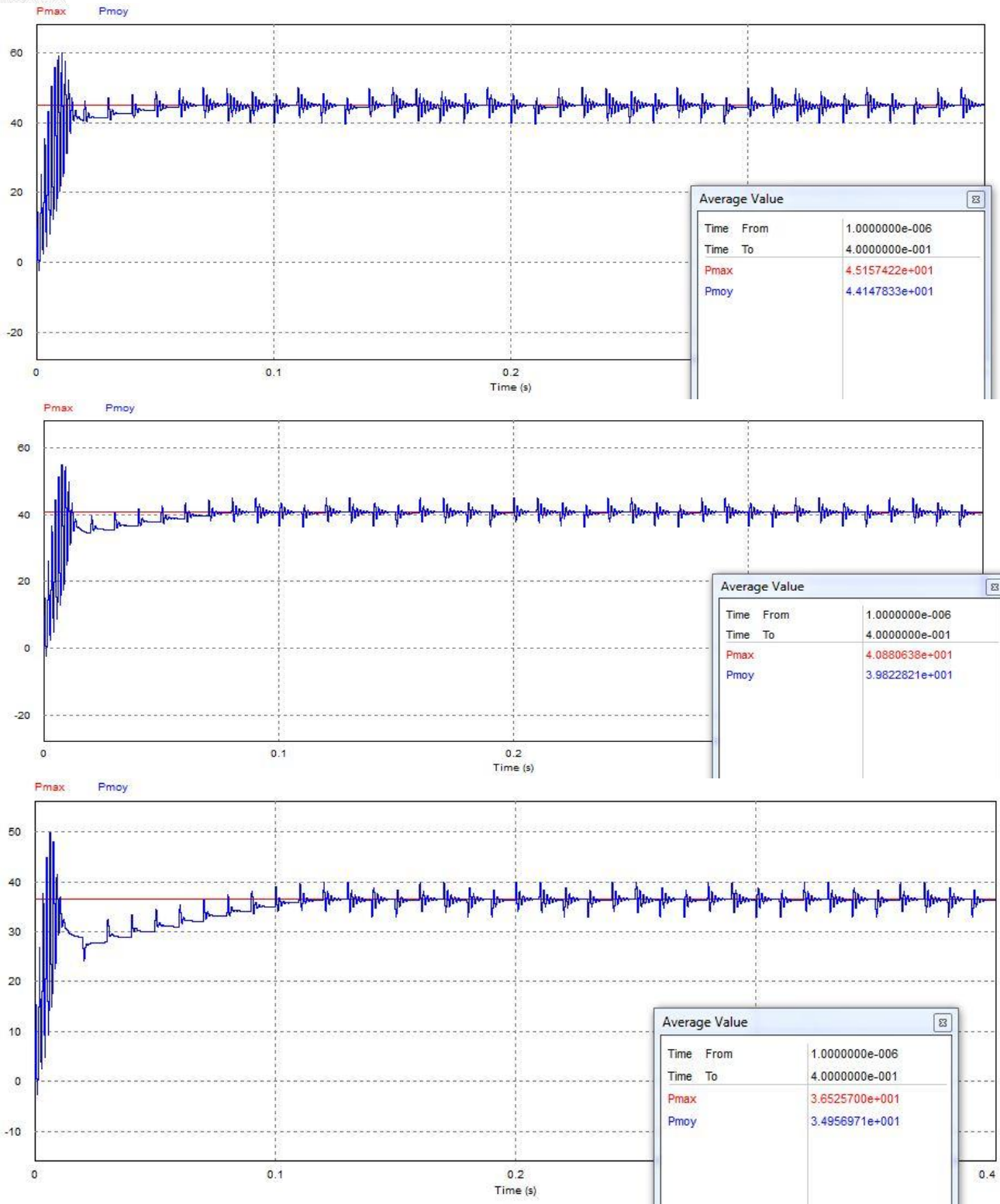
Figure 3.15 : performances de poursuite du MPP pour un ensoleillement de 800 W/m^2 et des températures de 40, 60 et 80 °C (du haut en bas respectivement).
