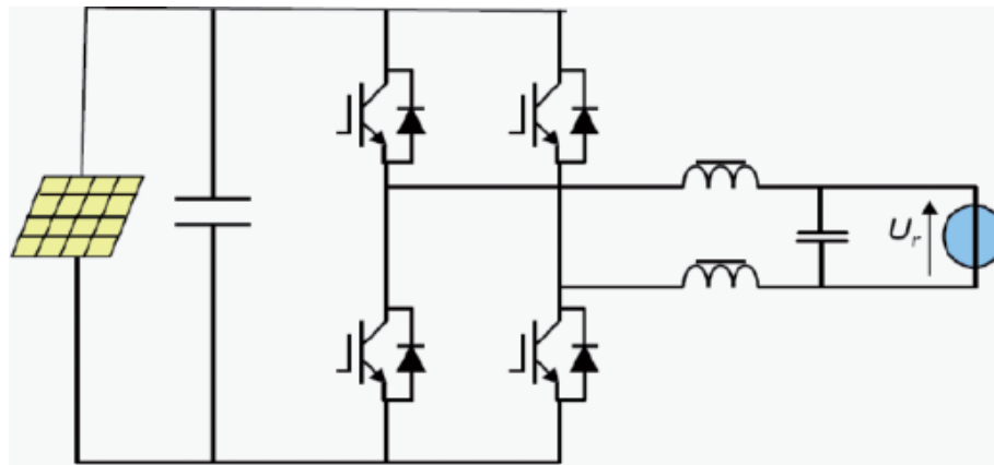
Figure 1.6 : onduleur sans transformateur.
