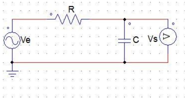
Figure 2.25 : schéma électrique d'un filtre passe bas RC.
