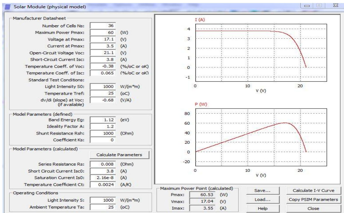
Figure 3.9: modèle d'un panneau solaire donné par le logiciel PSIM.
