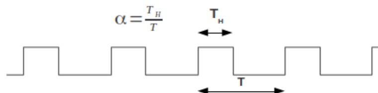
Figure 3.3 : signal rapport cyclique de la commande de l'interrupteur S ( \alpha = \frac{T_H}{T} étant le rapport cyclique).
