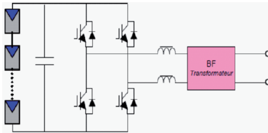
Figure 1.4 : onduleur en pont avec transformateur BF [3].
