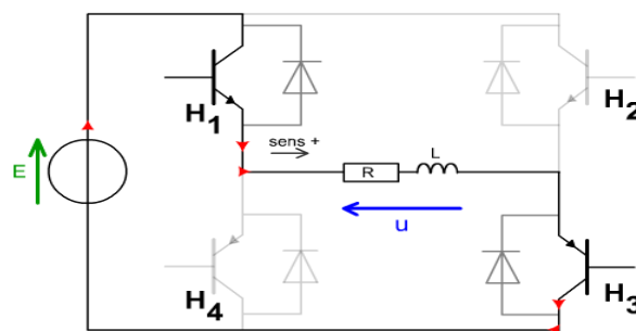
Figure 2.4 : interrupteurs H 1 et H 3 en conduction.
