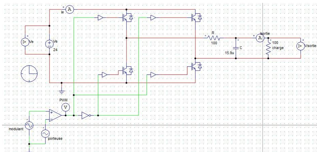
Figure 2.29 : onduleur avec filtre RC chargé par une charge résistive.
