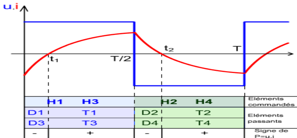
Figure 2.10 : formes de u(t) et i(t) à la sortie du pont.
