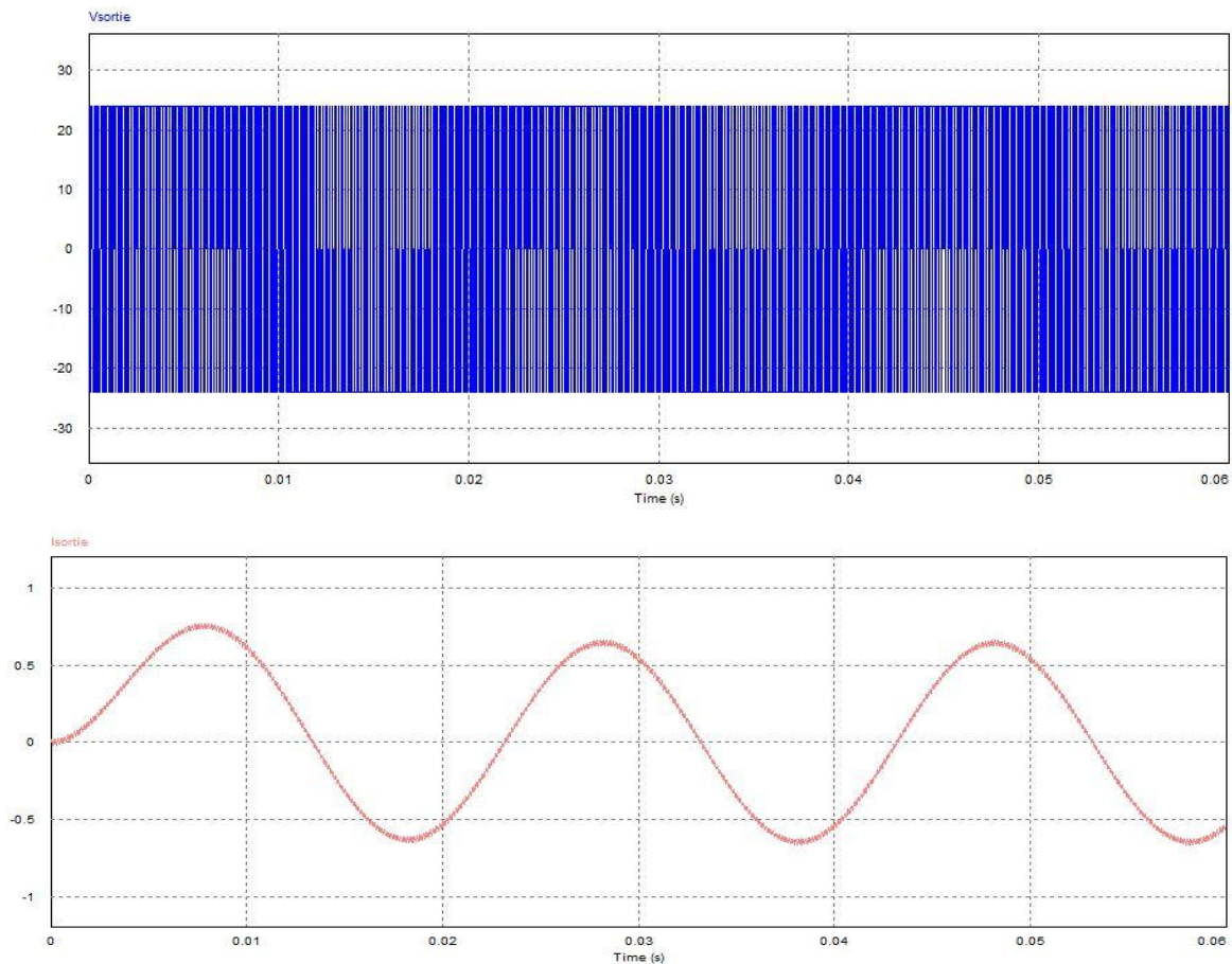
Figure 2.23 : tension et courant de sortie pour ( f_p=6 kHz, V_m=3 V).
