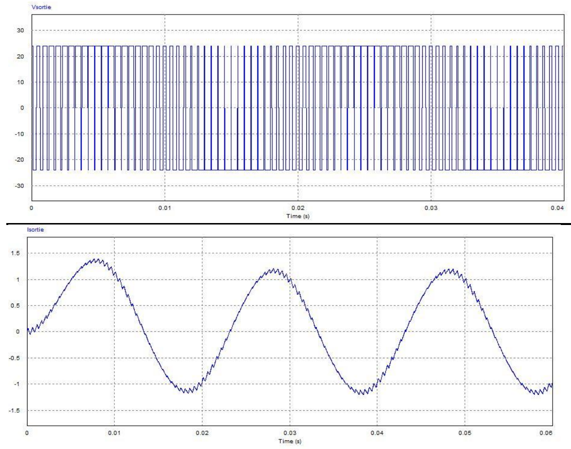
Figure 2.19 : allures tension et courant aux bornes de la charge.
