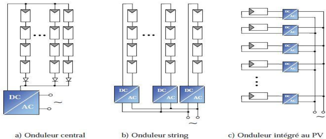
Figure 1.12 : schémas de principe de différentes topologies [4].
