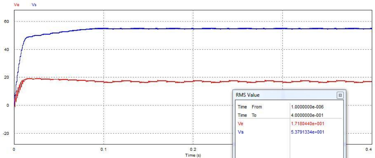
Figure 3.11 : tension d'entrée(en rouge) et de sortie (en bleu) du convertisseur DC-DC.
