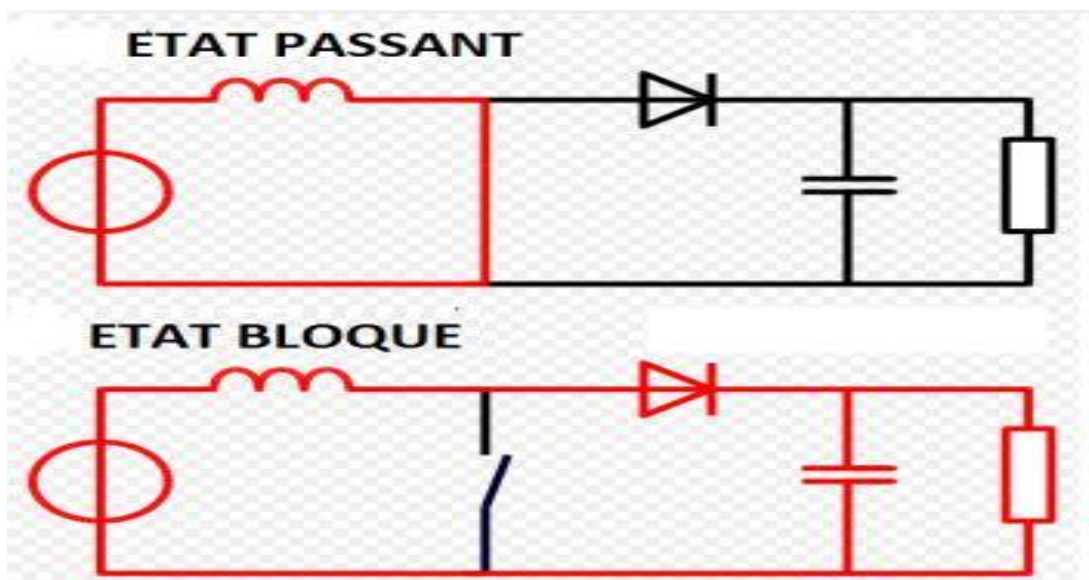
Figure 3.4 : configuration d'un convertisseur DC-DC suivant l'état de l'interrupteur.
