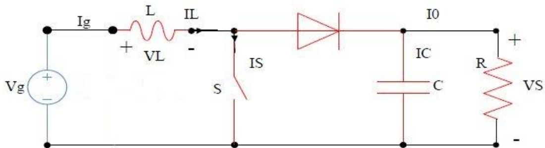
Figure 3.2 : schéma électrique de base d'un hacheur survolteur.
