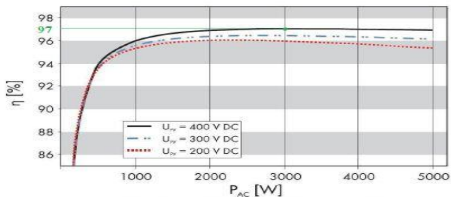
Figure 1.9 : courbe de rendement pour trois tensions d'entrée.
