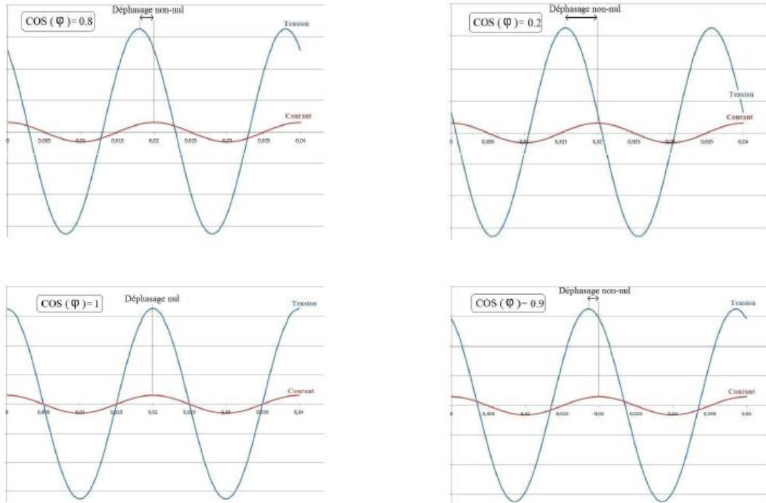
Figure 1.8 : déphasage entre courant et tension (facteur de puissance) [2].
