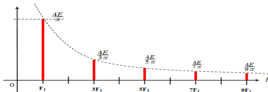
Figure 2.12 : spectre de fréquence de la commande pleine onde.
