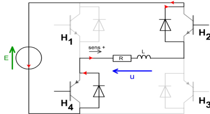
Figure 2.8 : deuxième phase de récupération.
