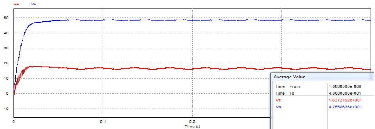
Figure 3.14 : allure de tension d'entrée sortie de la deuxième simulation
