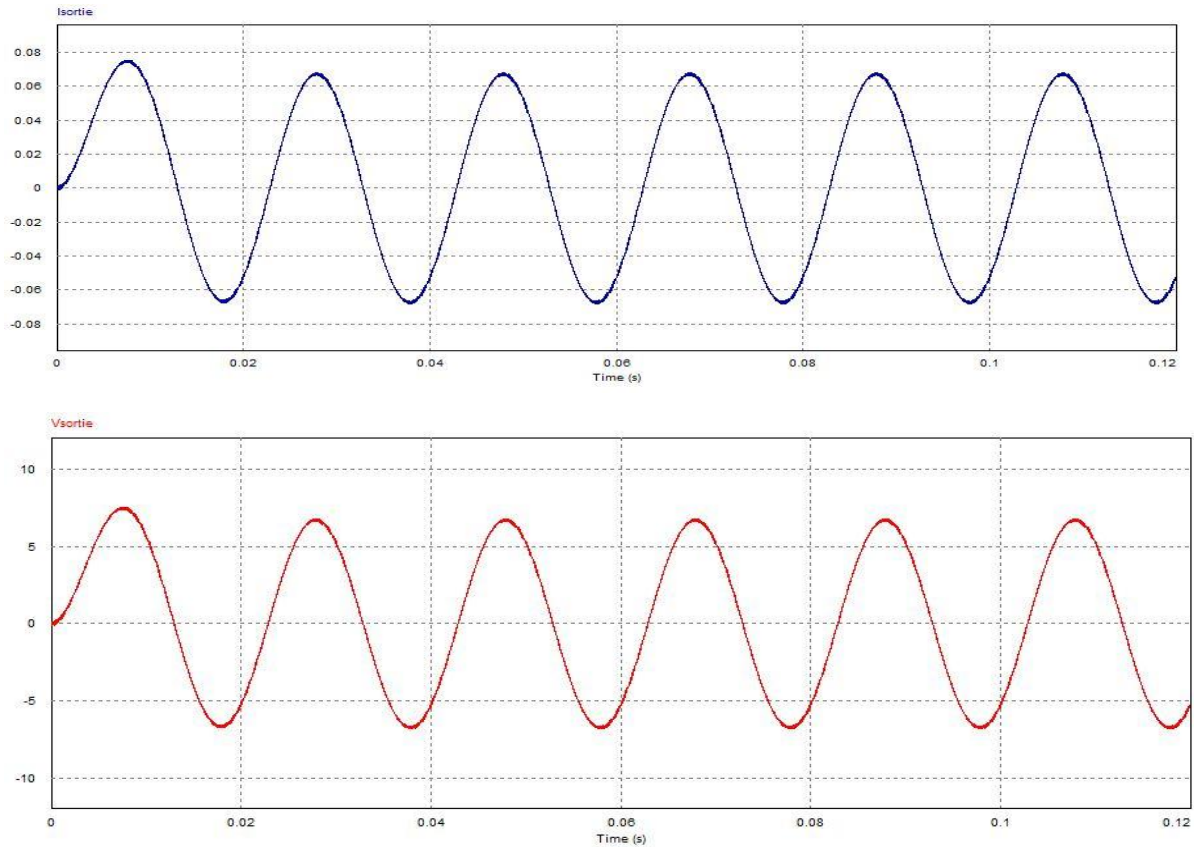
Figure 2.31 : tension et courant quasi-sinusoidaux de fréquence 50Hz.
