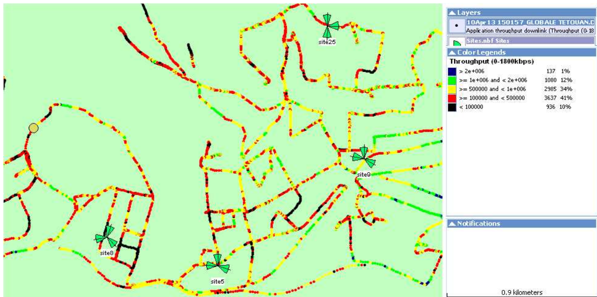
Figure 34: Le débit de la zone à problème 3
