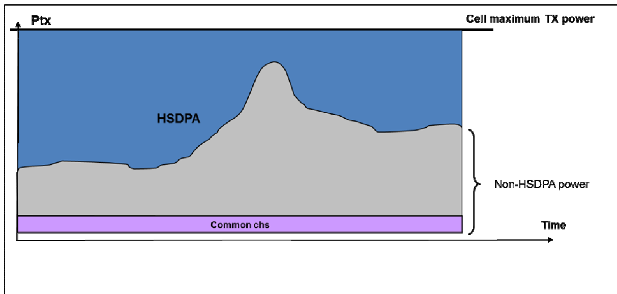
Figure 22: Allocation dynamique de la puissance HSDPA[7]
