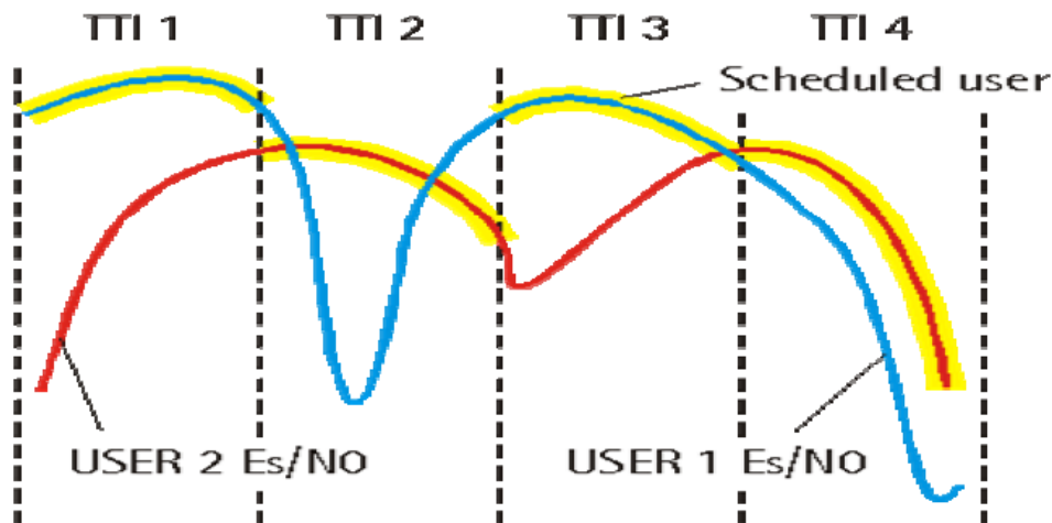
Figure 19 : Le principe de l'algorithme « Proportional Fair Scheduling ».
