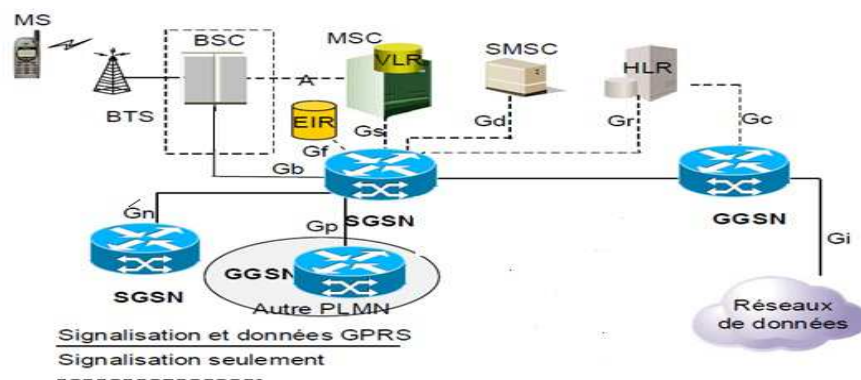
Figure 2 : Evolution de l'architecture de GSM vers GPRS [8]
