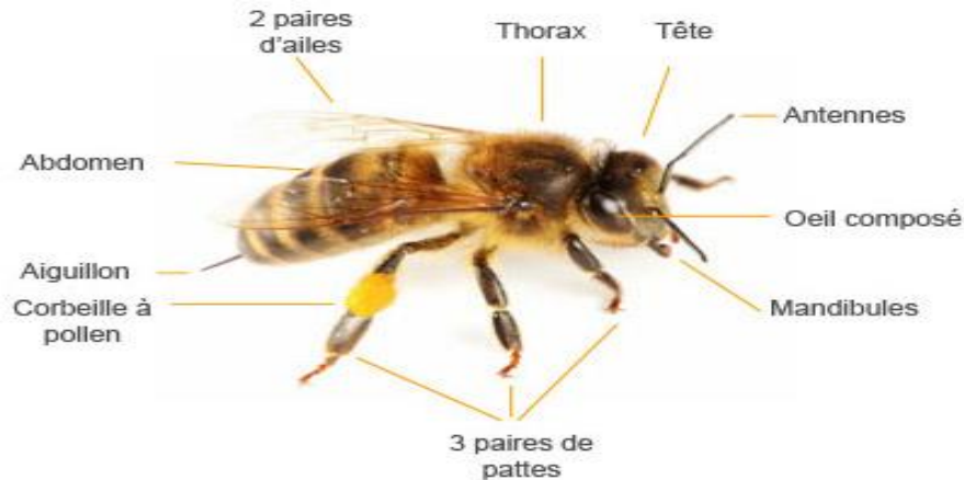
Figure 1 : Image montrant les différentes parties morphologiques d'une abeille
