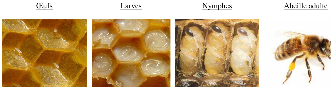
Figure 7 : Images montrant les différentes étapes de développement
