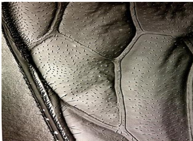
Figure 4 : Image montrant les nervures d'une aile (vue au microscope électronique X 65 fois).
