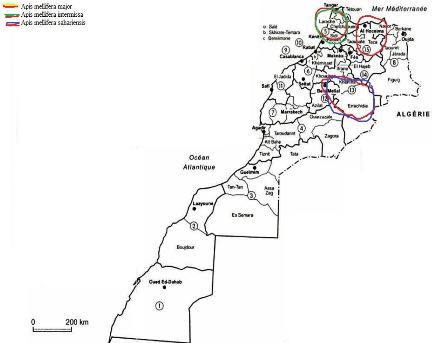
Figure 12: Répartition géographique des trois espèces d'abeilles au Maroc à l'échelle nationale.
