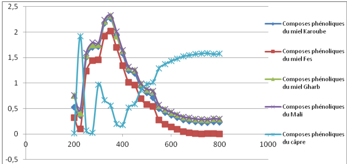
Figure 25 : Les spectres d'absorbance des composés phénoliques des miels étudiés D'après la figure ci-dessus, on constate que les miels absorbent plus dans l'invisible (200 et 400 nm) que dans le visible (400 et 800 nm).
