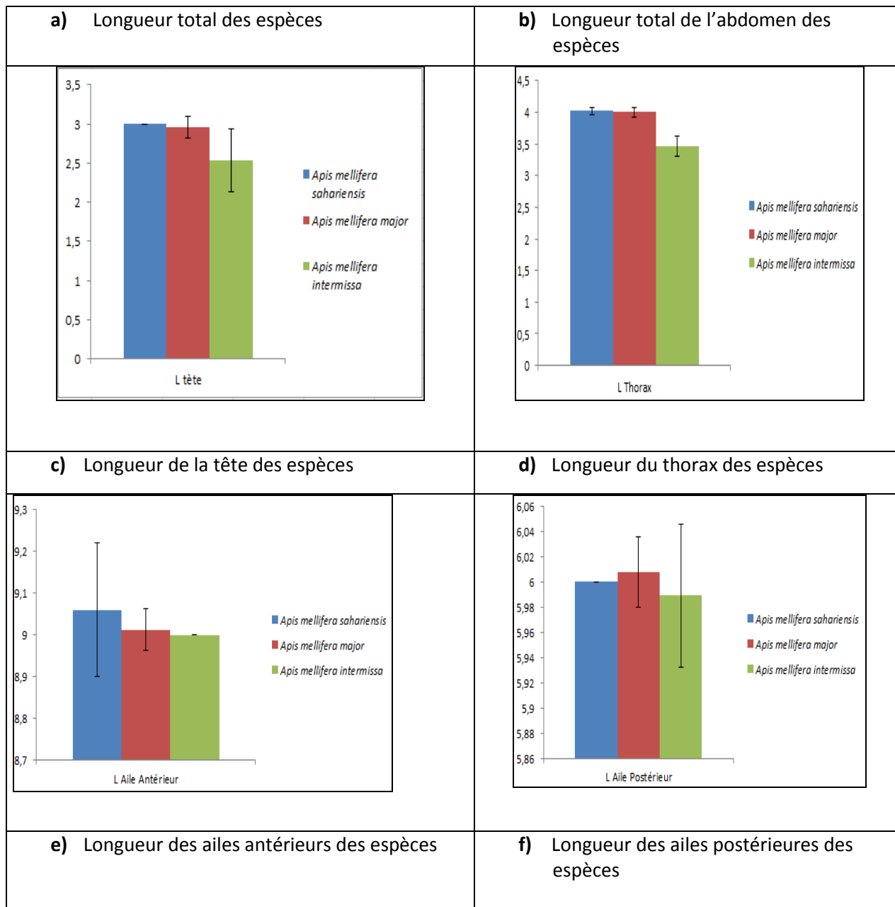
Figure 21 : Représentation graphique des différents paramètres étudiés chez les 3 populations d'abeilles a : LT, b : LT Ab, c : L Tête, d : L Th, e : L Aile Ant, f : L Aile Post.
