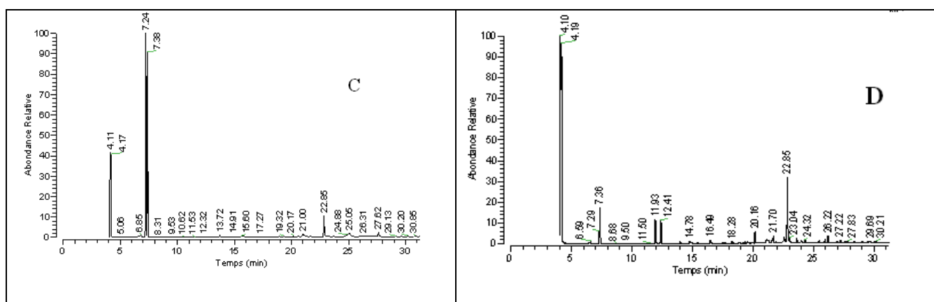
Figure 27 : Analyse CG des composés phénoliques présents dans échantillons C et D
