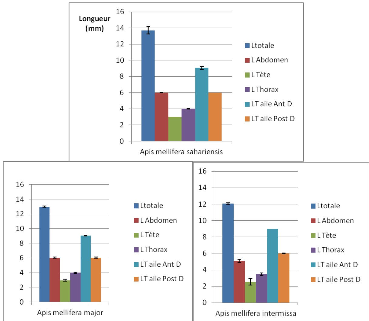
Figure 20 : Représentation graphique des différents traits morphologiques des 3 populations d’abeilles marocaines
