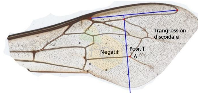
Figure 23 : Image d'une aile d'abeille montrant l'indice de la transgression discoïdale.
