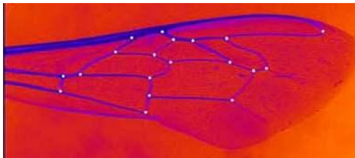
Figure24 : Image d'une aile d'abeille montrant les points de rencontres des nervures
