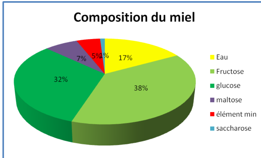
Figure 16 : Composition du miel (%)
