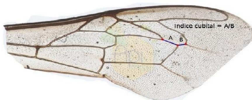
Figure 22 : Image d'une aile d'abeille montrant la nervure de la 3 ème cellule cubitale permettant le calcul de l'indice cubital (A/B)
