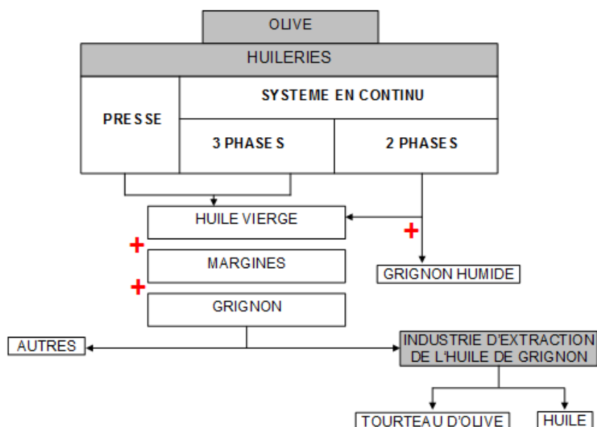
Figure 5 : Procédé général de production d'huile d'olive.
