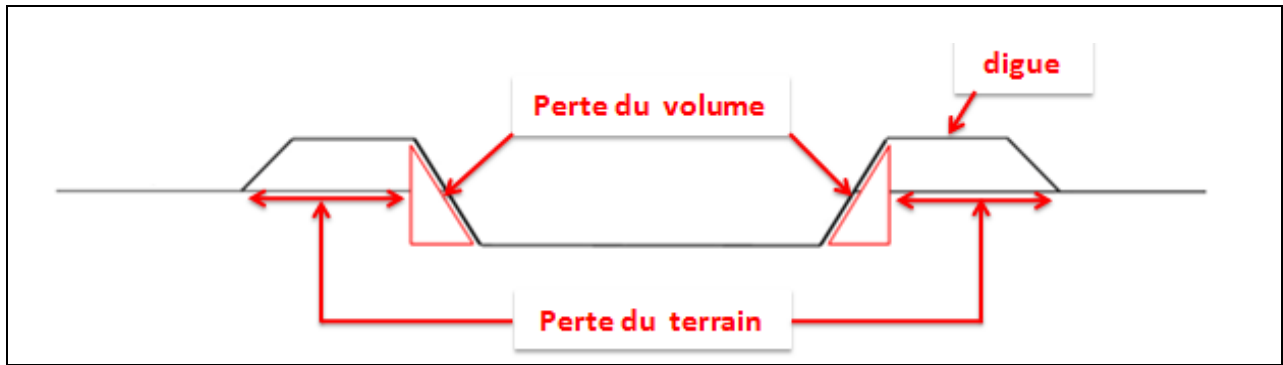
Figure 18 : Forme et pertes concernant les bassins d'évaporation avec fond argileux.
