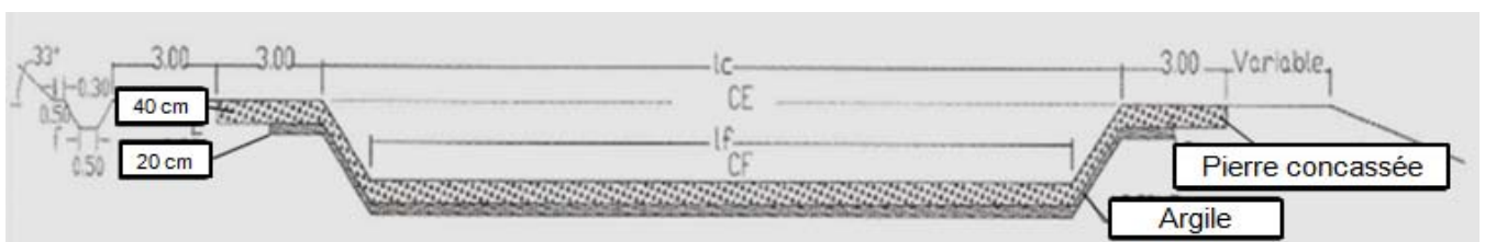
Figure 15 : Texture des bassins d'évaporation (ABHS 2011).
