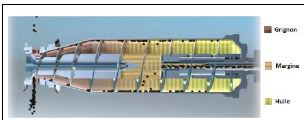
Figure 2 : Coupe transversale d'une centrifugeuse horizontale ( https://www.youtube.com/watch?v=zSL_-DcsjR4 ).
