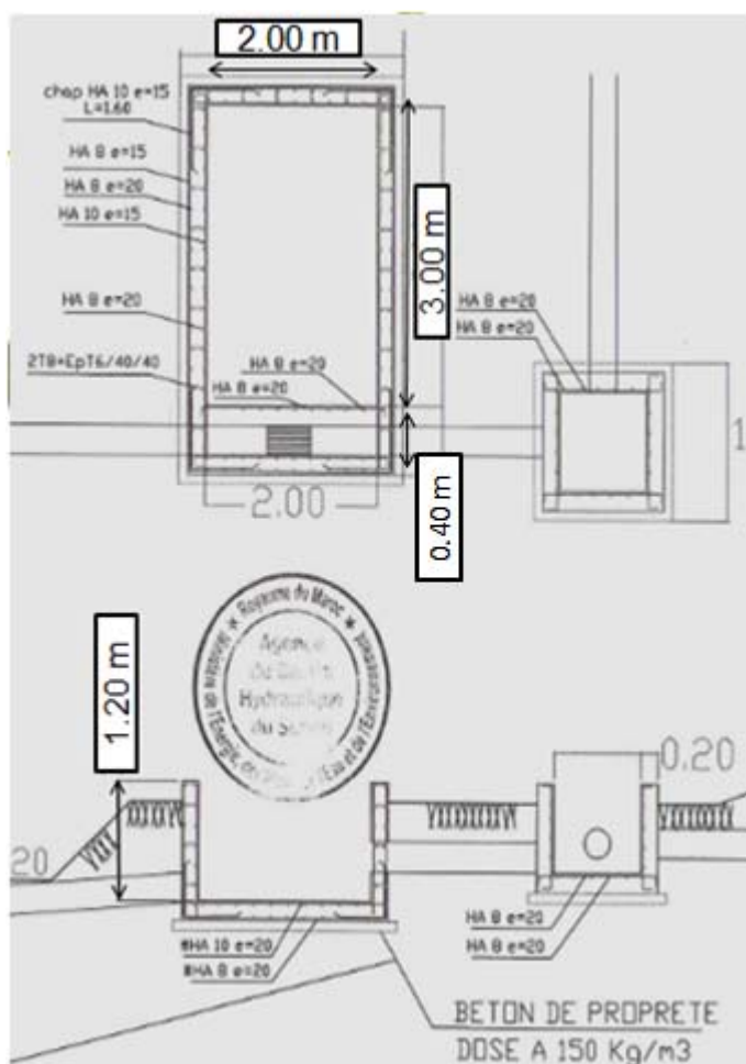
Figure 12 : Dimensionnement du Dégrilleur (ABHS 2011).
