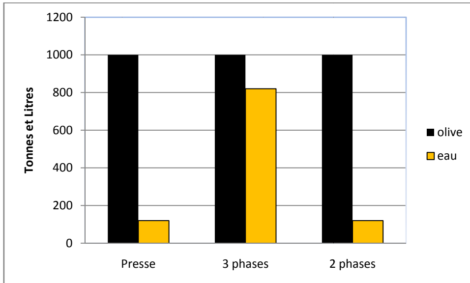
Figure 6 : Quantités des entrées dans chaque système.
