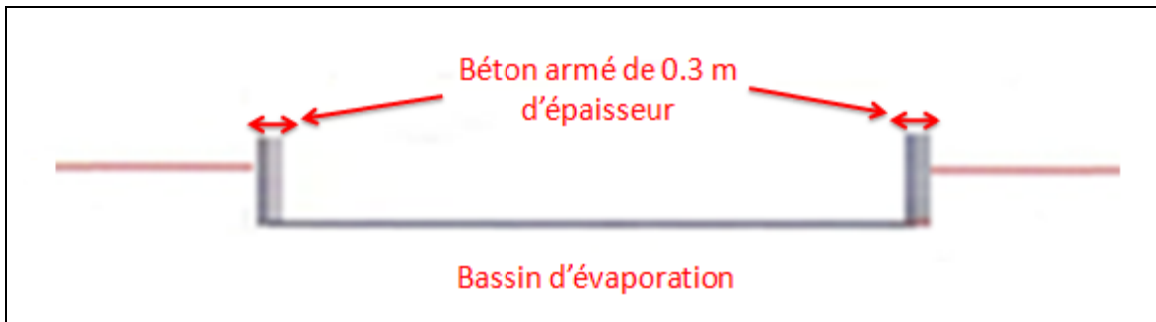
Figure 21 : Forme et texture les bassins d'évaporation proposés.
