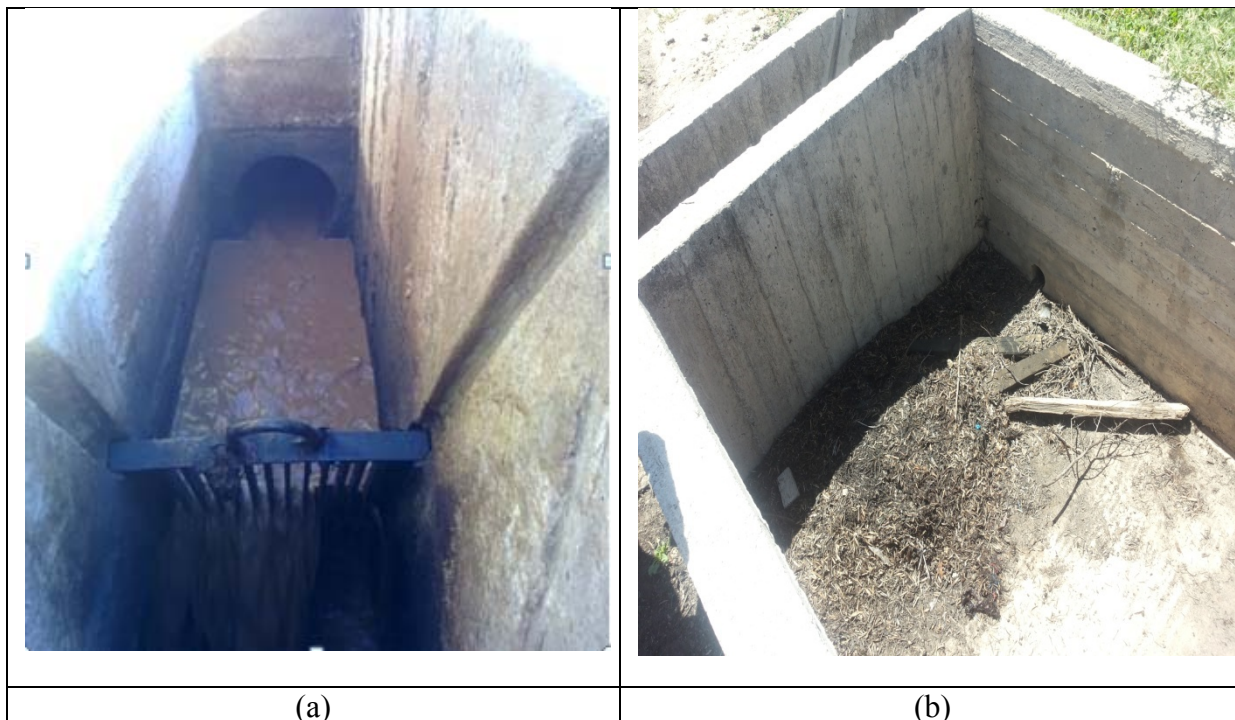
Figure 11 : (a) Dégrilleur (ABHS). (b) dégrilleur et bassin annexe (photo prise sur terrain le 8/5/2015).
