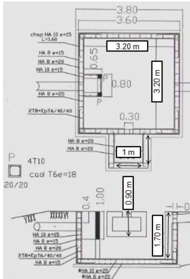
Figure 14 : Dimensionnement du déshuileur (ABHS, 2011).
