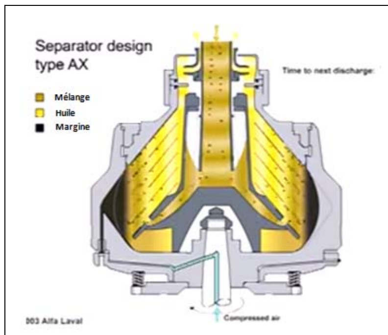
Figure 3 : Coupe transversale d'une centrifugeuse verticale ( https://www.youtube.com/watch?v=zSL_-DcsjR4 ).
