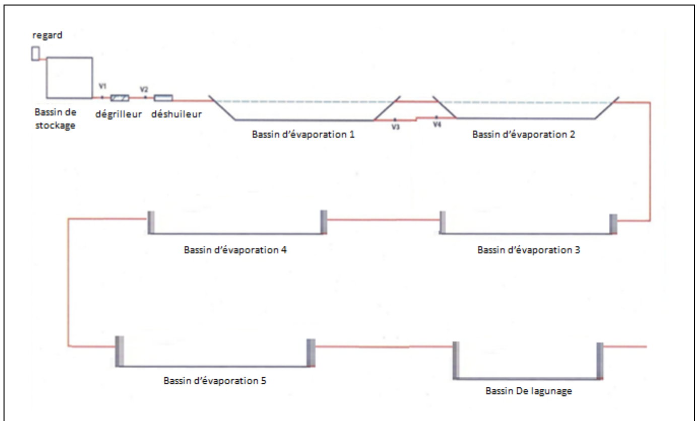
Figure 19 : Ensembles des constituants déjà existés et proposés de la station d'évaporation.
