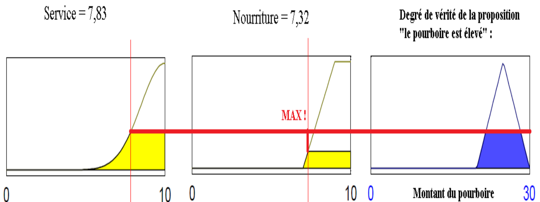
Figure 1.9: Exemple d'implication Floue avec conjonction OU traduite par un MAX
