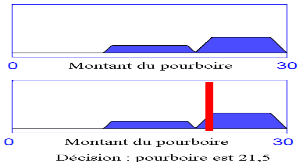
Figure 1.12: Defuzzification avec la méthode centre de gravité (COG)
