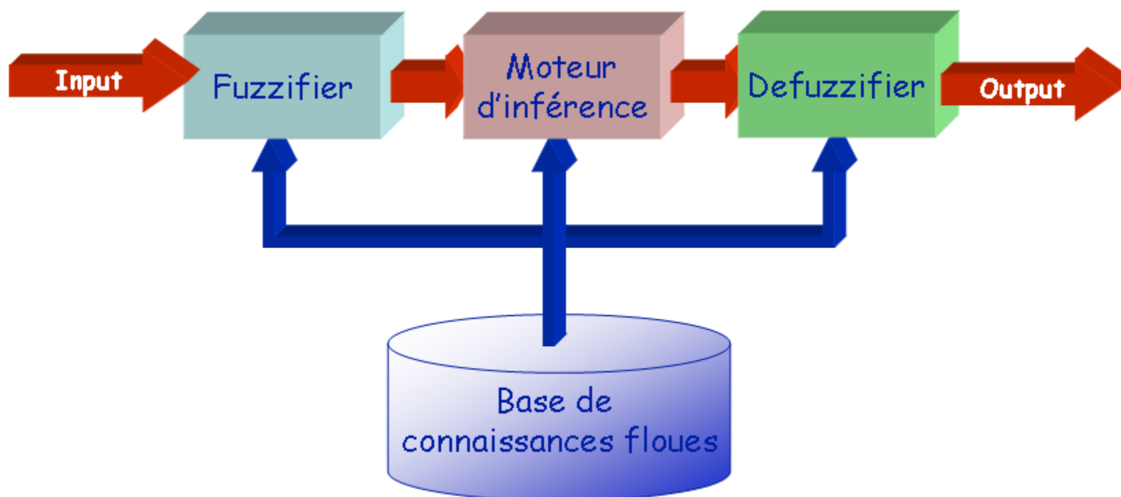
Figure 1.13: Aperçu synoptique d'un système Flou
