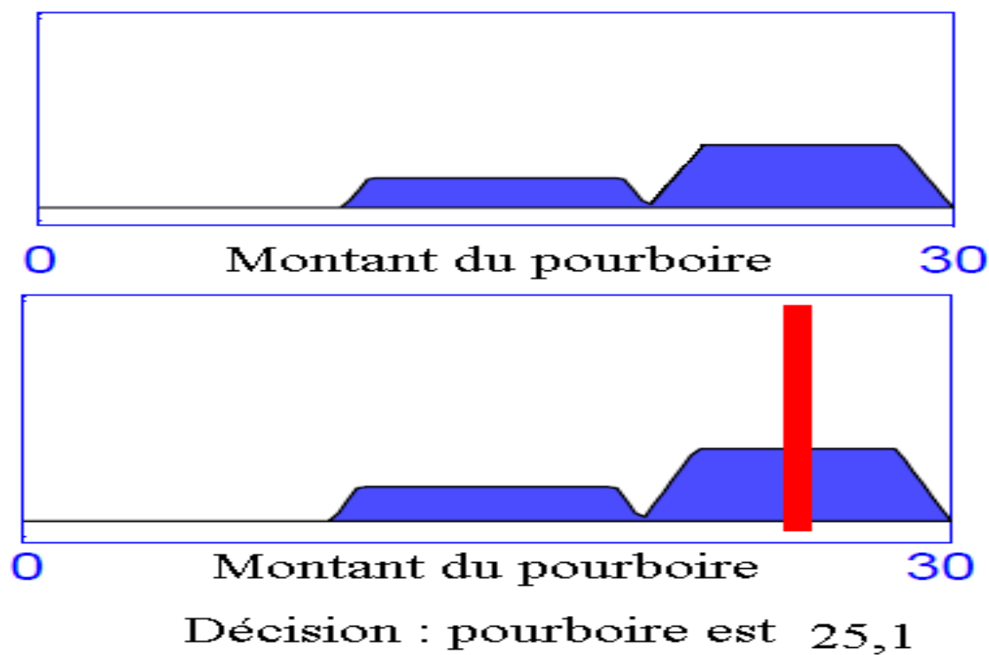
Figure 1.11: Defuzzification avec la méthode moyenne des maxima(MM)
