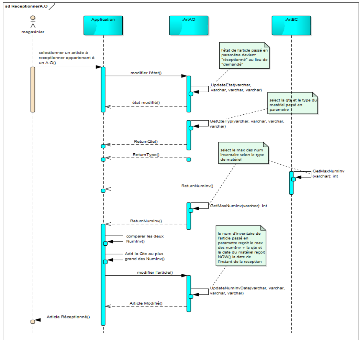
Figure 122: diagramme de séquence «ReceptionnerA.O»
