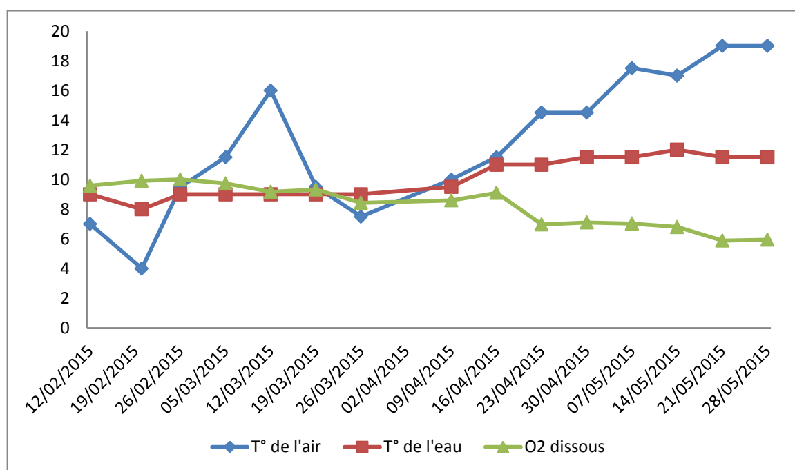
Figure 19: Evolution de l'effet de la température sur la solubilité de l'oxygène dissous
