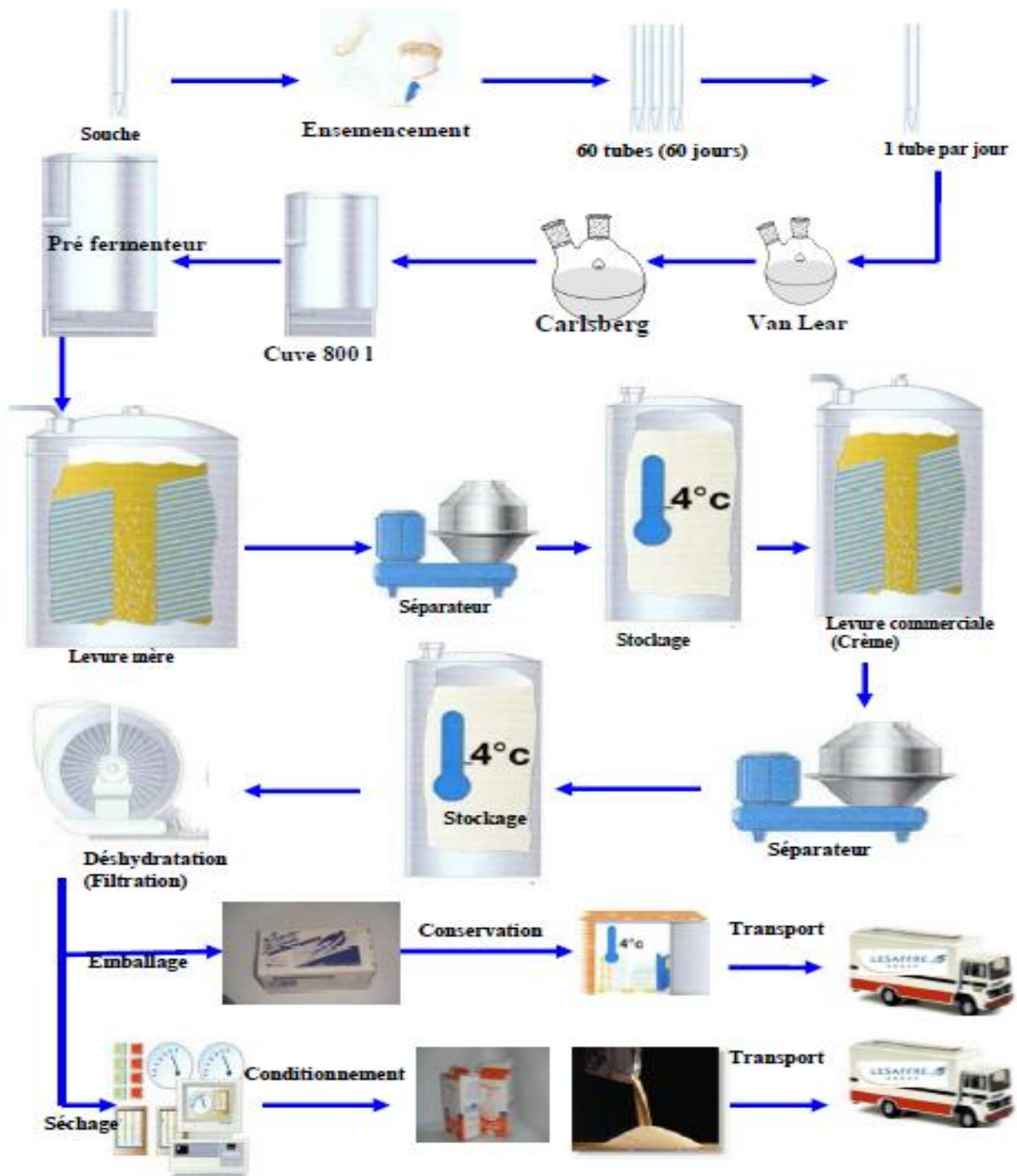
Figure 1 : Schéma général des différentes étapes de production de la levure
