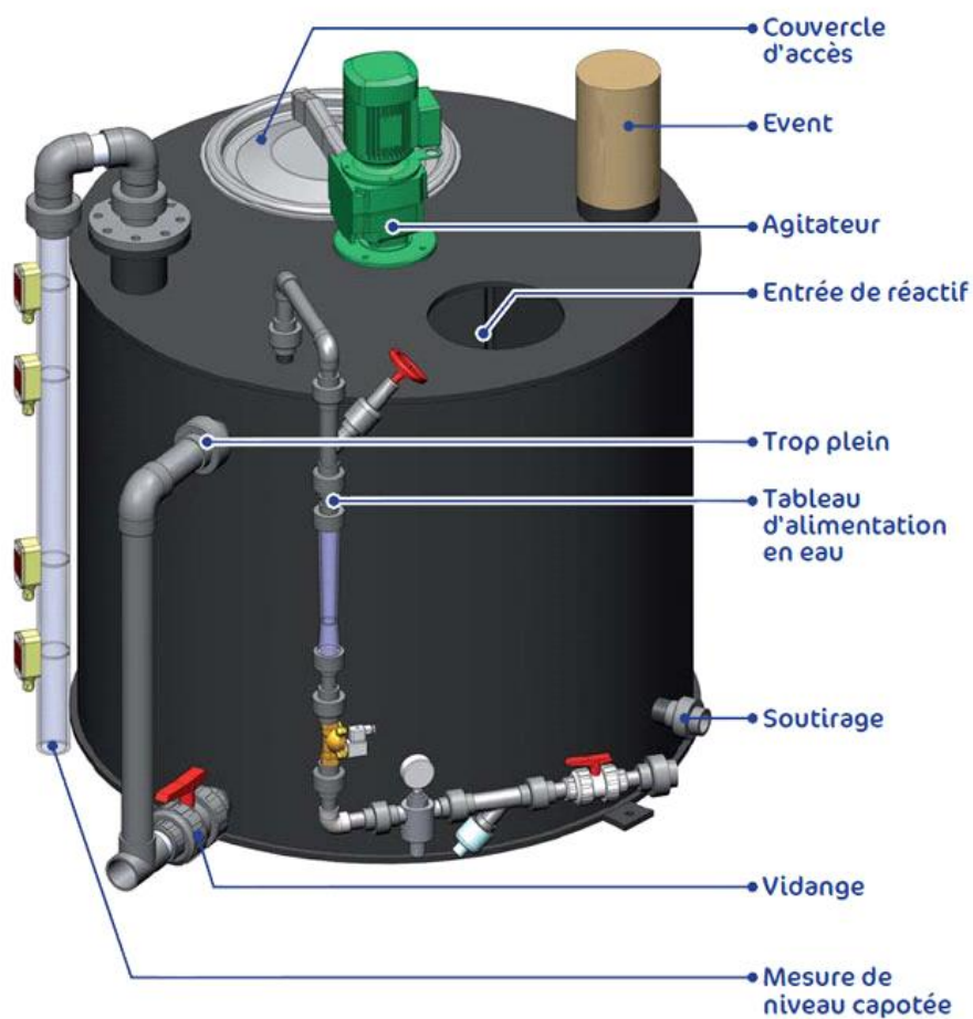
Figure 2 : Bac de préparation
