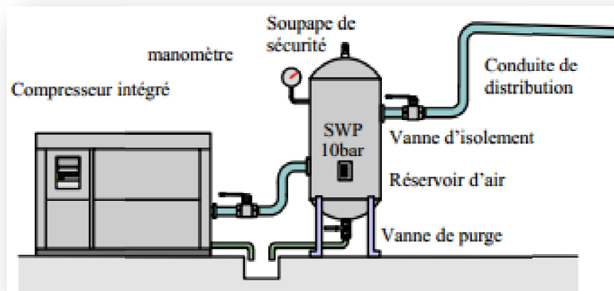
Figure 16: compresseur d'air
