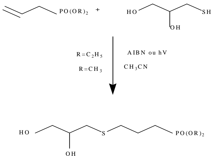
Schéma 24: Addition de thioglycérol sur l'allylphosphonate
