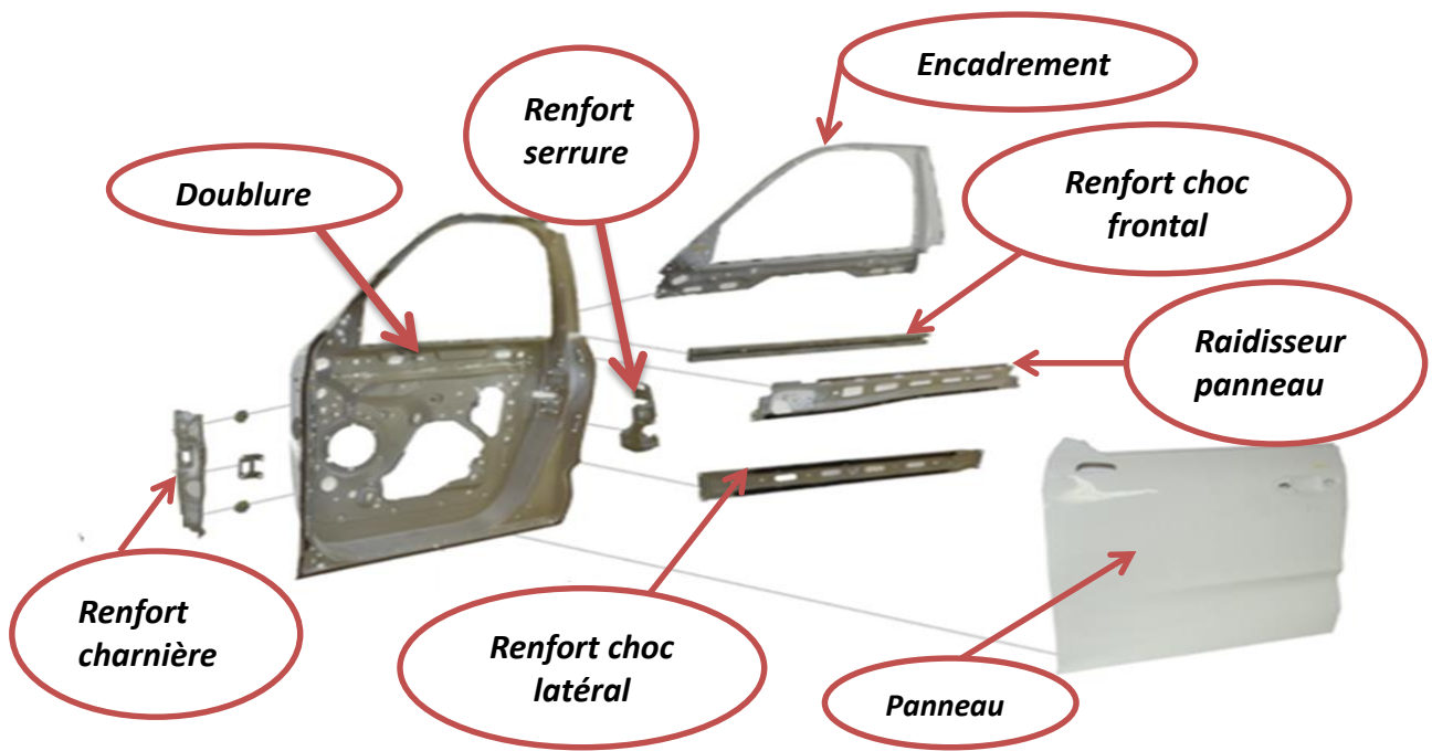
Figure 12 : Pièces tôlerie de porte latérale
