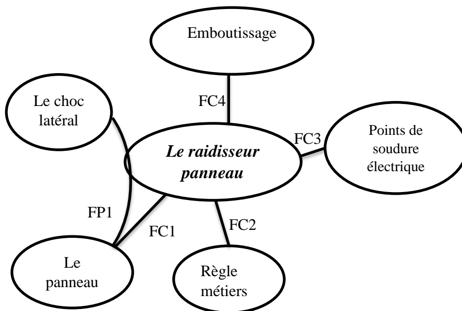
Figure 61 : la pieuvre de raidisseur panneau
