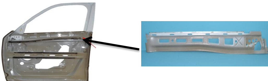
Figure 19 : La position de raidisseur panneau dans la porte
