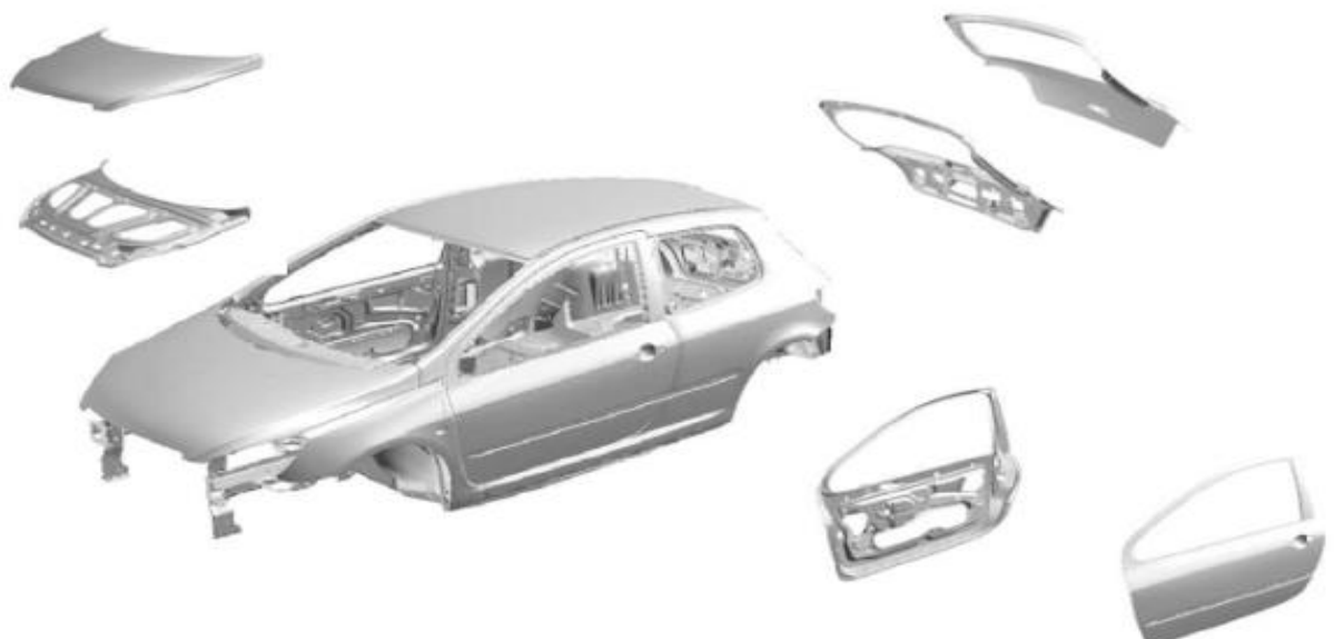
Figure 29 : Exemples d'ouvrants sur véhicules qui sont assemblés par sertissage
