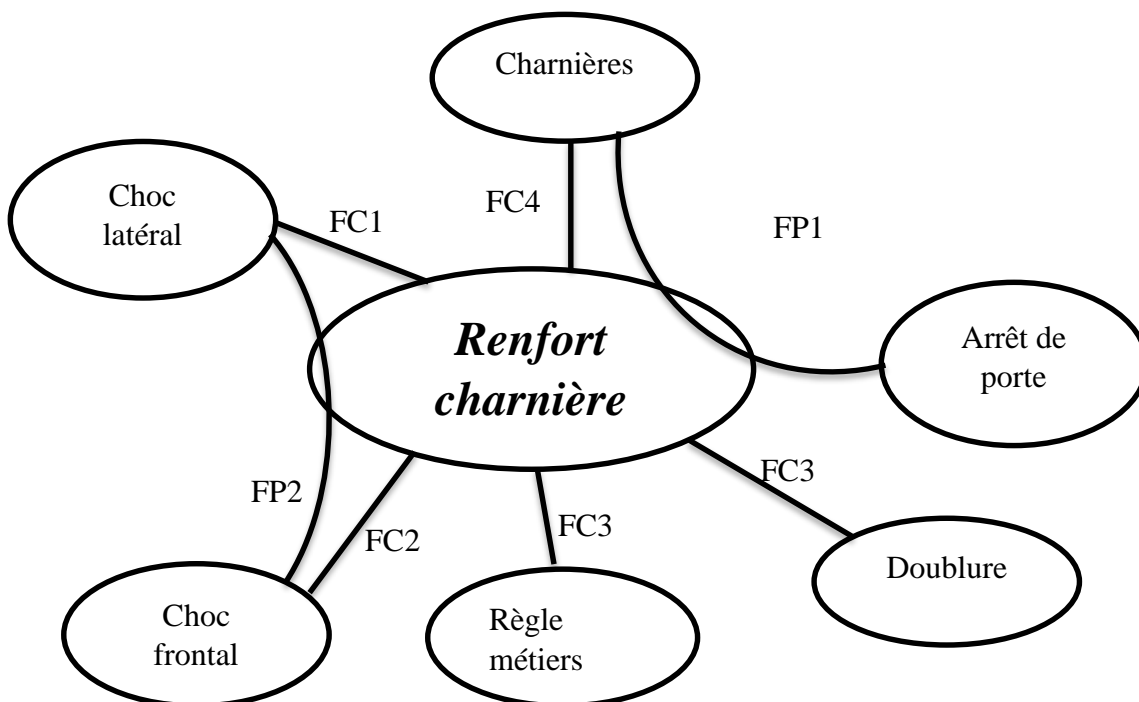
Figure 63 : la pieuvre de renfort charnière
