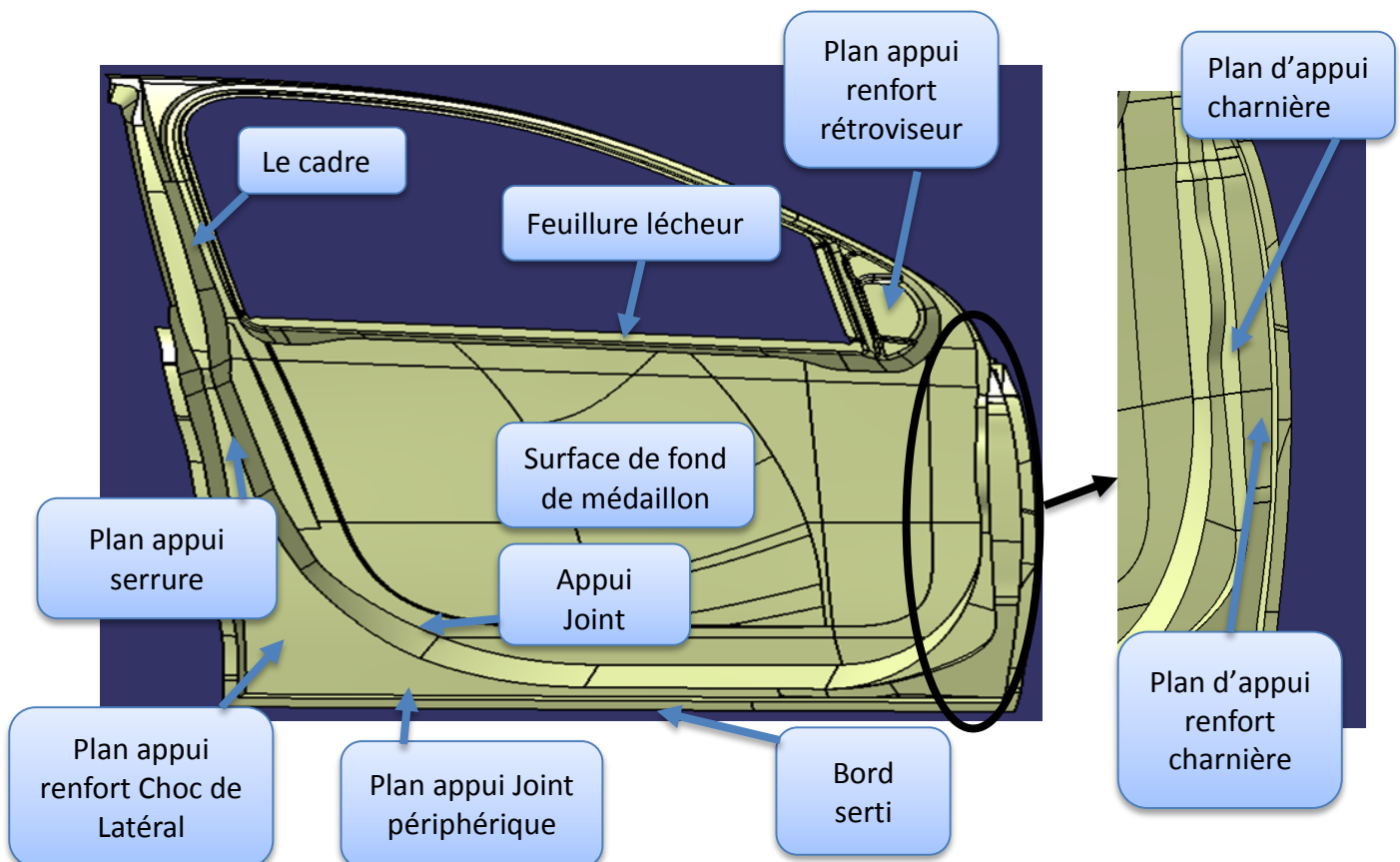
Figure 38 : Les différentes de zones de la doublure
