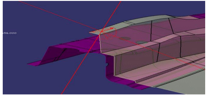
Figure 39 : section montre le jeu cinématique entre la doublure et le coté habitacle
