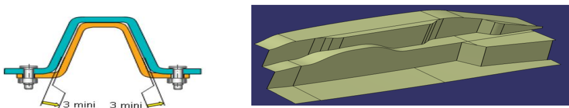
Figure 65 : Construction du volume du renfort charnière
