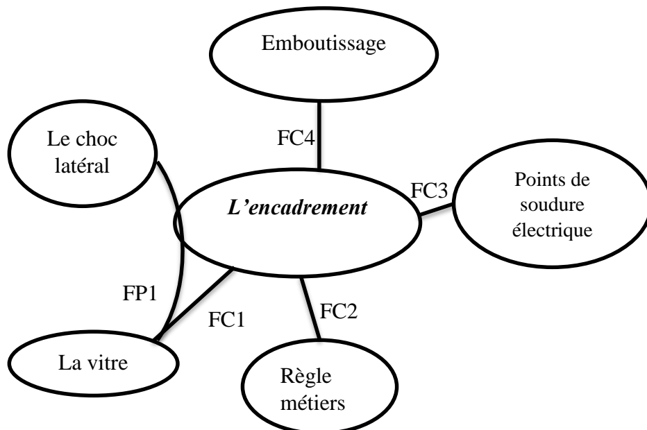
Figure 59 : la pieuvre de l'encadrement
