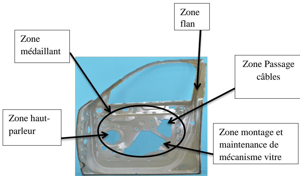
Figure 13 : La doublure de porte latérale
