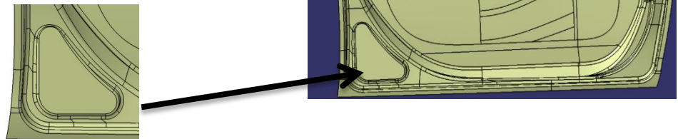
Figure 40 : Position de l'embouti dans la doublure
