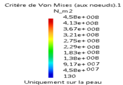
Figure 85 : Résultats des contraintes de Von Mises
