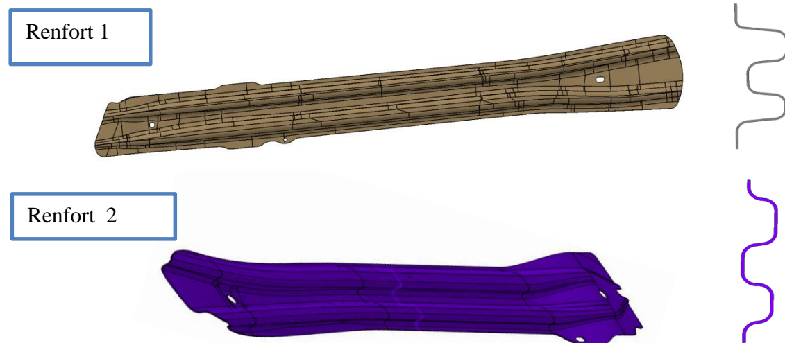
Figure : 25 les deux renforts de choc latéral étudiés
