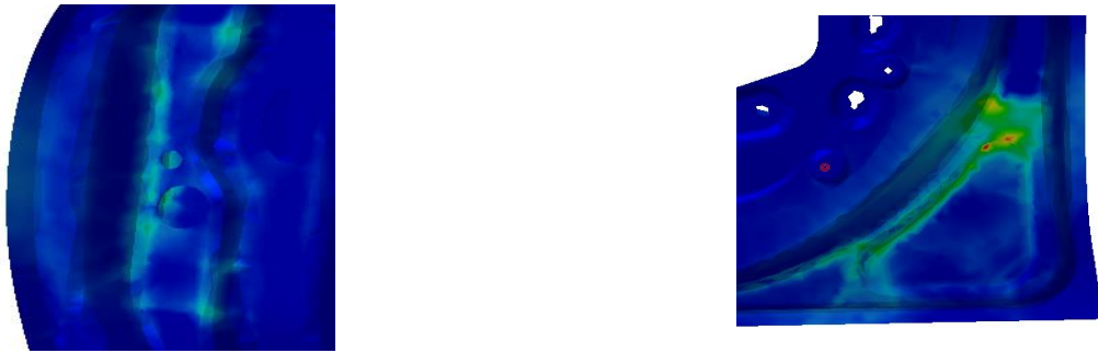
Figure 86 : Position des contraintes les plus sollicitées
