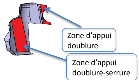
Figure 58 : Les zones d'appui de renfort serrure
