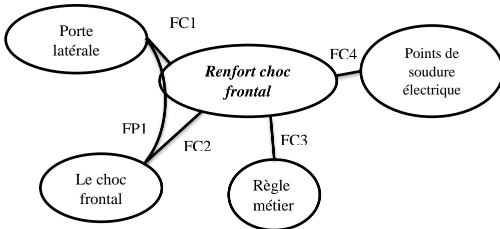
Figure 50 : la pieuvre de renfort choc frontal
