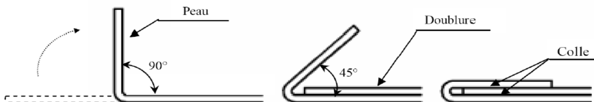
Figure 31 : Opérations de tombage, de pré sertissage et de sertissage des tôles métalliques
