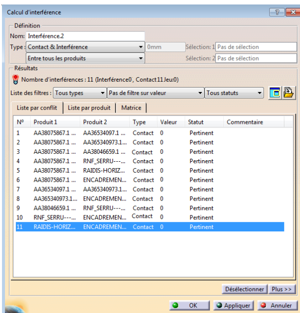
Figure 79 : Résultats de calculs d'interférence
