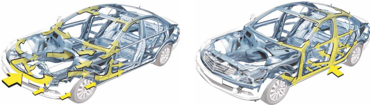
Figure 24 : Parcours de force en cas de choc latéral et frontal
