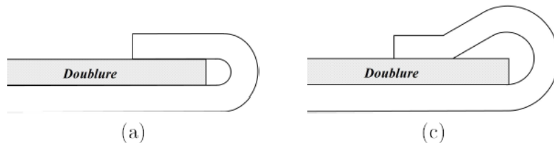
Figure 32 : Schématisation des différentes géométries de sertissages existantes :
