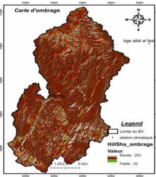
Fig16 : Carte d'Ombrage au niveau du bassin versant
