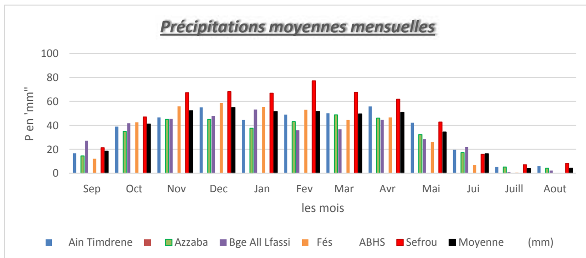
Fig 38: Précipitations moyennes mensuelles au niveau des 5 stations
