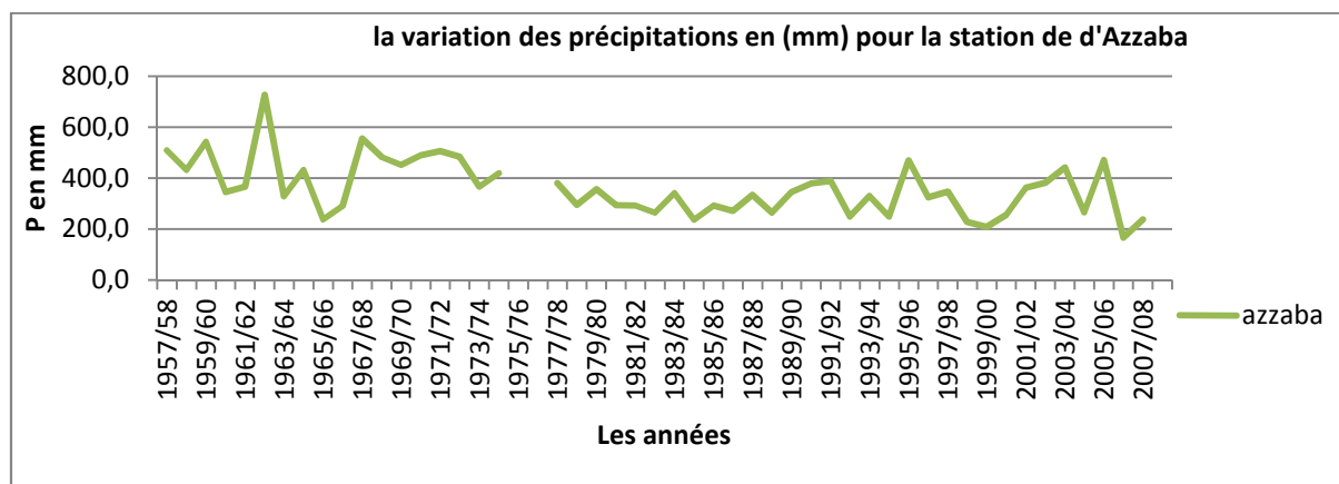
Fig 28: la variation des précipitations en (mm) pour la station d'Azaba
