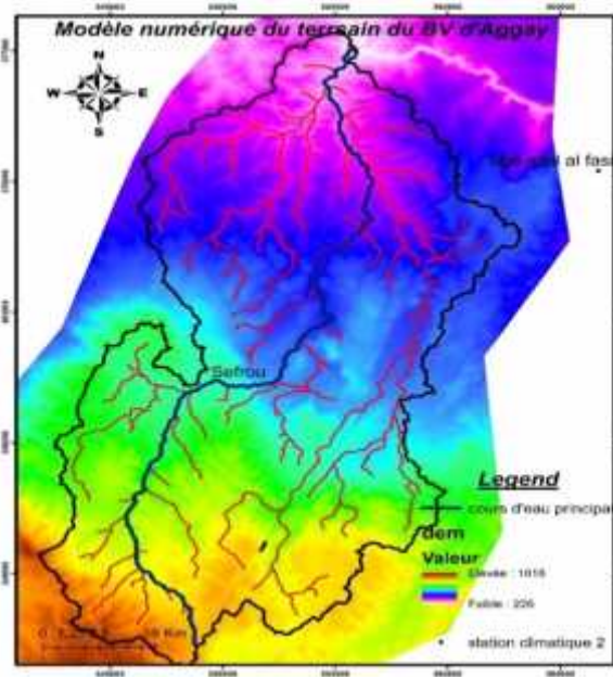
Fig6: Le MNT au niveau du bassin
