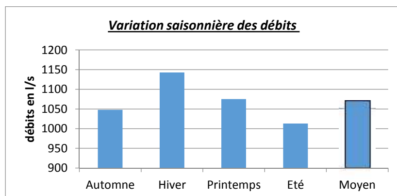
Fig 53 : Variation saisonnière des débits
