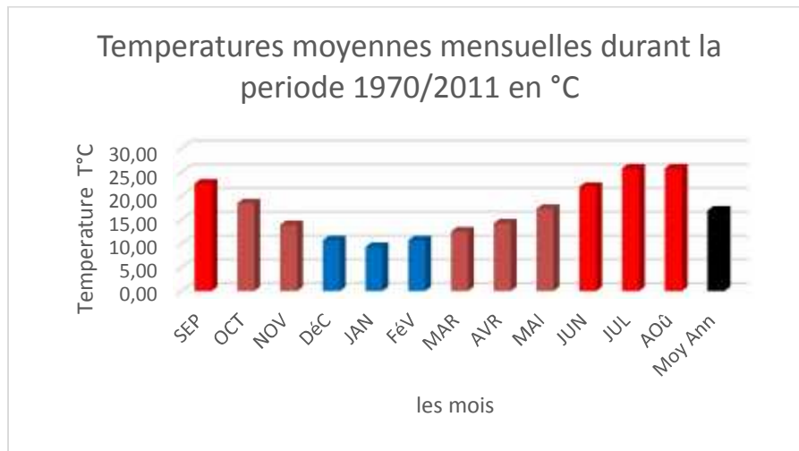
Fig 42: Températures moyennes mensuelles durant la période 1970/2011 en °C
