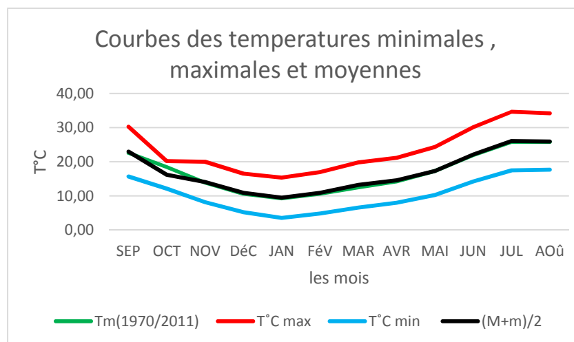
Fig 43: Courbes des températures minimales, maximales et moyennes
