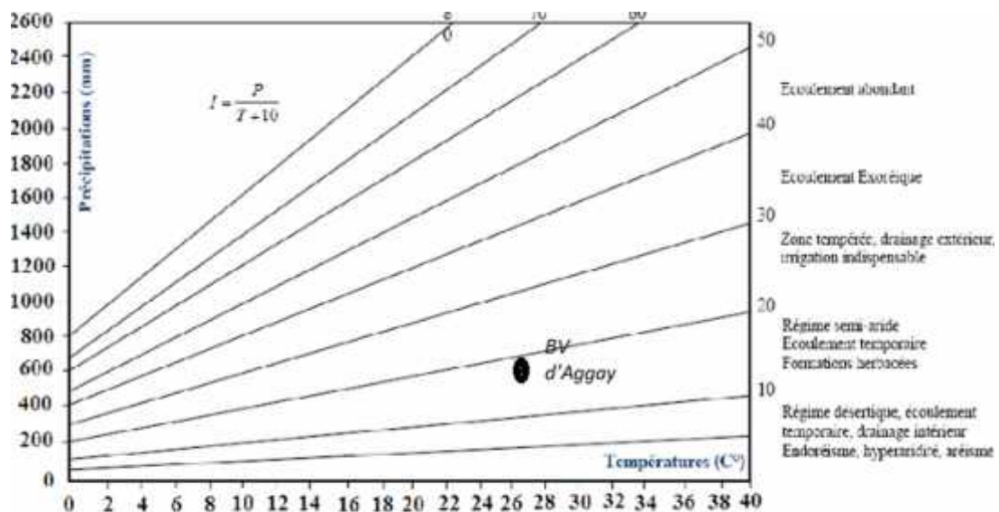
Abaque de L'indice d'aridité annuel De Martonne
