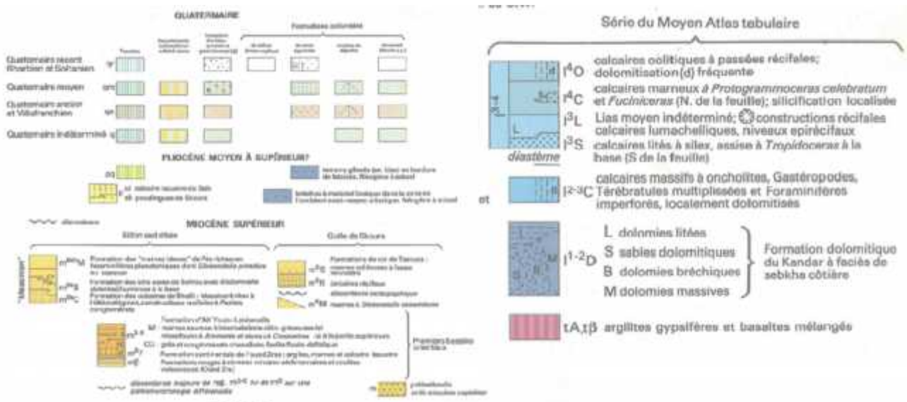
Fig 22 La litho-stratigraphie du bassin versant d'Aggaj
