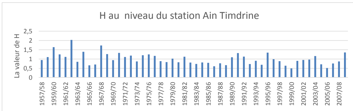
Fig 33 : La variation du H au niveau de la station d'Ain Timdrine
