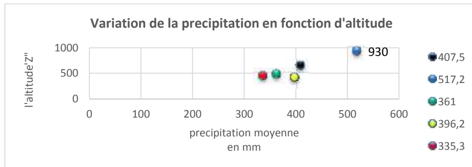
Fig39 : Variation de la pluviométrie en fonction d'altitude
