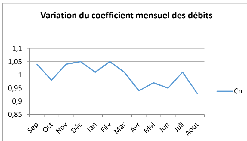
Fig 52 : Variation du coefficient mensuel des débits
