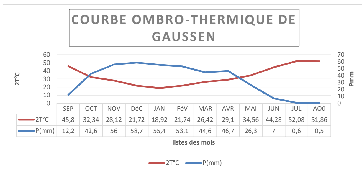
Fig 46: courbe ombrothermique de Gaussen
