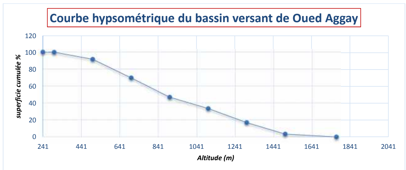
Fig8 : Courbe Hypsométrique du bassin versant d'oued Aggay
