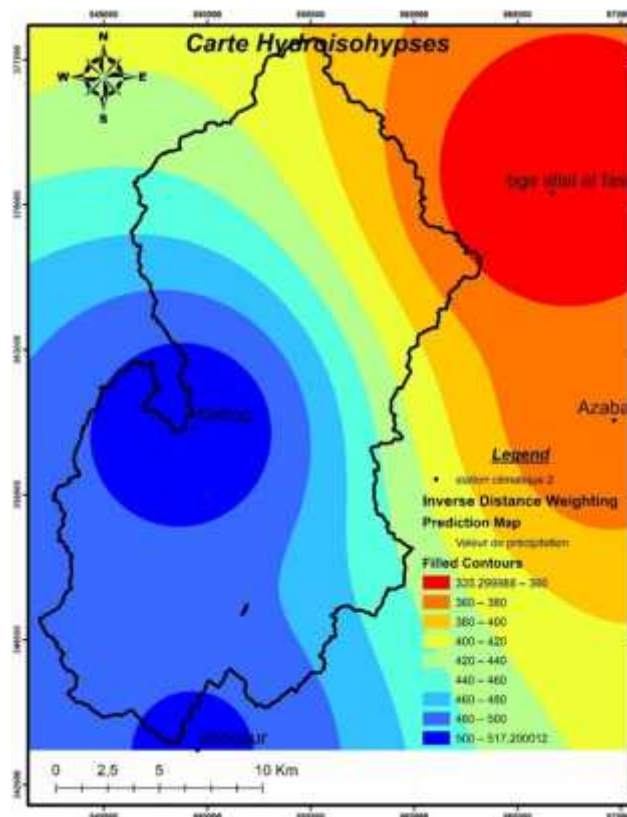
Fig 41: Carte Hydro isohypses par ArcGis
