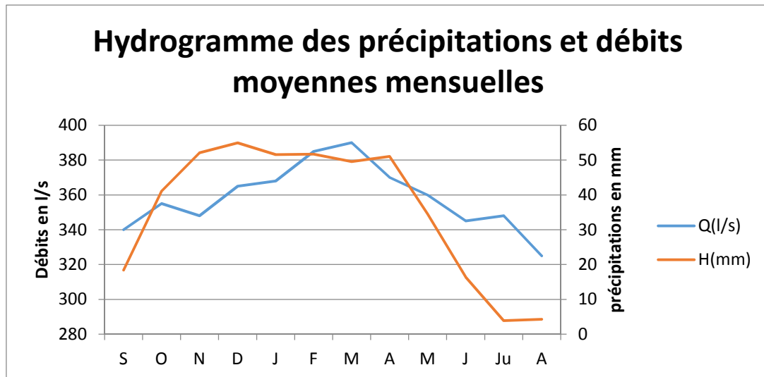
Fig 54 : Hydrogramme des précipitations et moyenne mensuelle et des débits moyens mensuels
