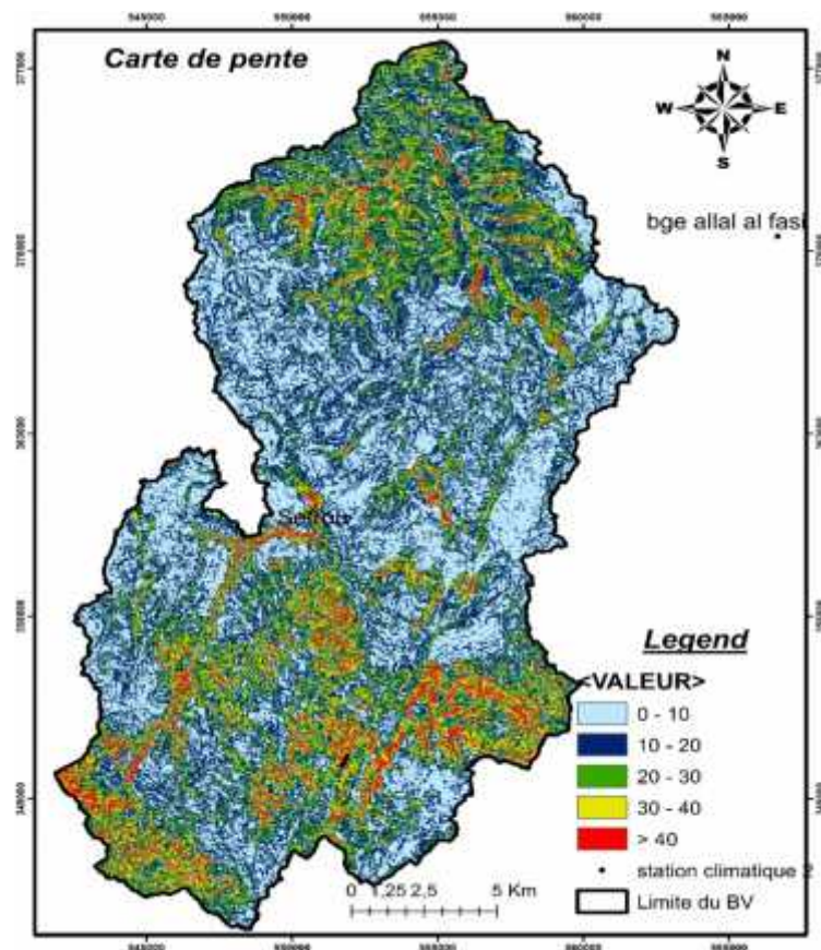
Figure 12 : la carte de pente au niveau de la zone d'étude d'après ArcGis
