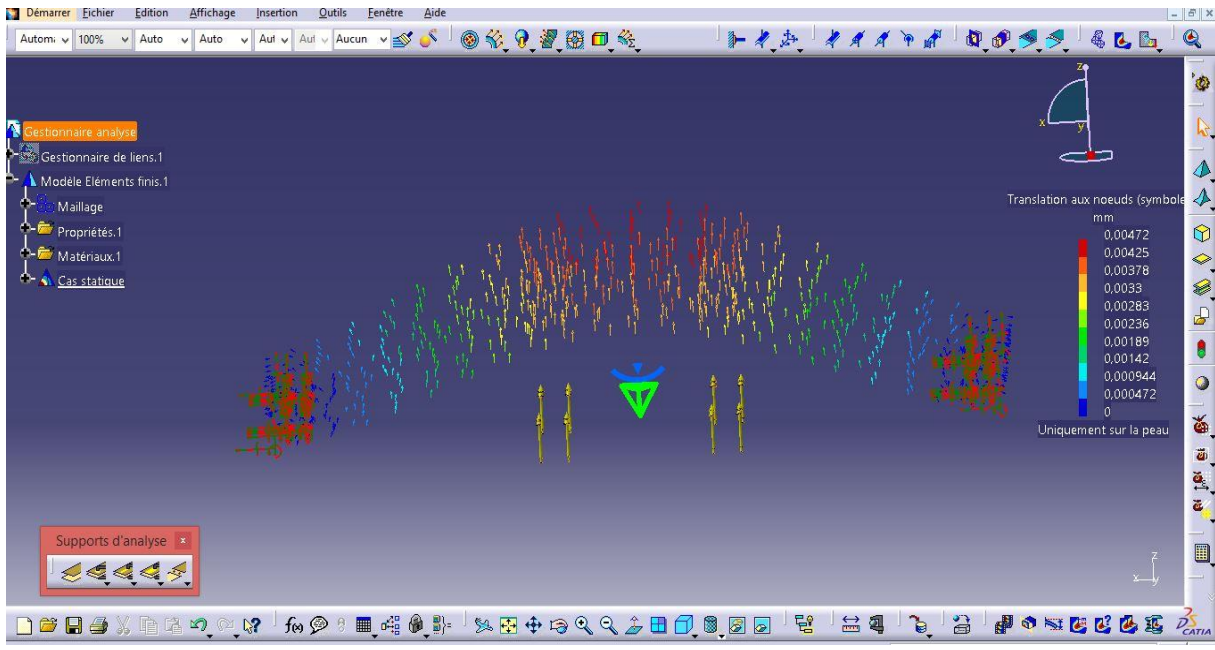
Figure 23:translation au nœud.
