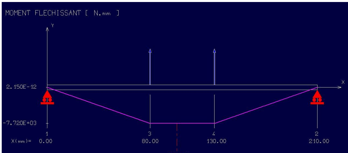
Figure 21: Diagramme des moments fléchissant.
