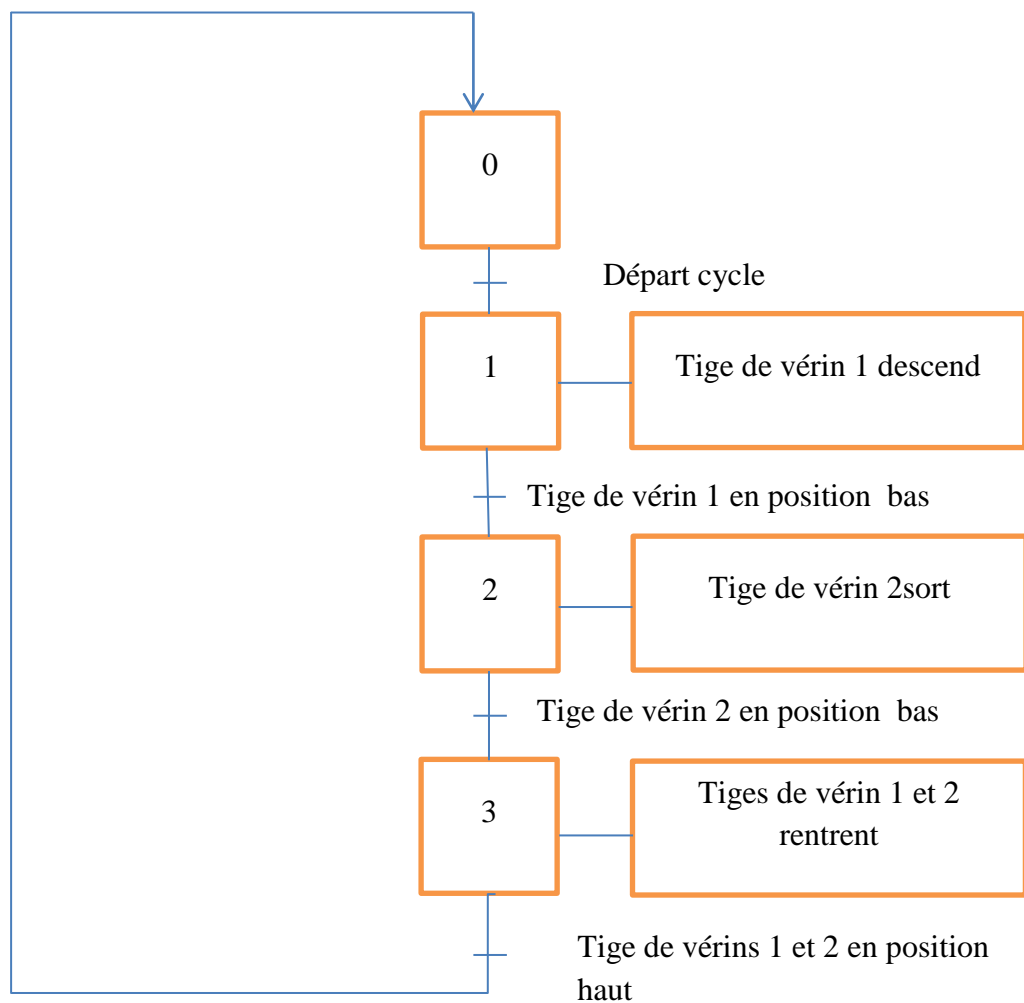
Figure 39: Grafcet (Niveau I).
