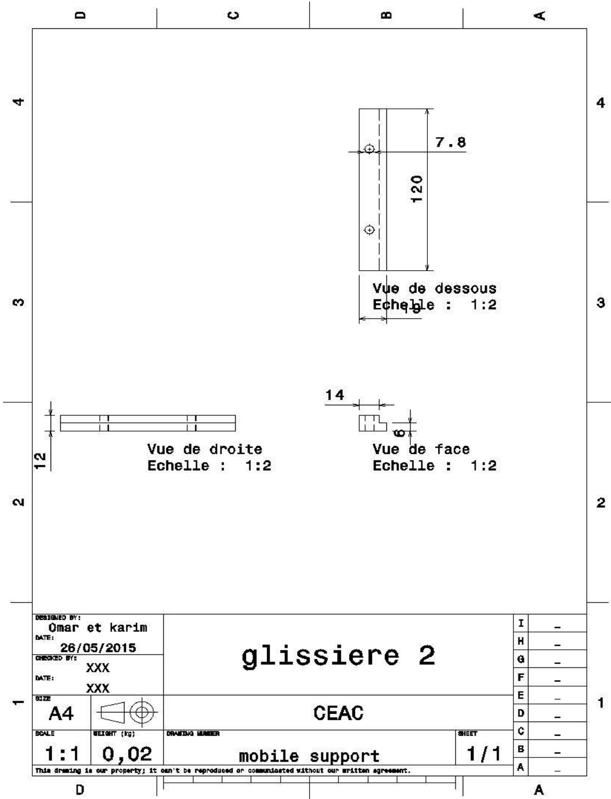
Figure 45: Drafting de glissière 2.
