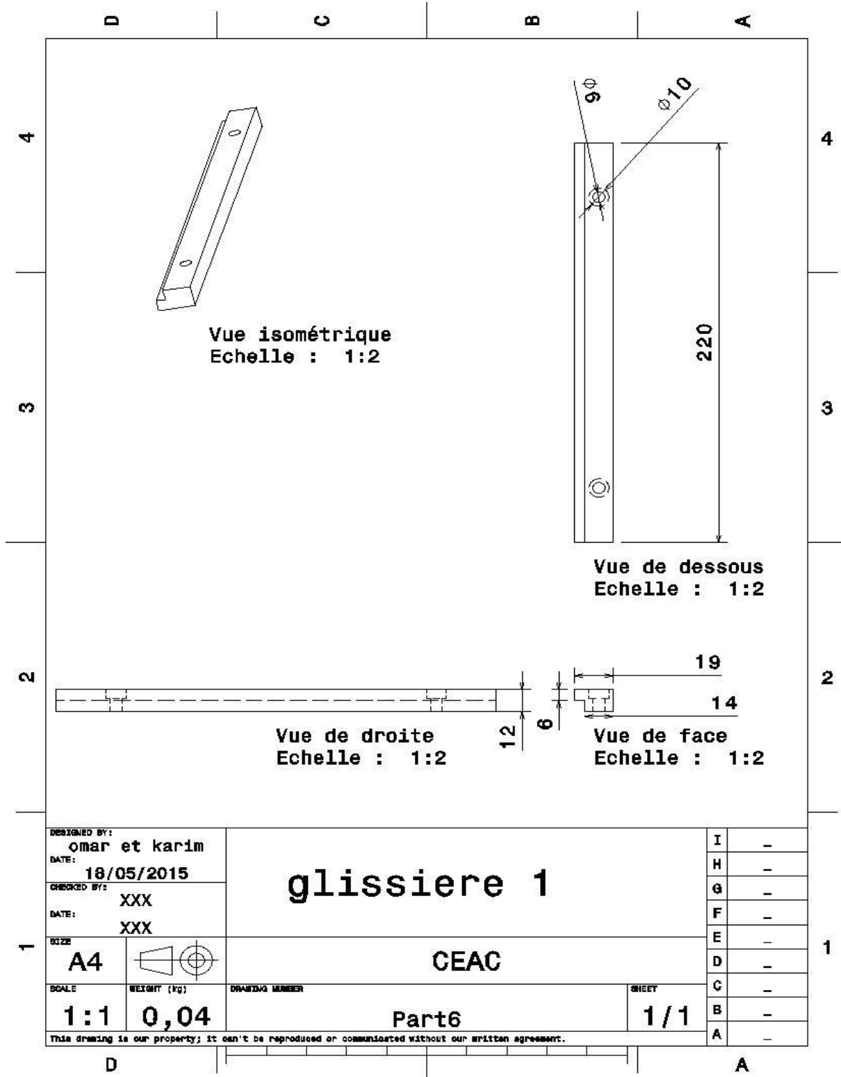
Figure 46: Drafting de glissière 1.
