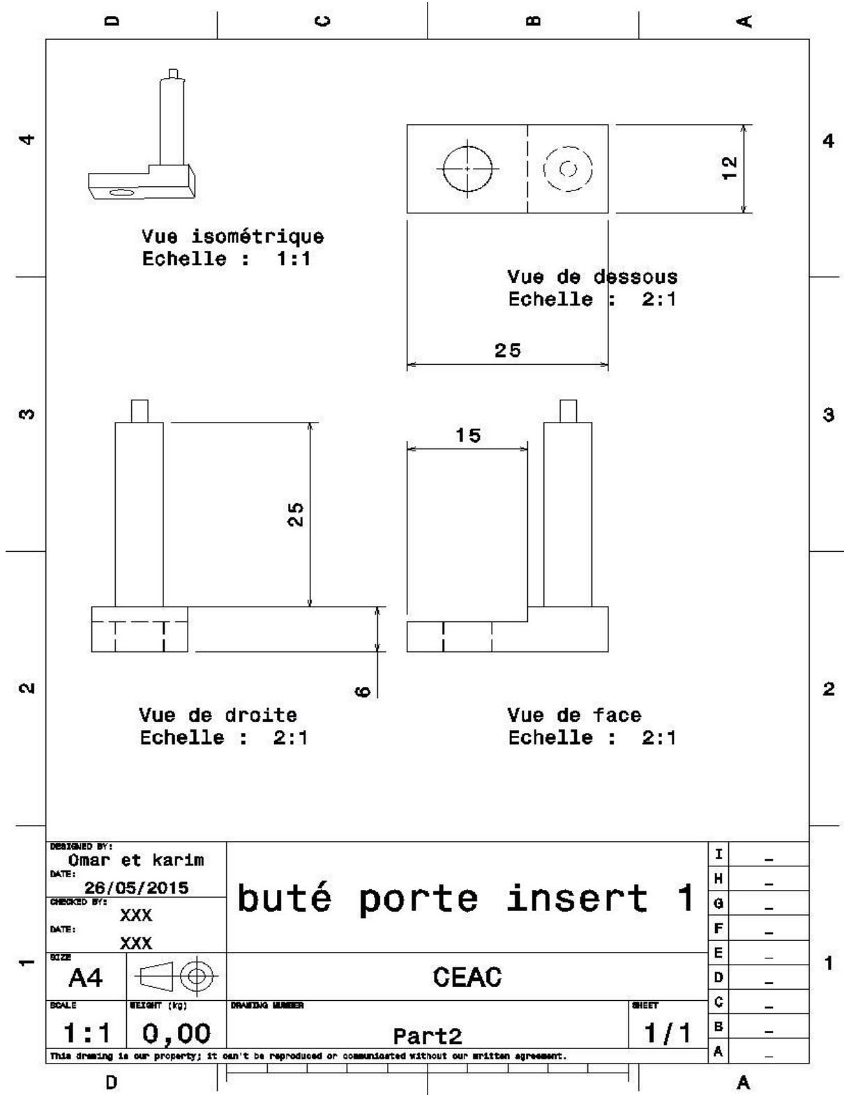
Figure 41: Drafting de buté 1.
