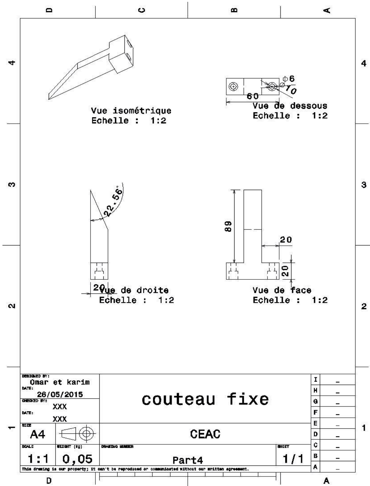
Figure 43: Drafting de couteau fixe.
