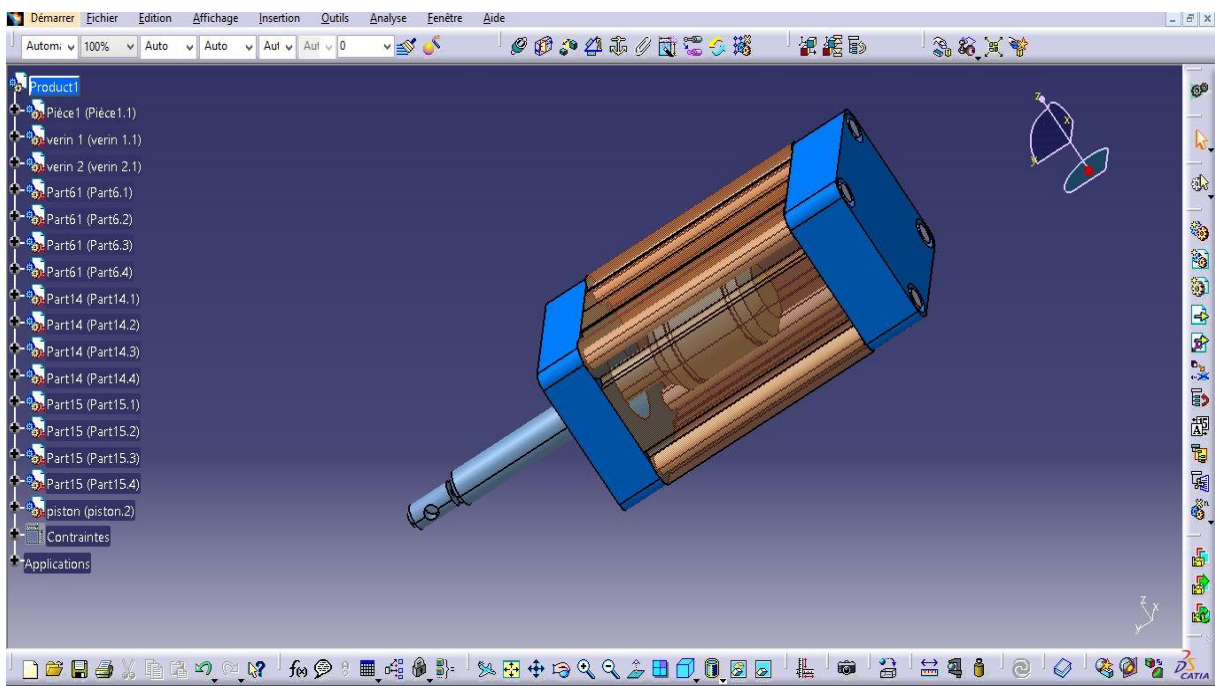
Figure 36: vérin pneumatique.
