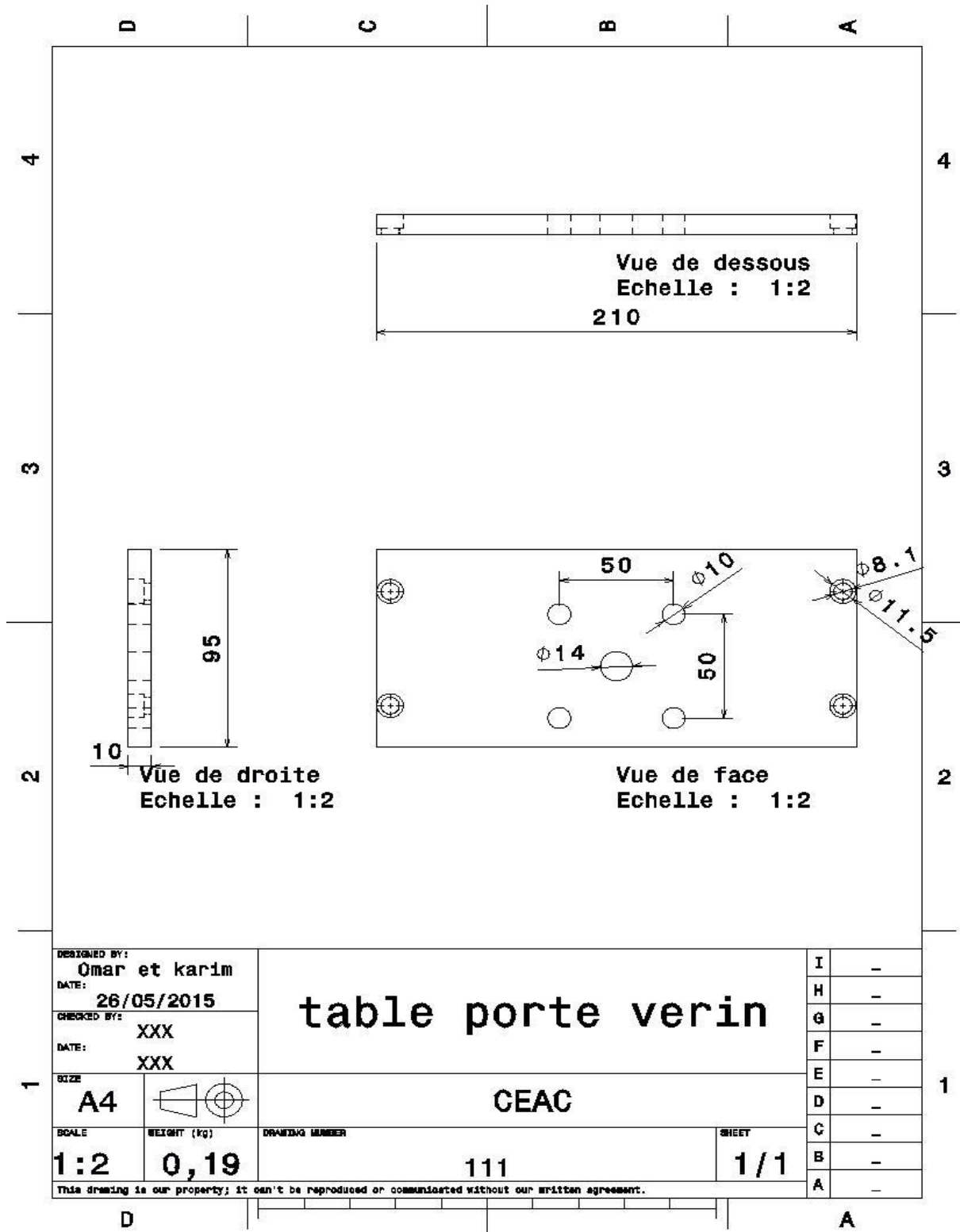
Figure 50: Drafting de table porte vérin.
