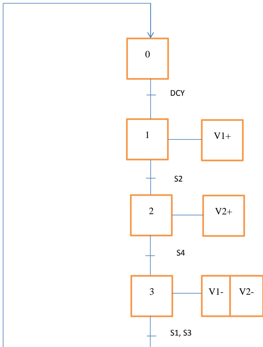
Figure 40: Grafcet (Niveau II).
