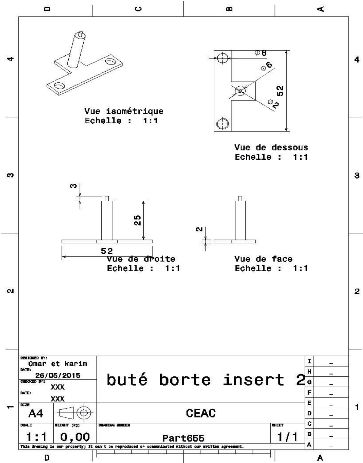
Figure 42: Drafting de buté 2.
