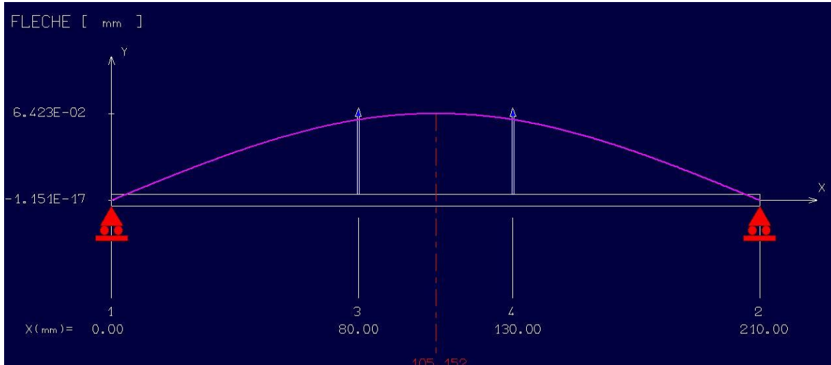
Figure 19: Diagramme de la flèche.
