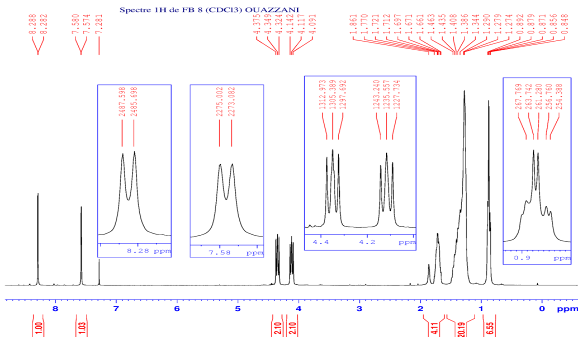
Figure13 : Spectre de RMN ^1\text{H} ( \text{CDCl}_3 - d_6 ; 300MHz) du composé 16.
