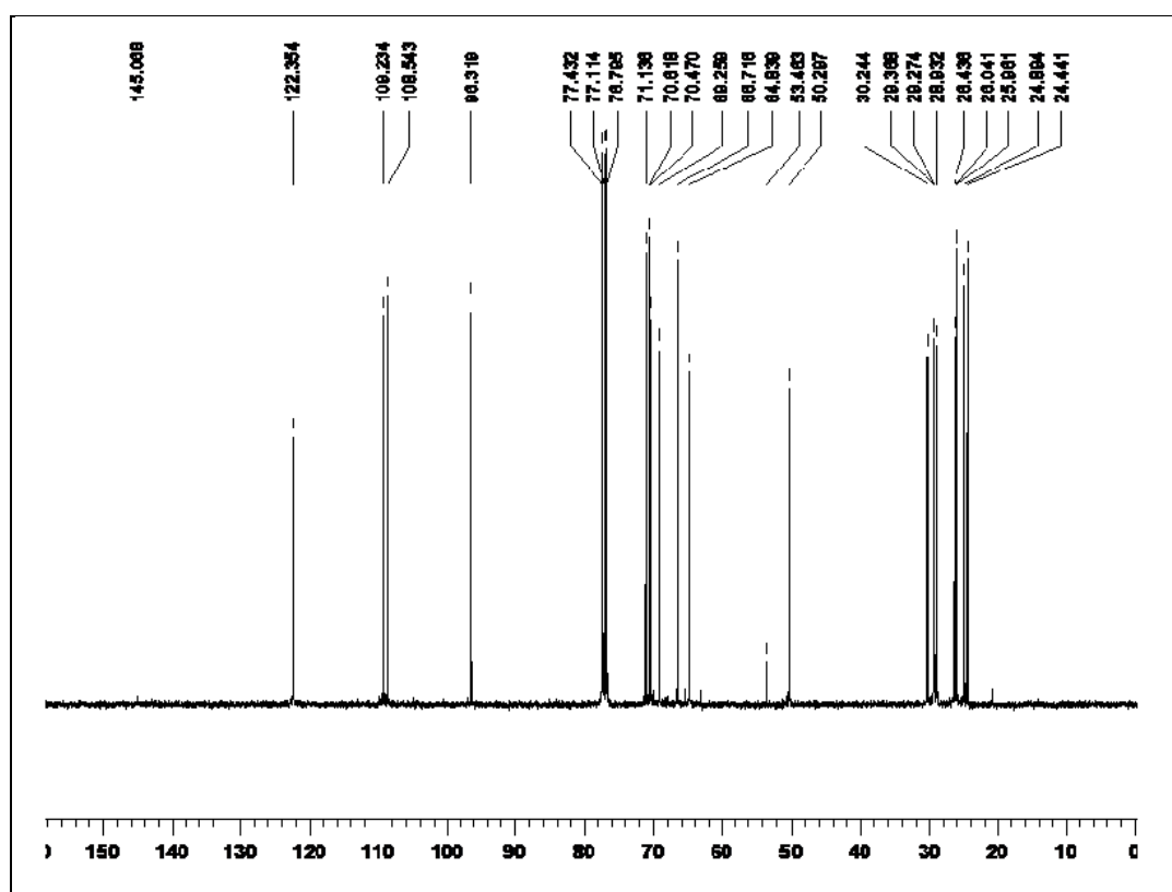
Figure 39 : Spectre de RMN 13C du 1'',12''-bis-[Galactosyl-1,2,3-triazol]-yl-dodécane 54.
