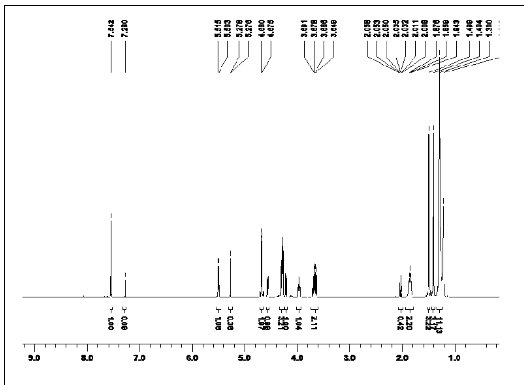
Figure 38 : Spectre de RMN 1H du 1'',12''-bis-[Galactosyl-1,2,3-triazol]-yl-dodécane 54.
