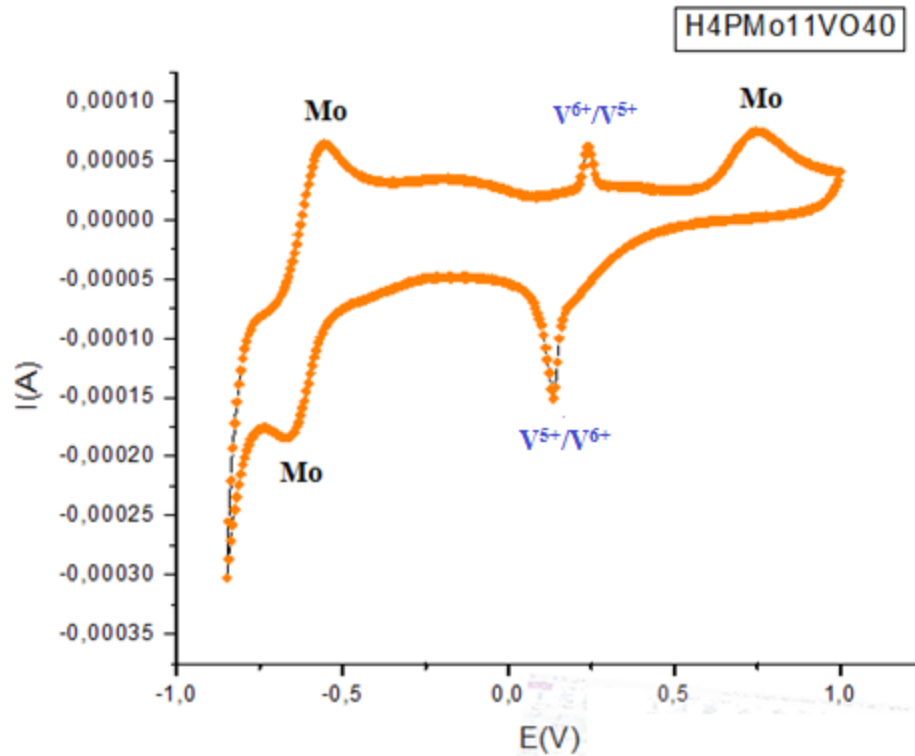
Figure 13 : Cyclovoltamogramme d'un échantillon de 1 mM de H_4PMo_{11}VO_{40} , dissout dans 0,5 M de Na_2SO_4 avec V_{bal}=10mV/s
