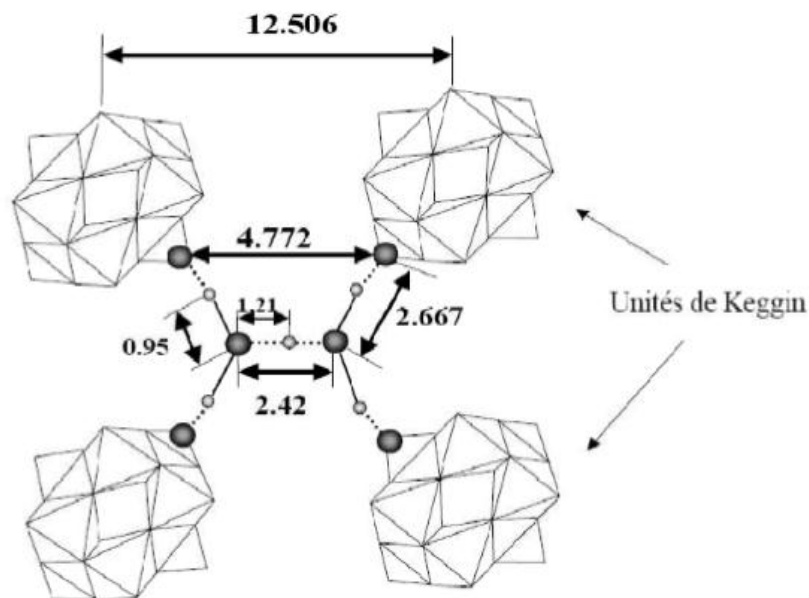
Figure 4: Hétéropolyacides avec des ponts dihydroxonium H_5O_2^+
