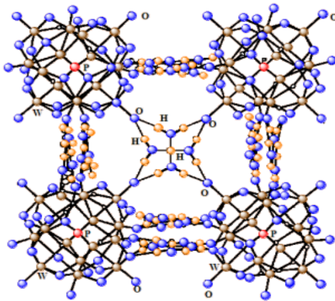
Figure 5 : hétéropolyacides avec des ponts tétrahydroxonium H_3O^{4+}
