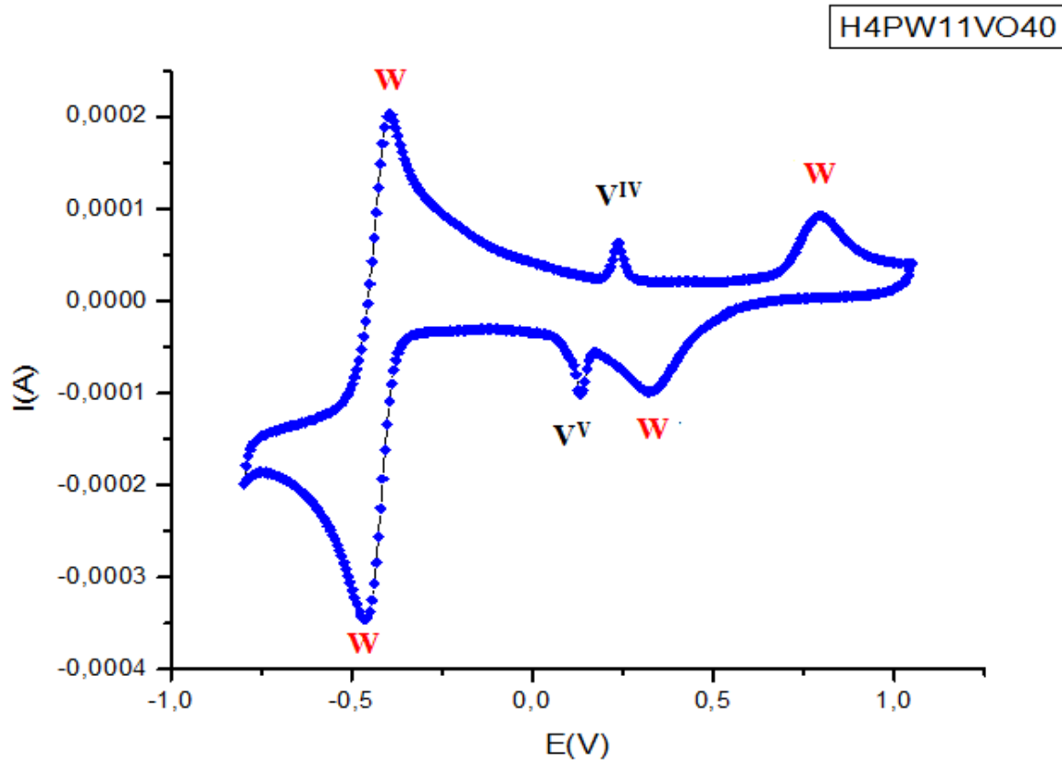
Figure 15 : Cyclovoltamogramme d'un échantillon de 1 mM de H_4PW_{11}VO_{40} dissout dans 0,5 M de Na_2SO_4 avec V_{bal}=10mV/s
