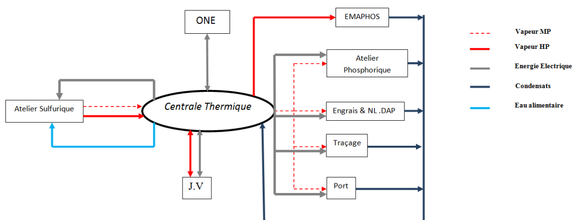
Figure 3: Cartographie présentant les entrées et les sorties des différentes utilités
