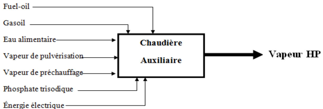
Figure 17: Schéma de la chaudière
