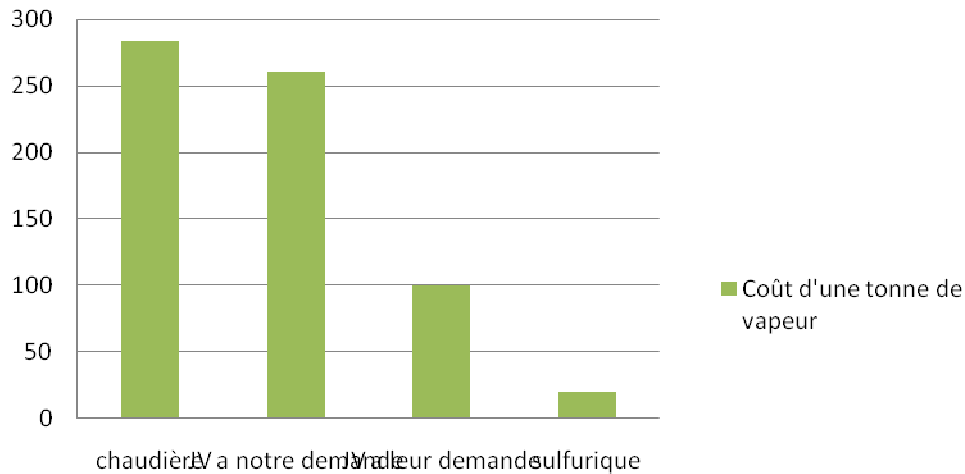
Figure 19: Comparaison entre le coût d'une tonne de vapeur HP produite par les différents fournisseurs
