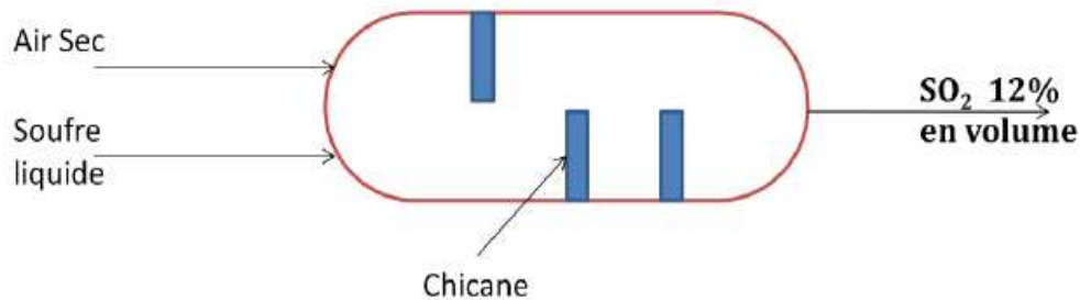
Figure 12: schéma simplifié du four de combustion
