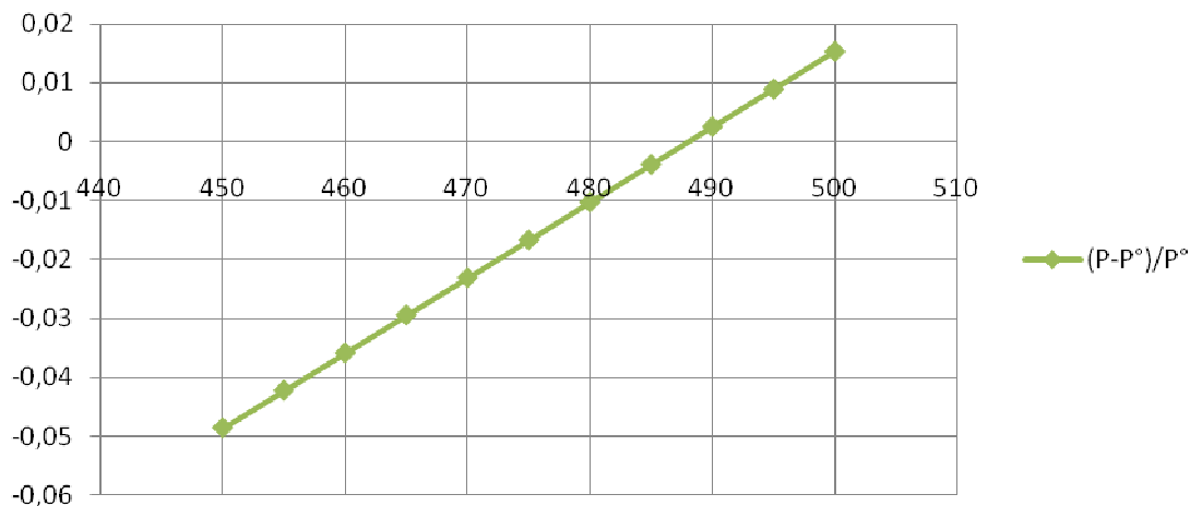
Figure 15: variation de la puissance relative en fonction de la température d'admission
