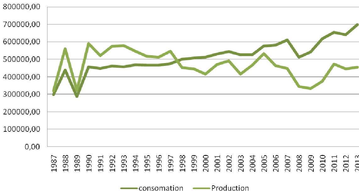
Figure 7: la production et la consommation d'énergie électrique
