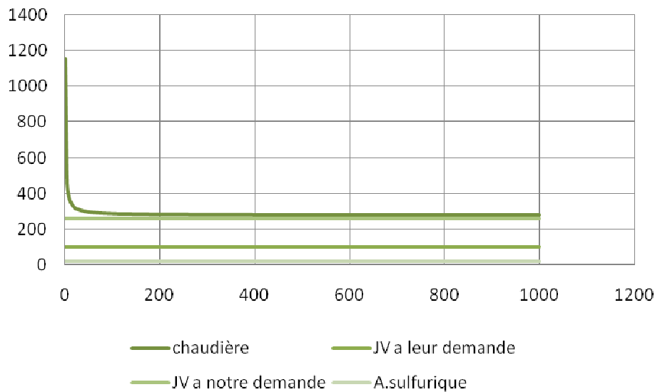
Figure 18: Variation du coût d'une tonne de vapeur
