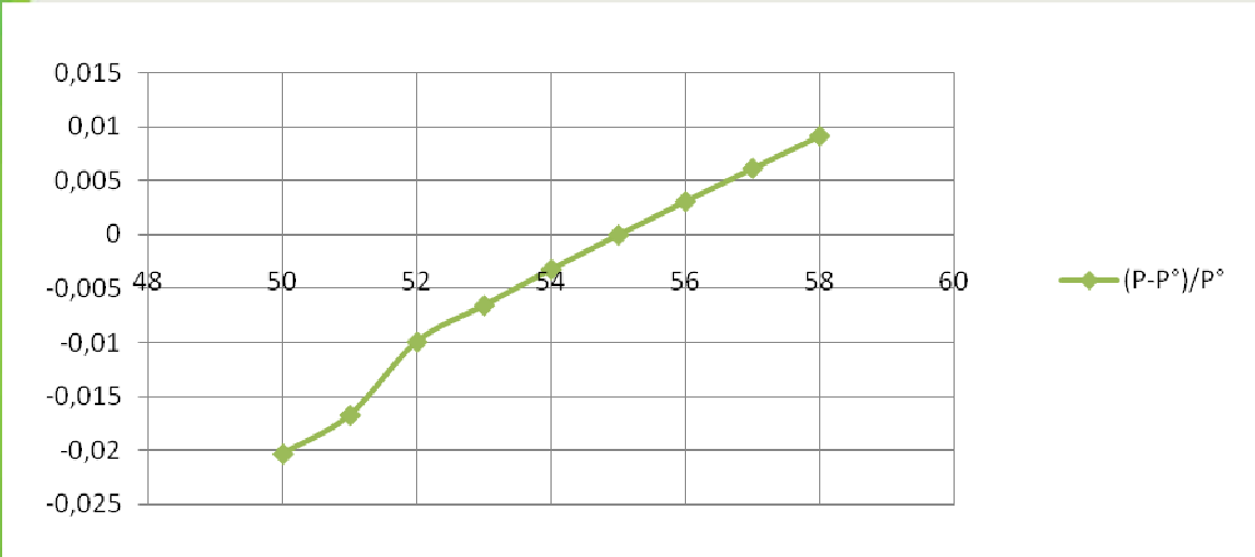
Figure 16: variation de la puissance relative en fonction de la pression a l'admission
