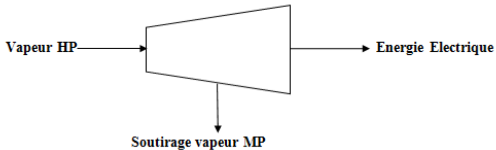
Figure 20: Schéma d'un GTA
