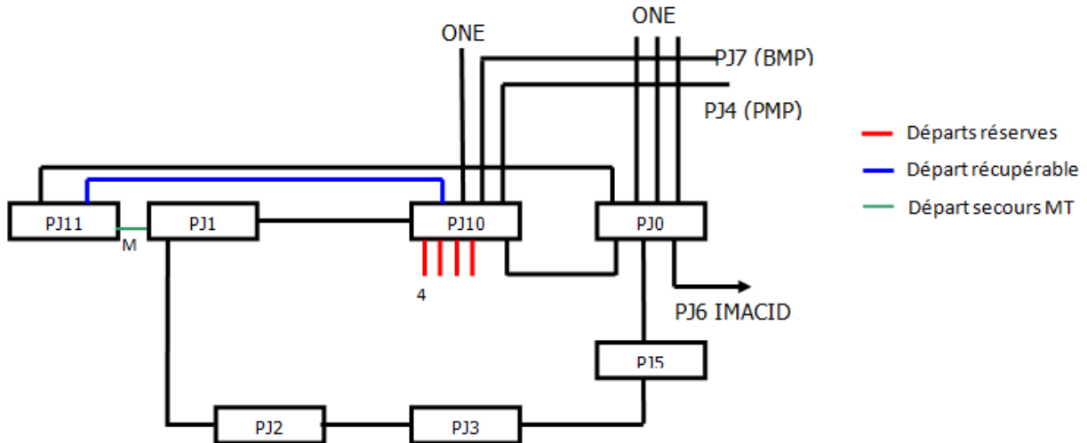
Figure 5: Boucle actuelle de l'E.E de JorfLasfar
