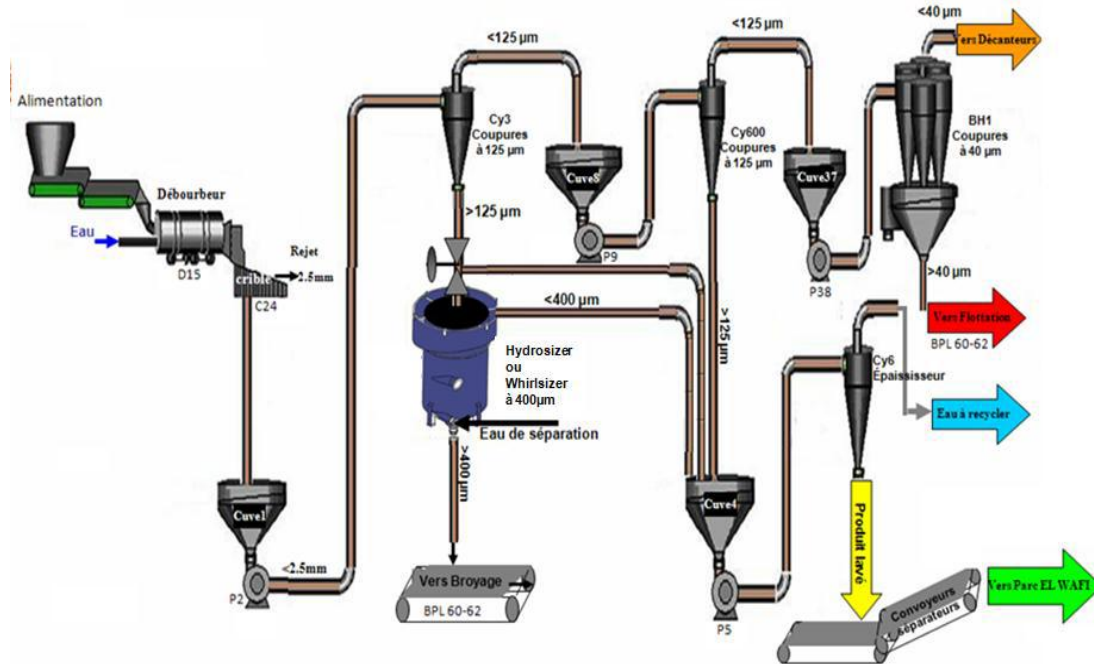
Figure 1 : logigramme d'une chaîne de lavage.
