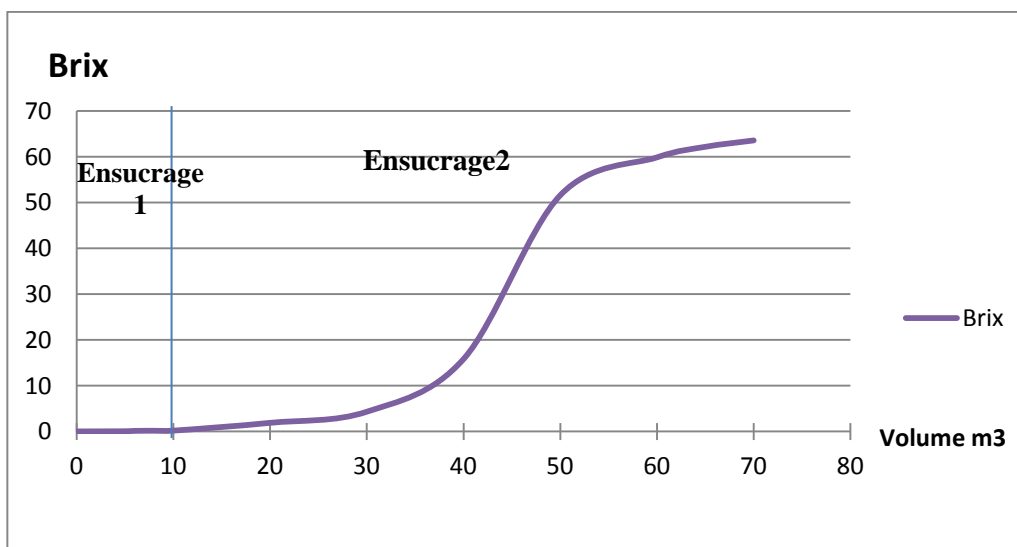
Figure 11: Evolution du Brix au cours de l'ensucrage.
