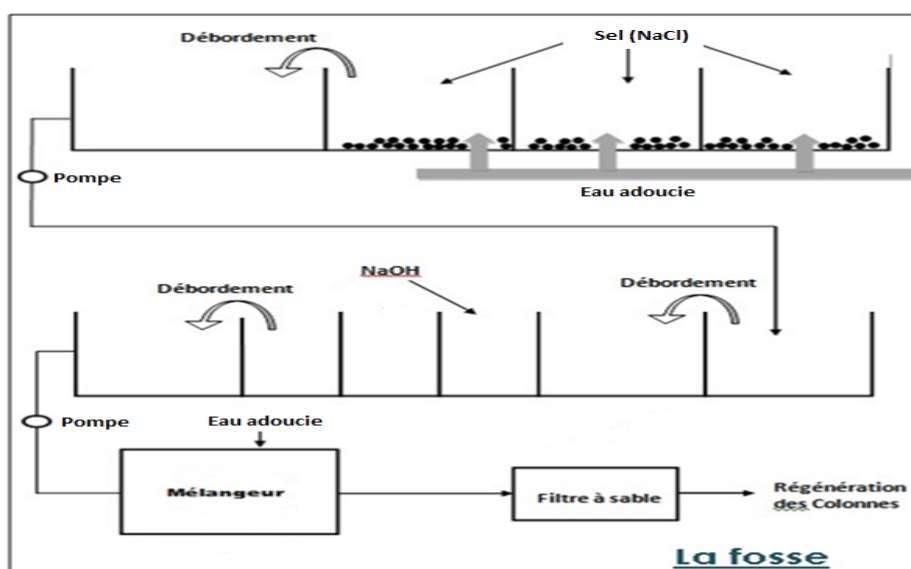
Figure 8: Schéma de la fosse à saumure.
