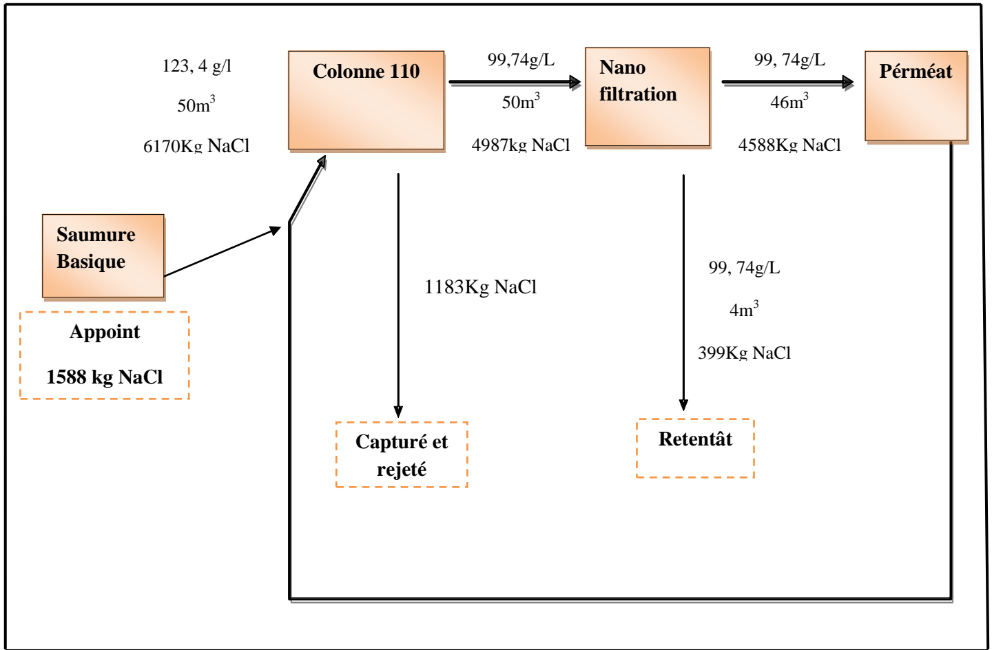
Figure 19 : Schéma du bilan de matière de NaCl
