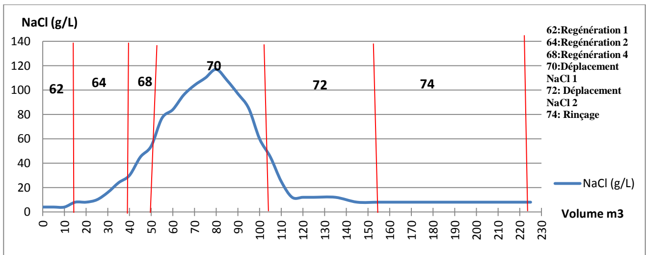
Figure 17 : Evolution de NaCl au cours de la régénération de la colonne après modification.
