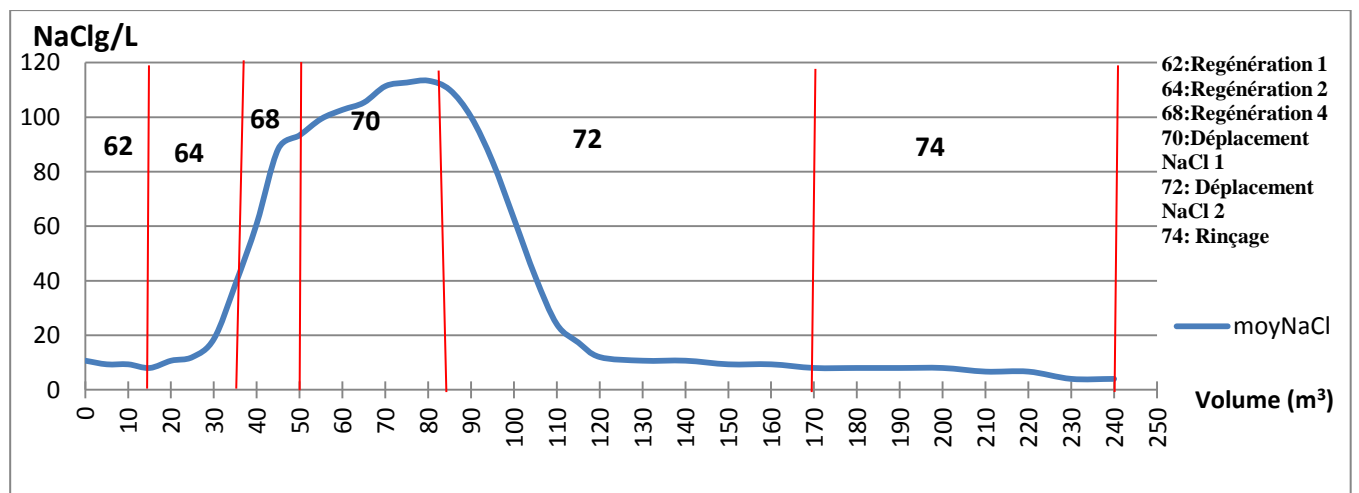
Figure 14 : Evolution de NaCl au cours de la régénération de la colonne
