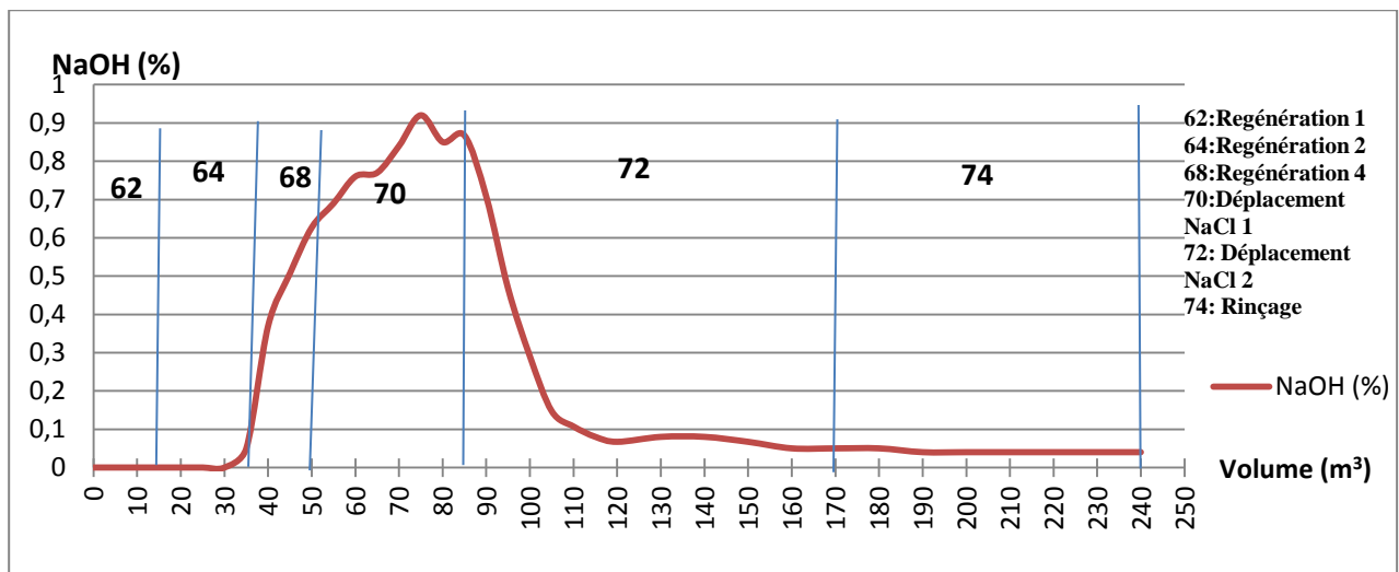
Figure 16 : Evolution de NaOH au cours de la régénération de la colonne
