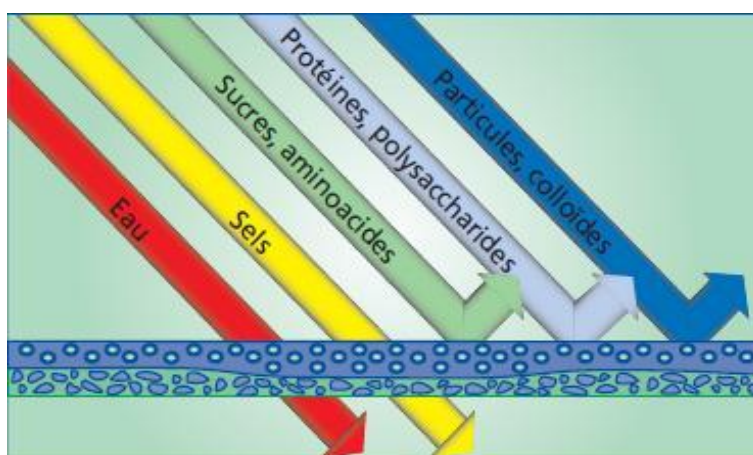
Figure 10: Principe de fonctionnement de la nanofiltration.
