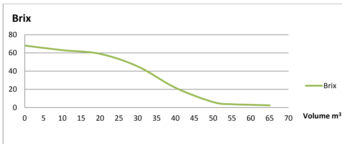
Figure 12: Evolution du Brix pendant le Dessucrage.
