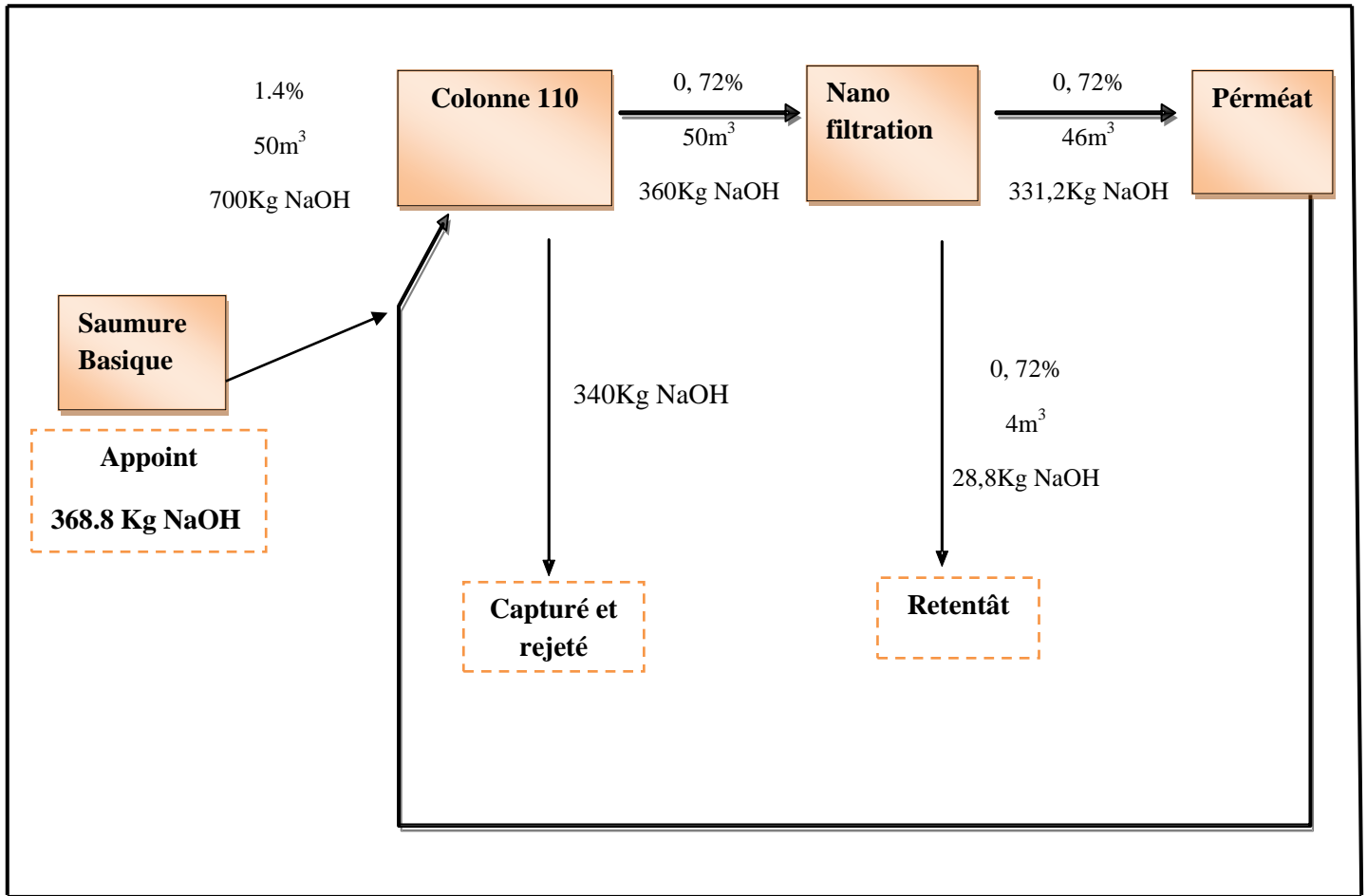
Figure 20 : Schéma du bilan de matière de NaCl
