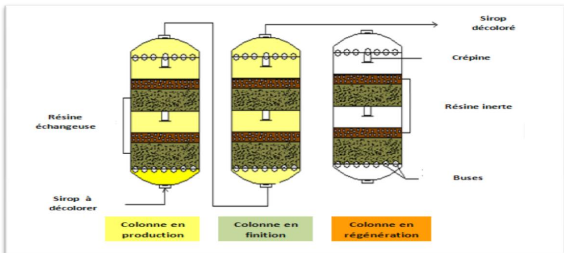
Figure 7 : Schéma de la chaîne de décoloration (colonnes 35.)
