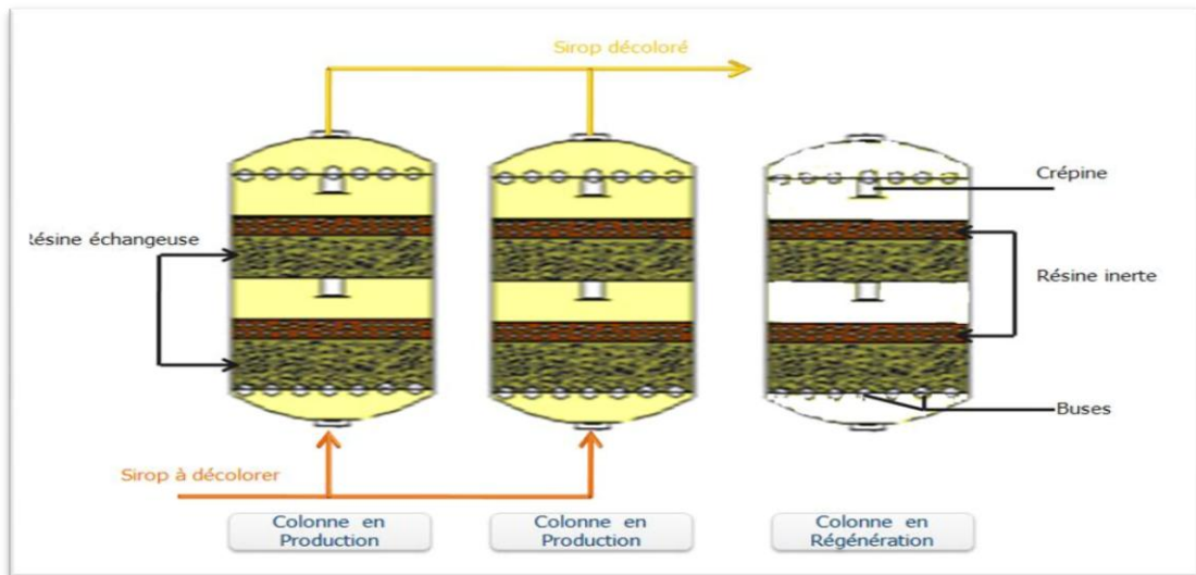
Figure 6 : Schéma de la chaîne de décoloration (colonnes 110).
