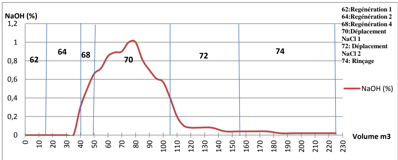
Figure 18 : Evolution de NaOH au cours de la régénération de la colonne après modification.
