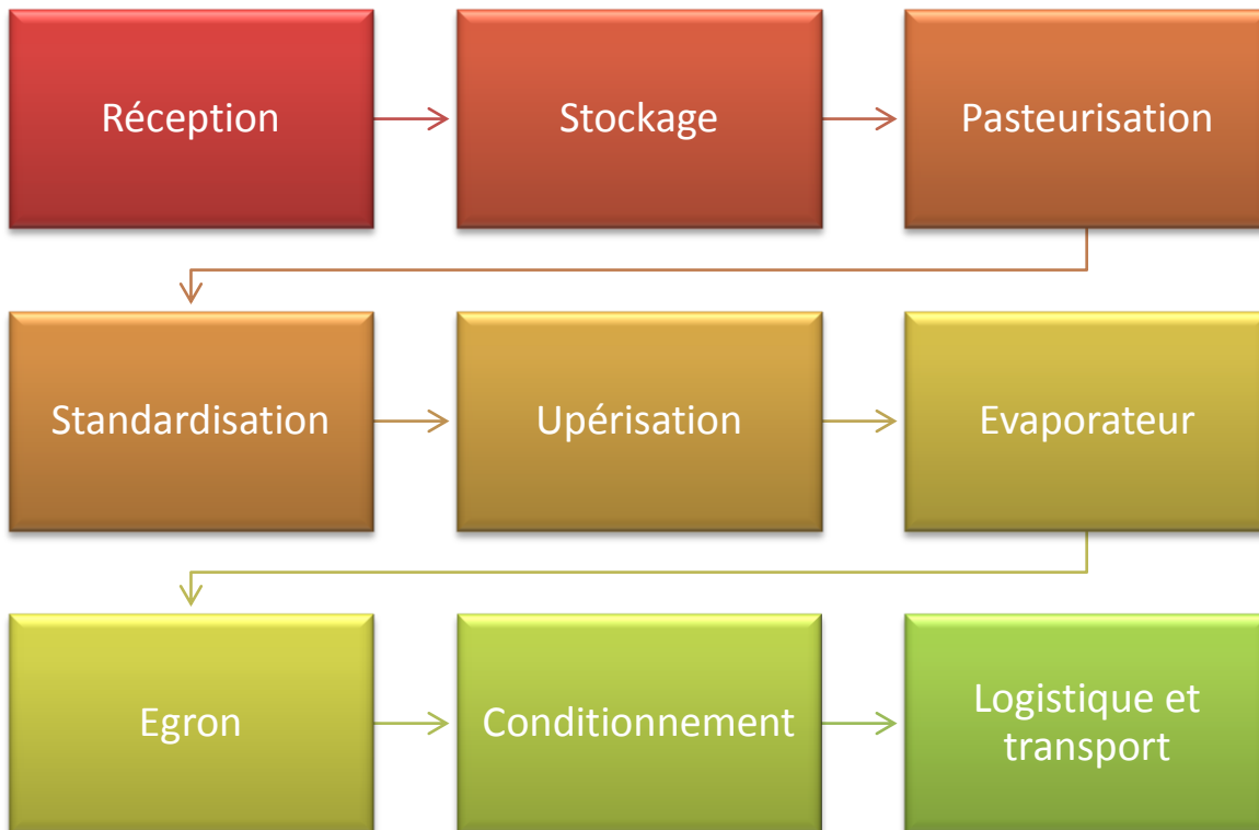
Figure 13 : Procédé de fabrication du lait en poudre
