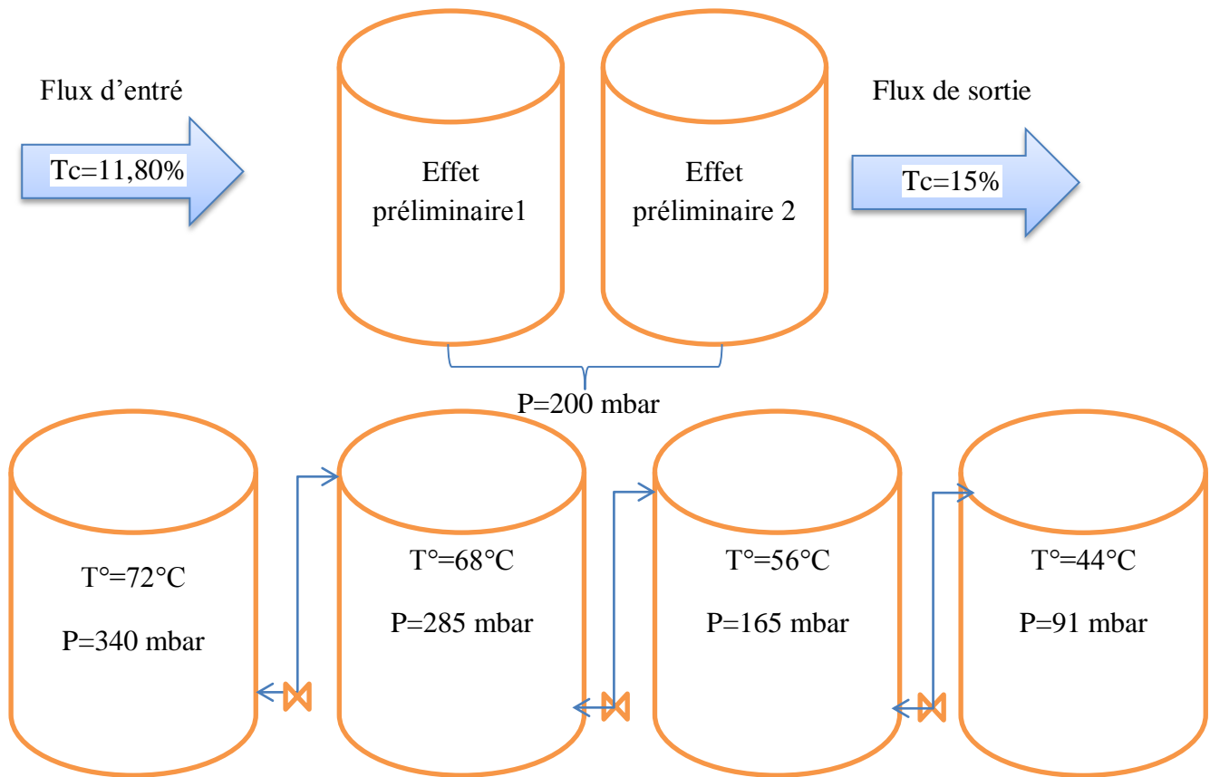
Figure 14 : Schéma simplifié des Six effets de l'évaporateur
