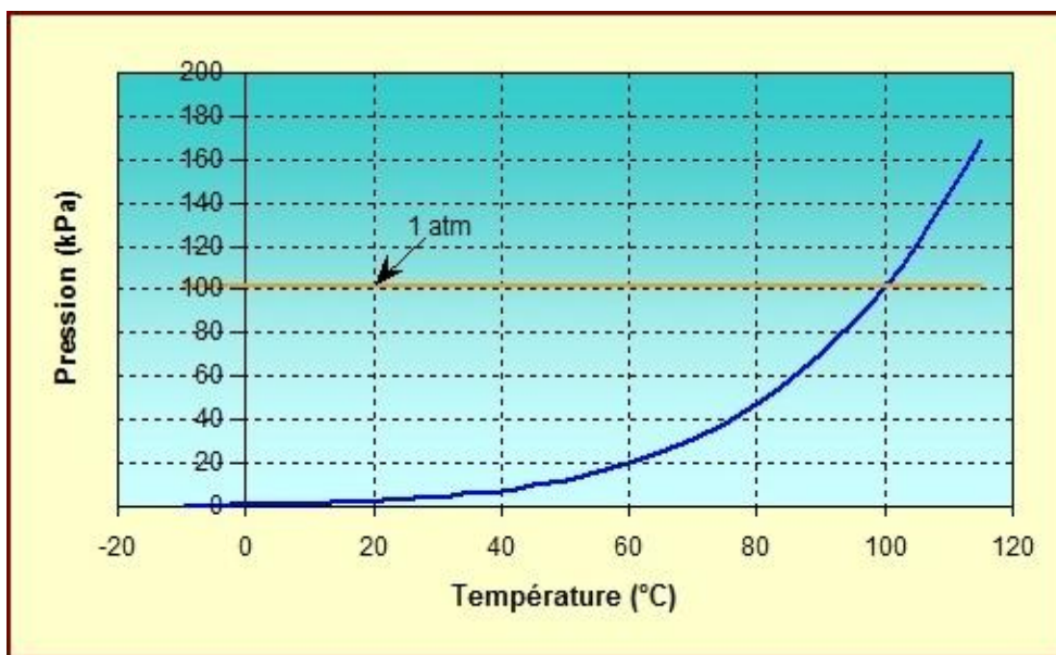
Figure 15 : Diagramme Pression-température
