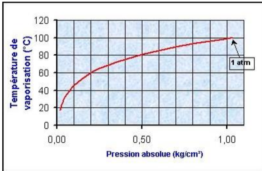
Figure 16 : Diagramme Pression-température à pression relative négatif
