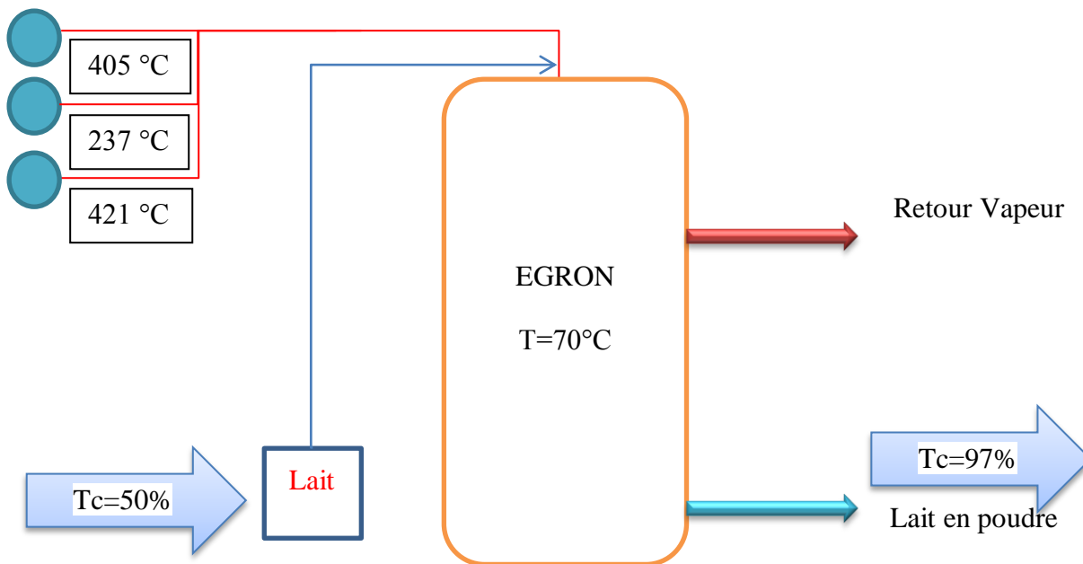
Figure 17 : Schéma descriptif de l'EGRON
