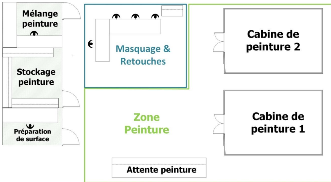
Figure 6 : Plan actuel de la zone peinture
