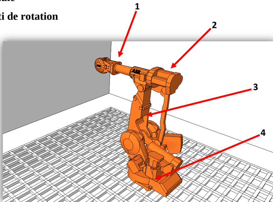
Figure 26: Conception 3D du robot proposé pour la peinture
