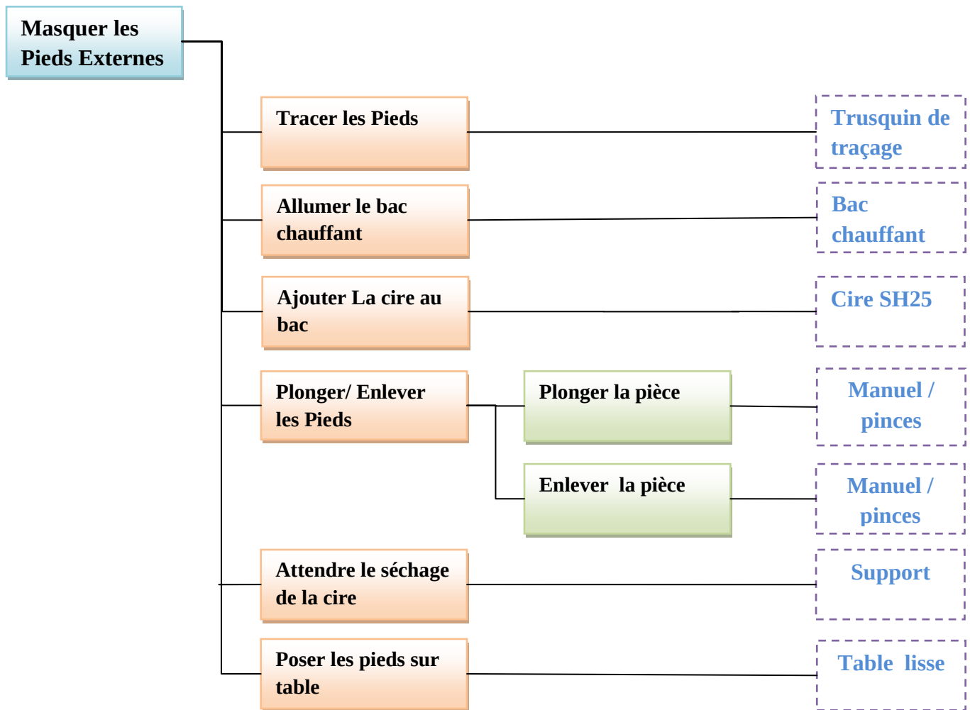
Figure 22 : Diagramme FAST du projet de masquage
