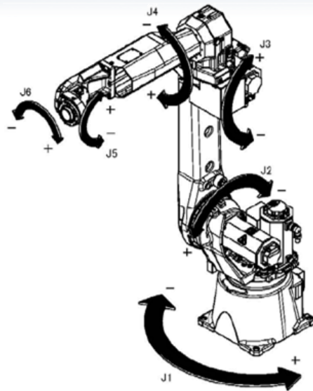
Figure 25 : Les 6 axes du bras robotique
