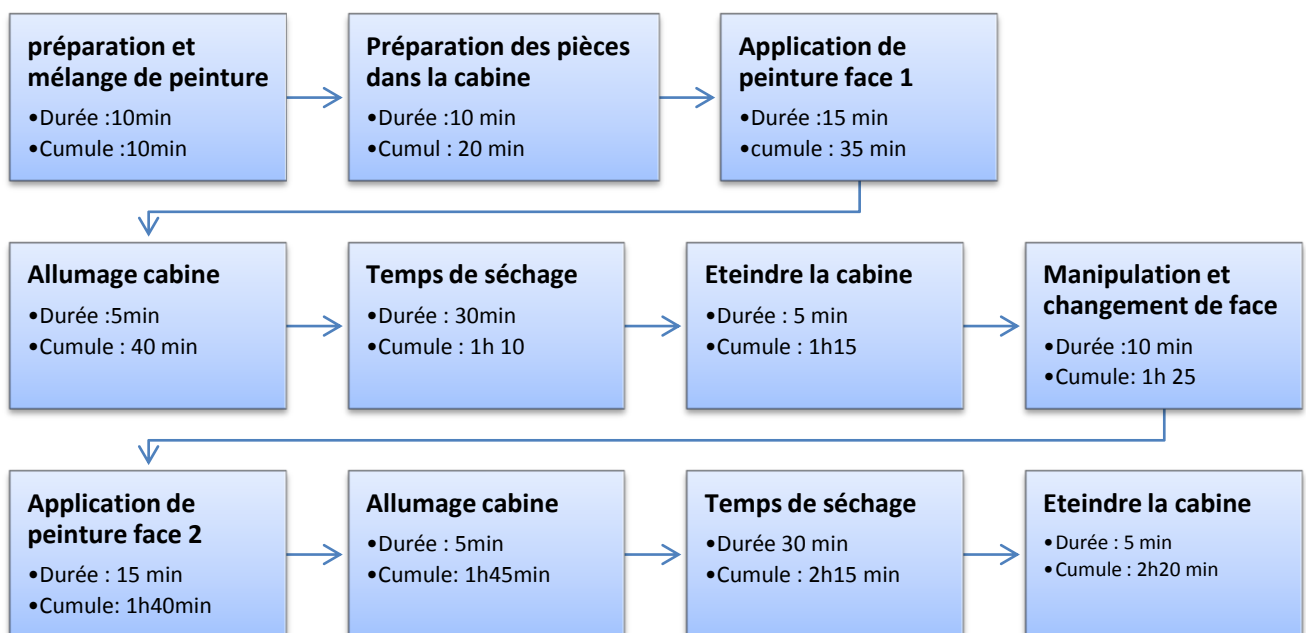
Figure 14 : Cycle de la cabine peinture pour F70
