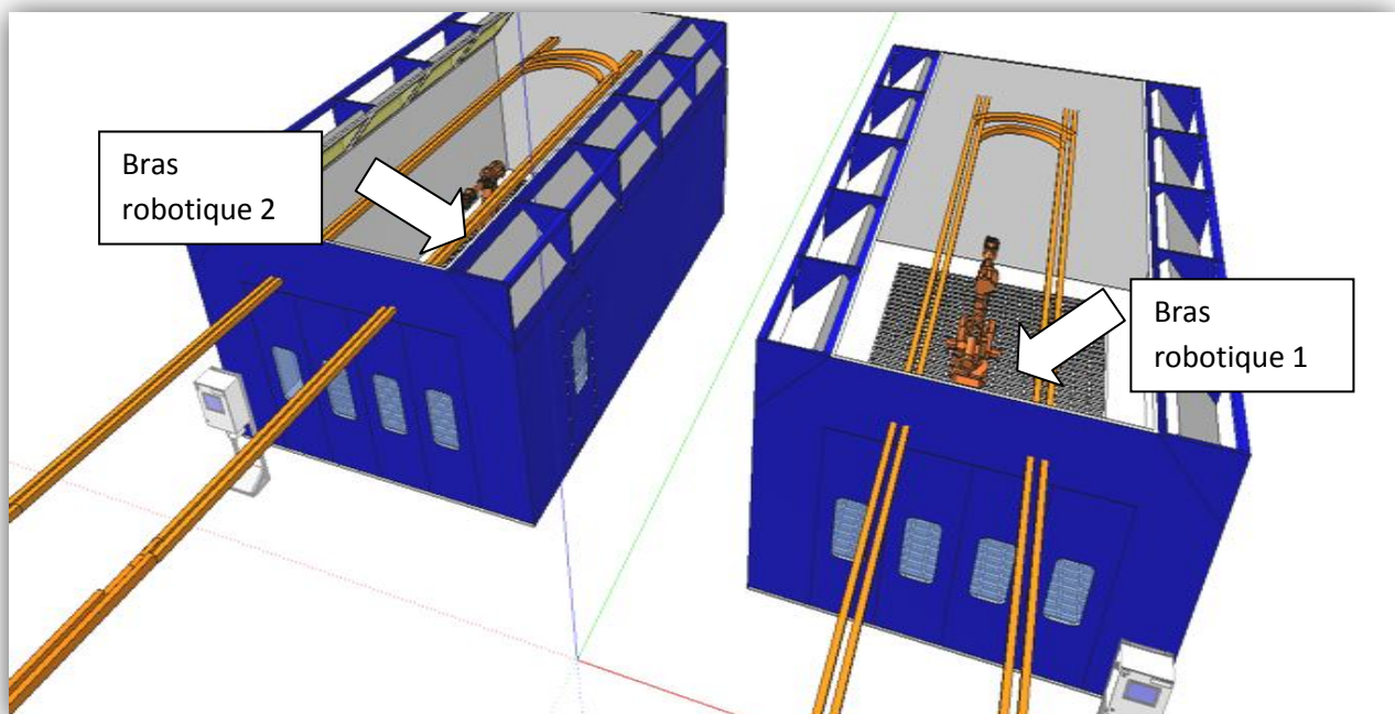
Figure 28: Conception de la robotisation de la zone peinture
