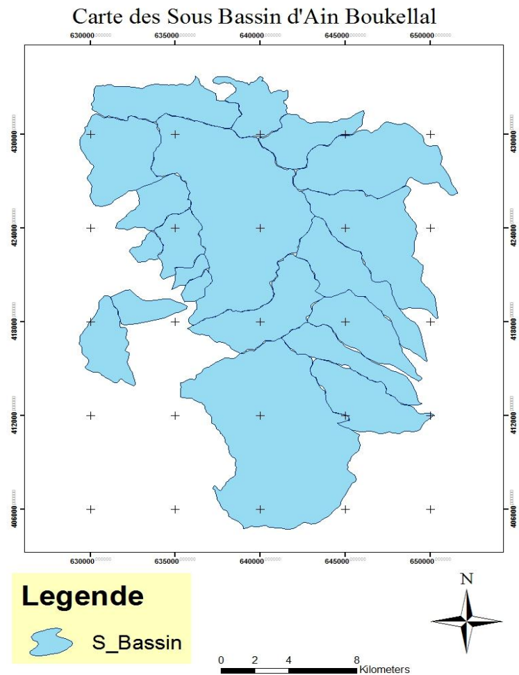
Figure 8 : Carte des sous bassins d'Ain Boukellal
