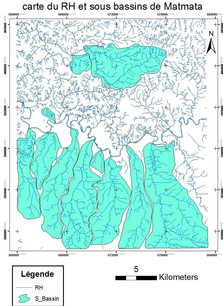
Figure 15 : Réseau hydrographique de type Parallèle de Matmata.:
