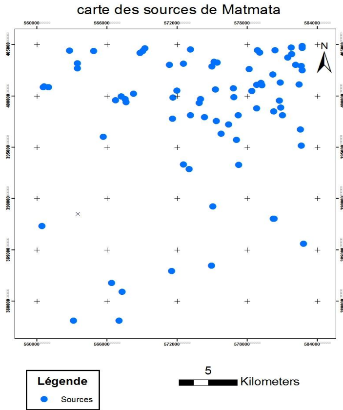
Figure 6 : Carte des sources de Matmata
