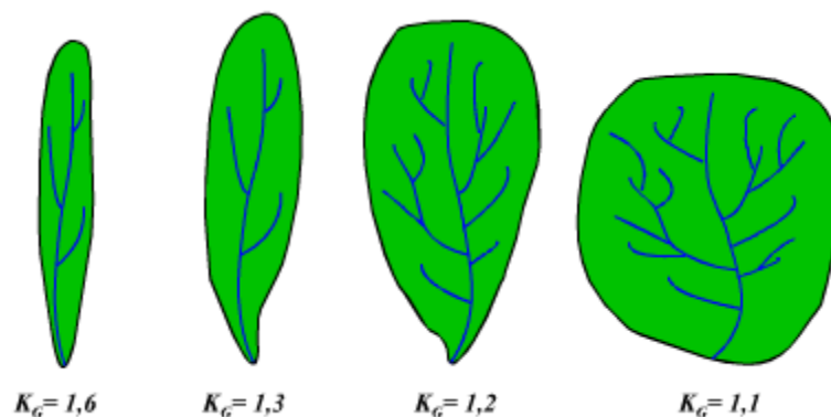
Figure 10 : exemple d'indice de compacité
