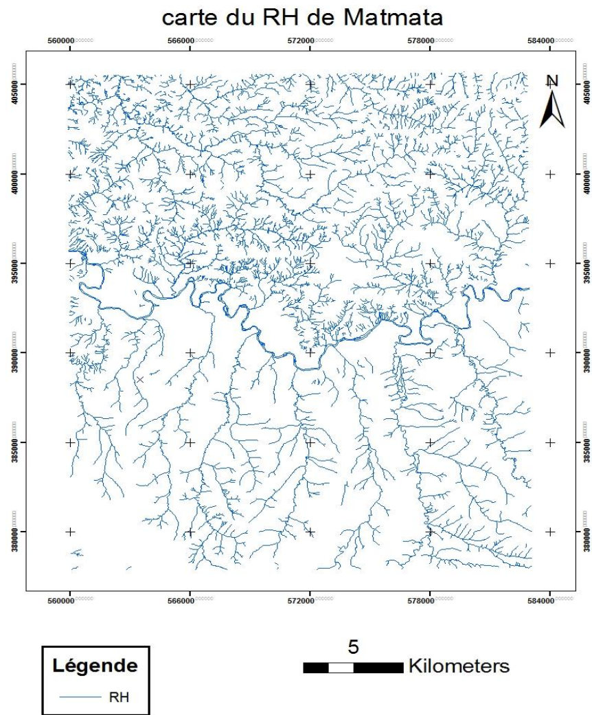
Figure 4 : carte du Réseaux Hydrographique de Matmata
