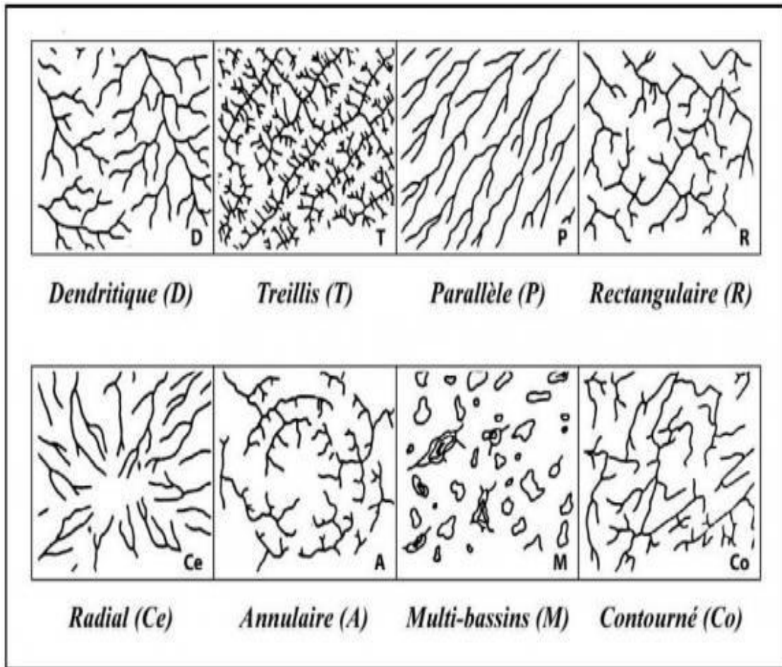
Figure 11 : Classification descriptive –types de base de réseaux hydrographiques (in B. DEFFONTAINES, 1990 ; d'après A.D. HOWARD, 1967).
