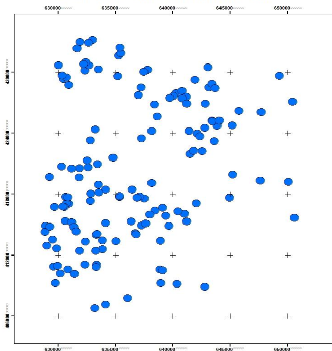
Carte des Sources d'Ain Boukellal
