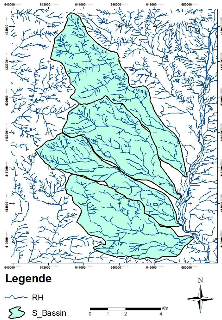
Figure 13 : Réseau hydrographiques de type parallèle d'Ain Boukellal
