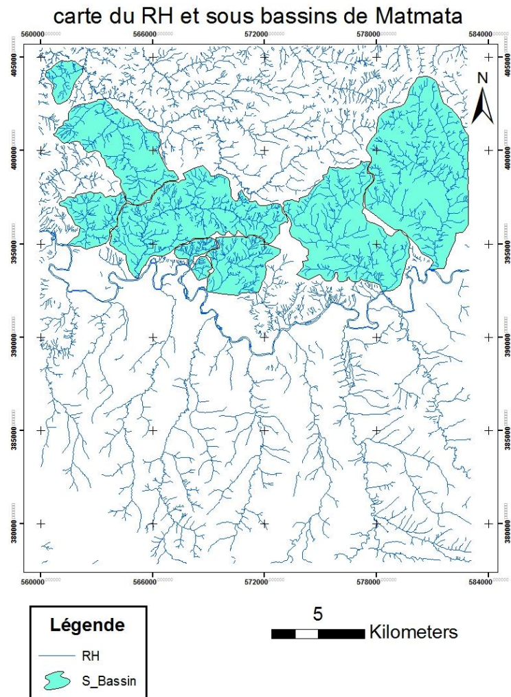
Figure 14 : Réseau hydrographique de type dendritique de Matmata
