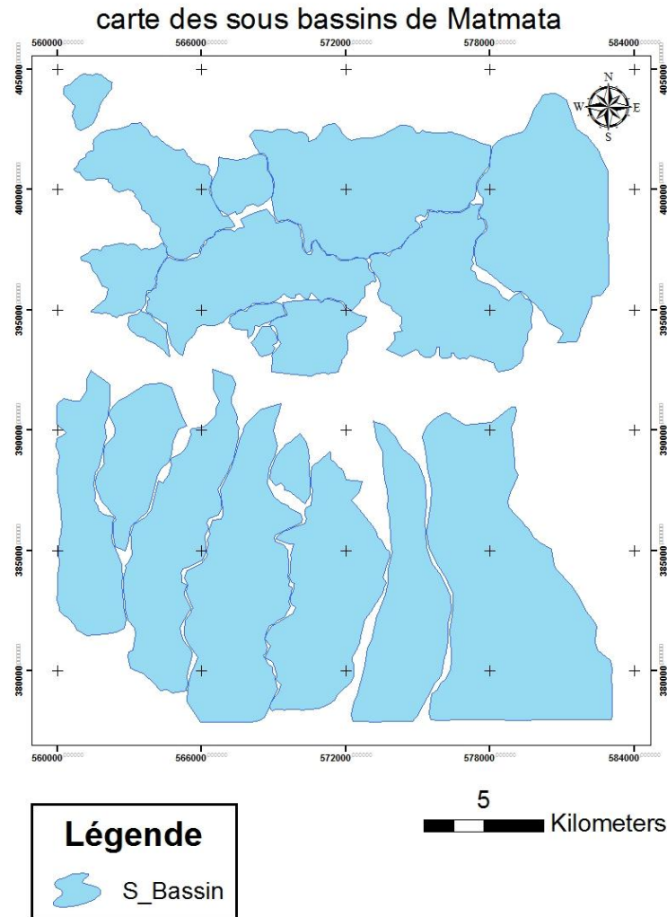
Figure 9 : Carte des sous bassins de Matmata
