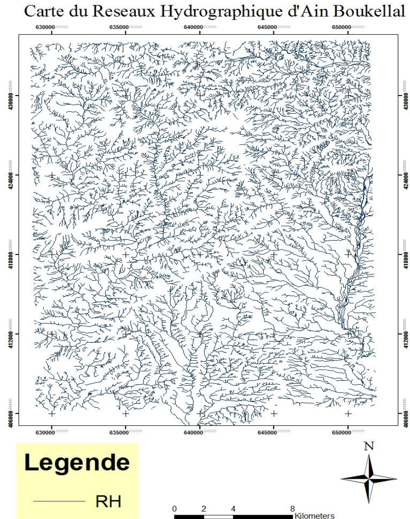
Figure 3 : carte du Réseau Hydrographique d'Ain Boukellal
