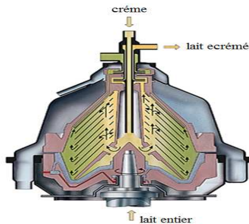
Figure 7 : Principe du fonctionnement d'une écémuse.
