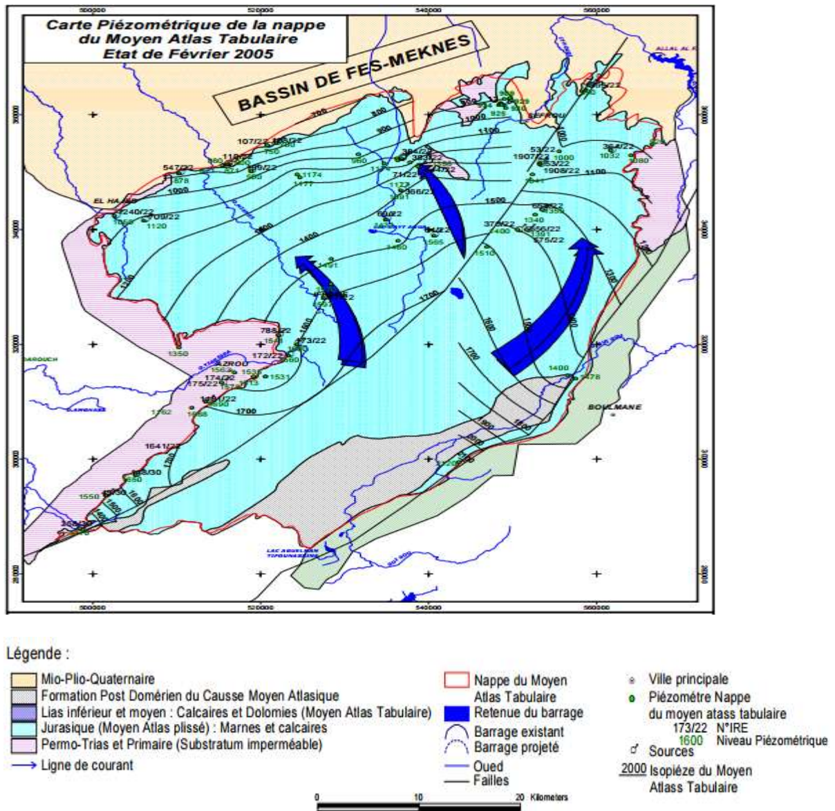
Fig. 9 : Carte Piézométrique de la nappe du Moyen Atlas tabulaire (PDAIRE Sebou-2007)
