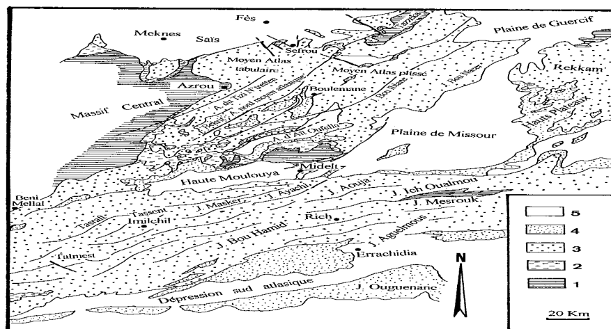
Fig. 2 : Carte géologique simplifiée du Moyen Atlas et du Haut Atlas central (d'après la carte géologique du Maroc au 1/1.000.000).
