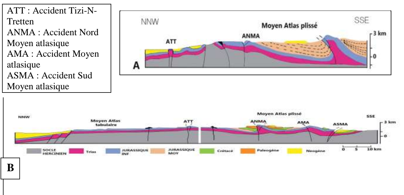
fig. 5 : coupes schématiques montrent les Accidents majeur entre le Moyen Atlas plissé et tabulaire (carte géologique du Sefrou, modifiée).
