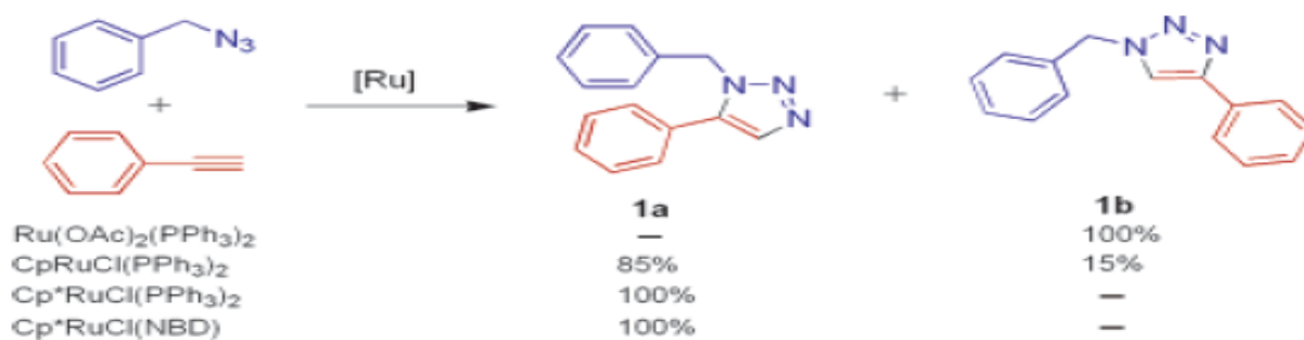
Schéma 20: Cycloaddition de l'azoture de benzyle avec le phénylacétylène catalysé par différents complexes à base de ruthénium [49] .
