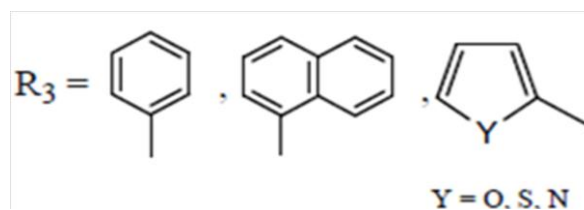
Schéma 10 : la préparation de dérivés de glycine portant en \alpha deux hétérocycles
