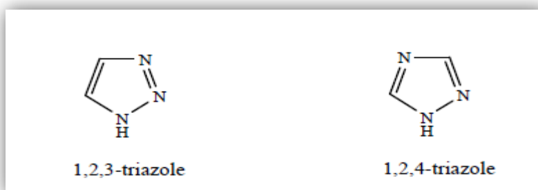
Schéma 1: Structure chimique de 1, 2, 3- et 1, 2, 4-triazoles.
