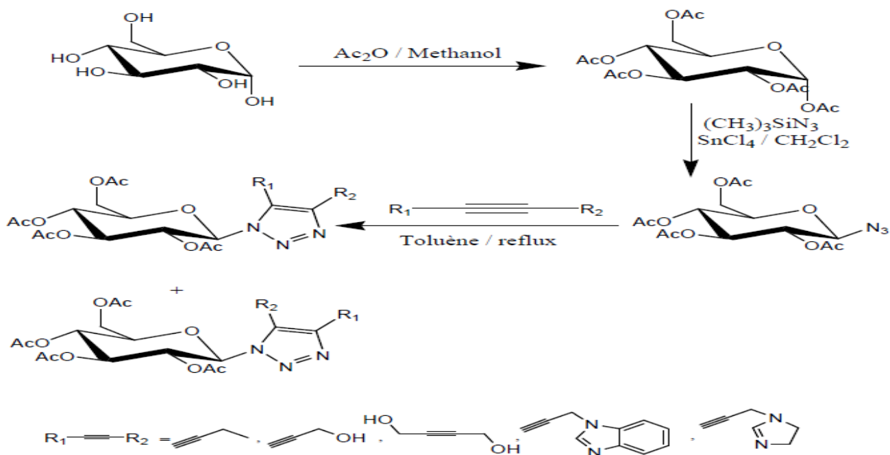
Schéma 13 : Synthèse de glycopyranosyl-1, 2,3-triazoles
