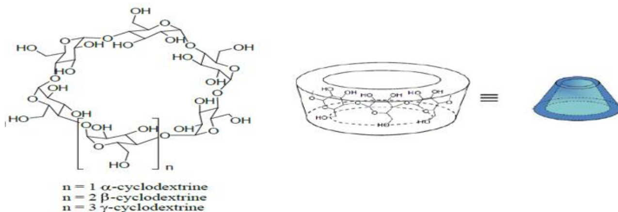
Figure 8: Formule générale des cyclodextrines et représentation schématique de la structure tridimensionnelle.
