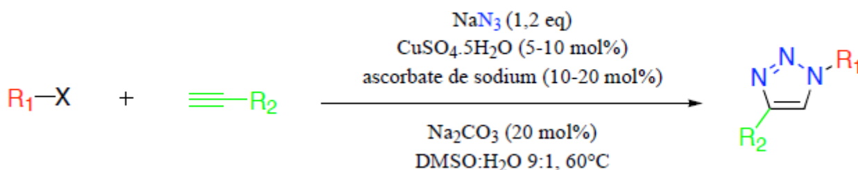
Schéma 21: Synthèse « one-pot » de 1, 2, 3,-triazoles [54] .
