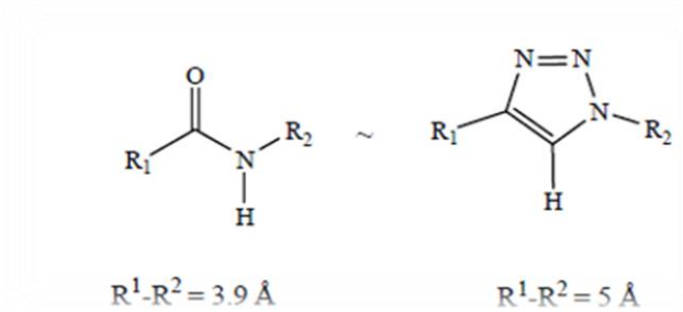
Schéma 2 : Similitudes topologiques et électroniques entre les unités amides et 1,2,3-triazole [15] .
