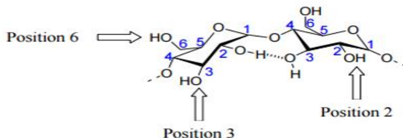
Schéma 31: localisation des hydroxyles sur une unité de \alpha -D-glucose et interaction inter-unité.
