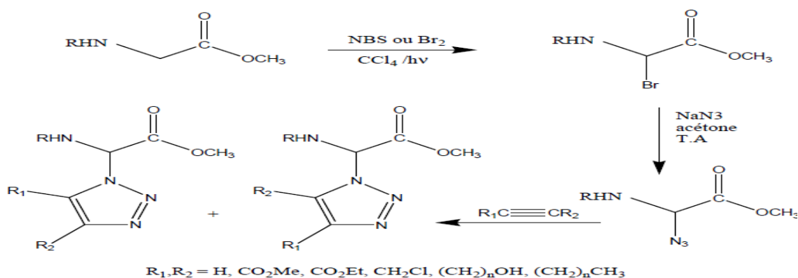
Schéma 9 : Synthèse d' \alpha -triazolyl- \alpha -aminoesters
