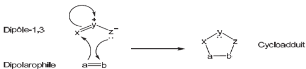
Schéma 3: Schéma simplifié de cycloaddition 1,3-dipolaire.
