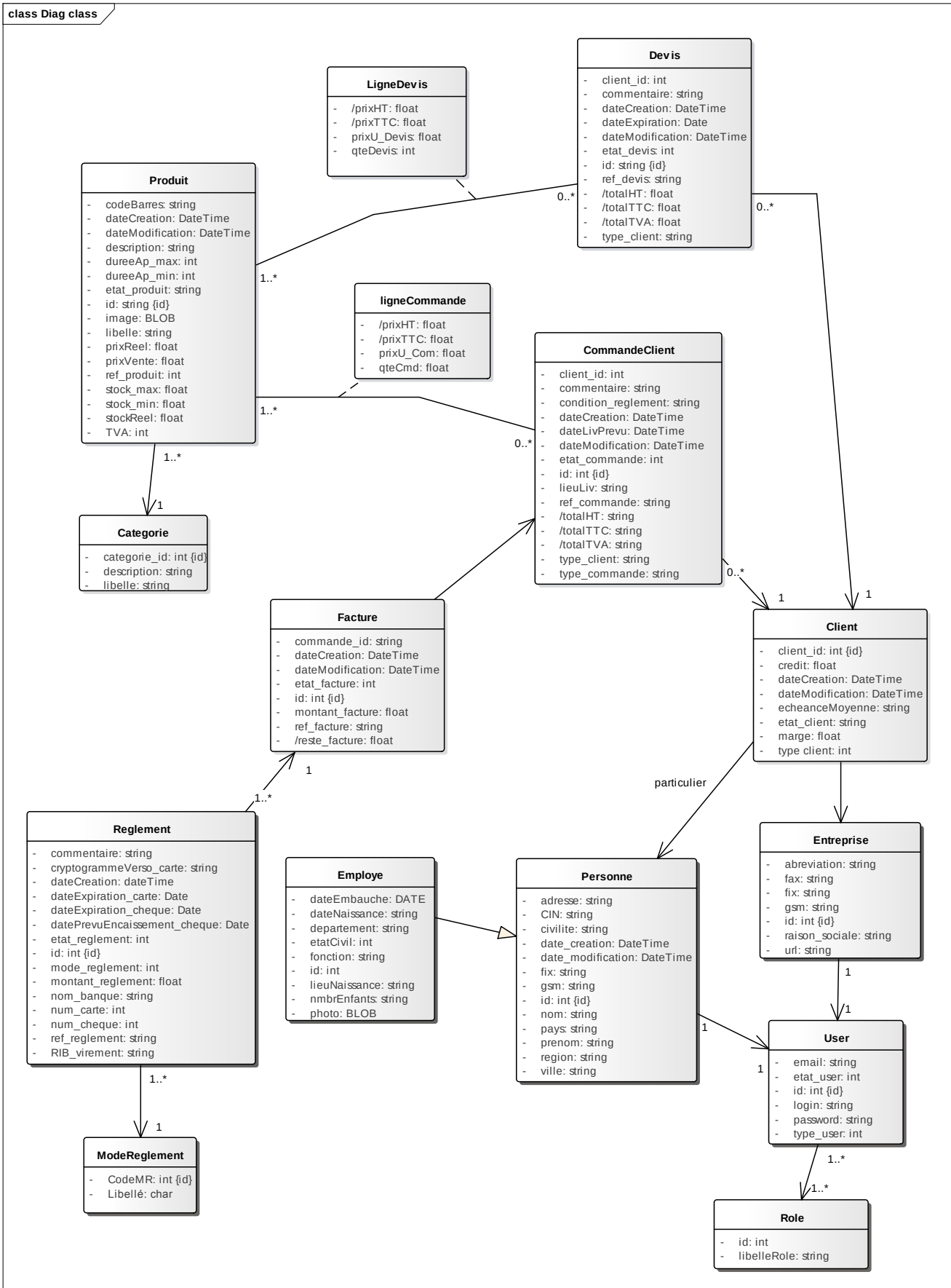
Figure 10 : Diagramme de classes
