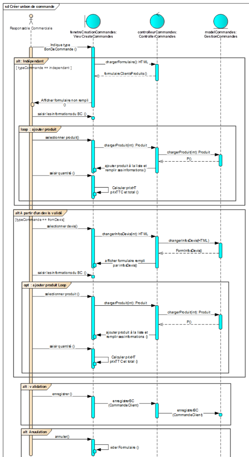
Figure 11 : Diagramme de séquence pour la création d'un bon de commande ( Resp.Commercial )
