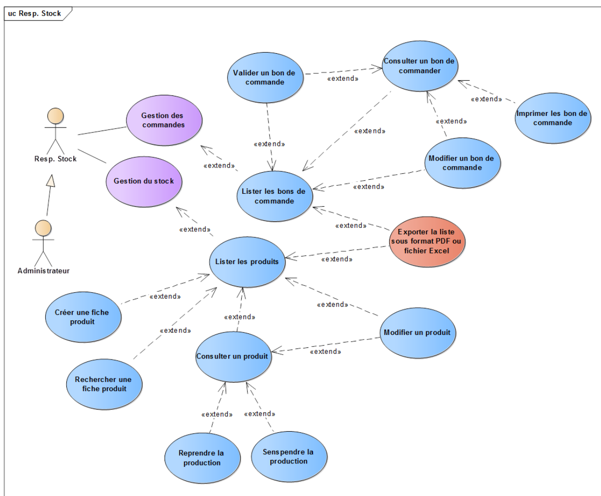
Figure 7 : Diagramme de cas d'utilisation pour le responsable de stock
