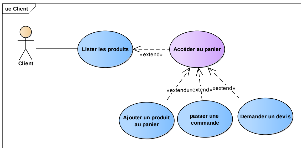
Figure 8 : Diagramme de cas d'utilisation pour le client
