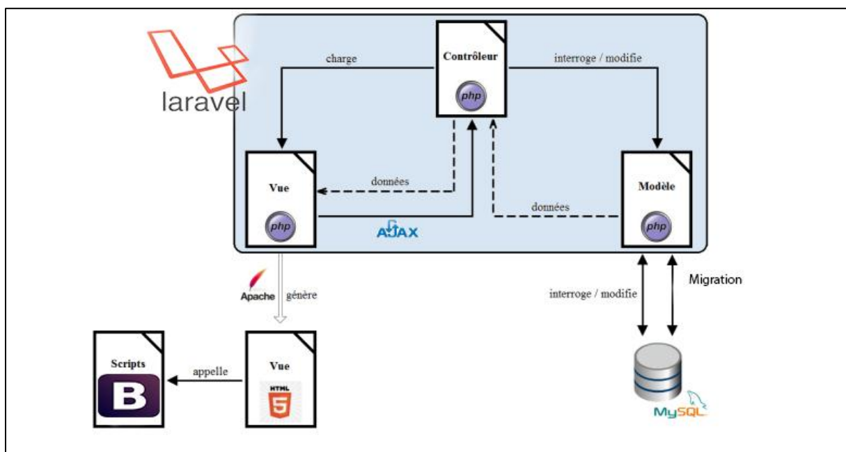
Figure 13 : schéma d'exécution d'un script avec le pattern MVC de Laravel
