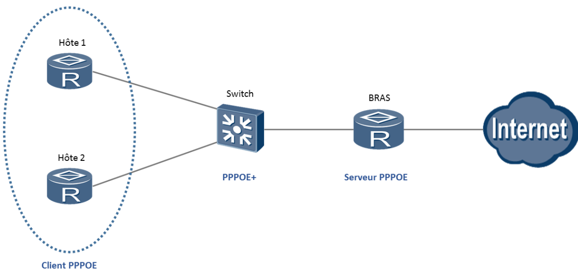
Figure 61: Réseau PPPoE+.
