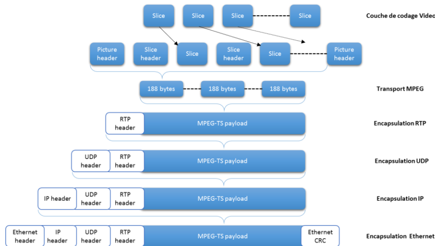
Figure 15: Encapsulation d'un paquet vidéo en IPTV. [6]
