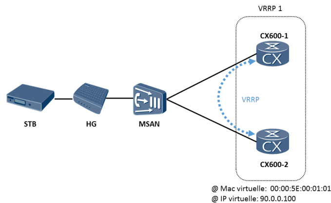
Figure 81: Implémentation du VRRP entre les deux routeurs CX600 de la boucle METRO IP.
