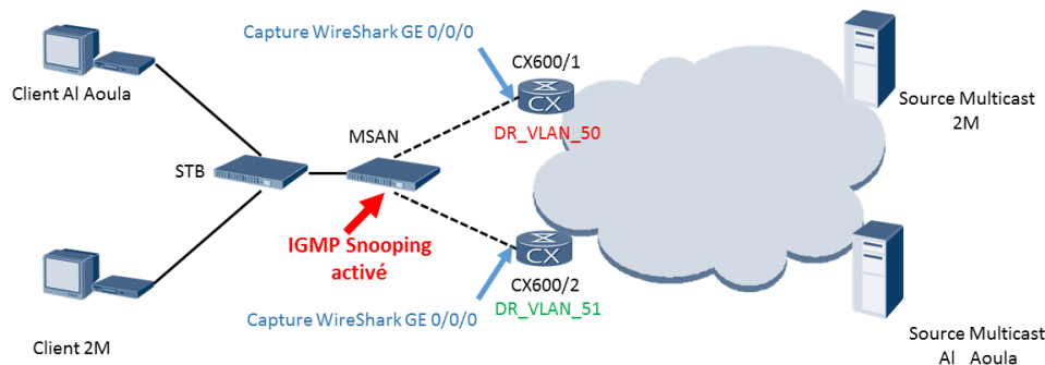
Figure 45: Specification du DR de chaque VLAN.
