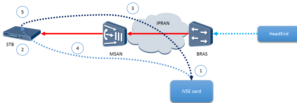
Figure 16: Processus d'implémentation de la RET. [6]
