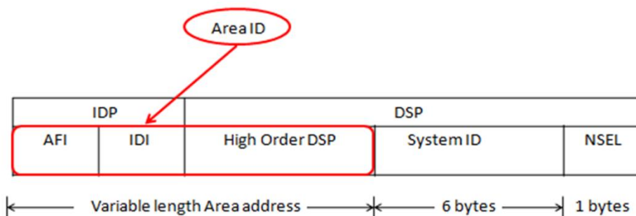
Figure 67: Format de l'adresse NSAP. [15]
