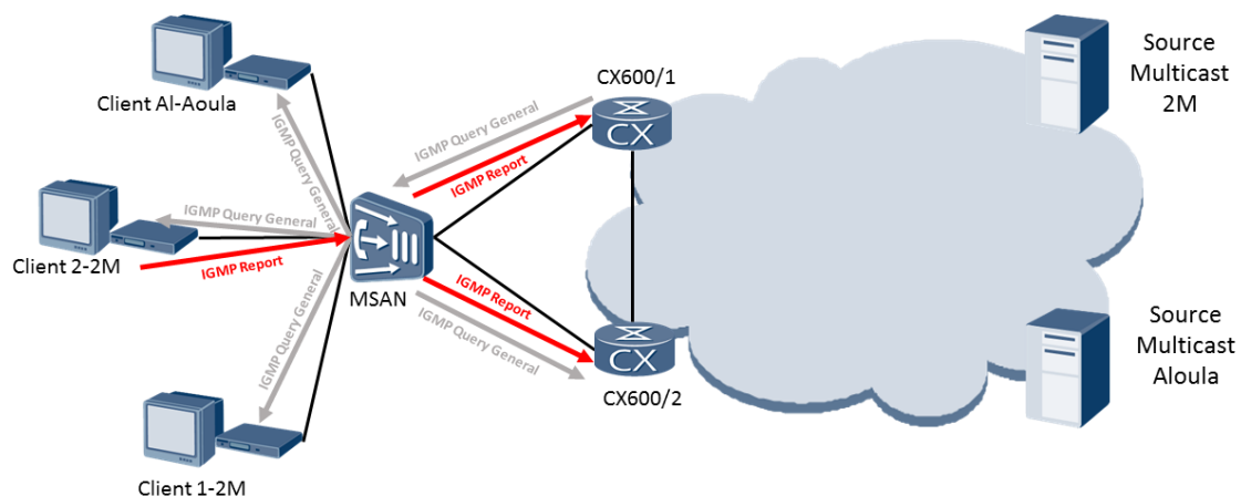
Figure 36: Principe de fonctionnement de l'IGMP.
