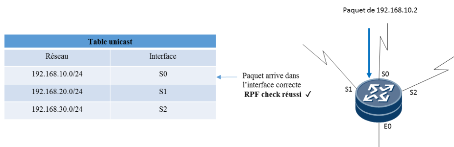
Figure 24: RPF check réussi. [4]
