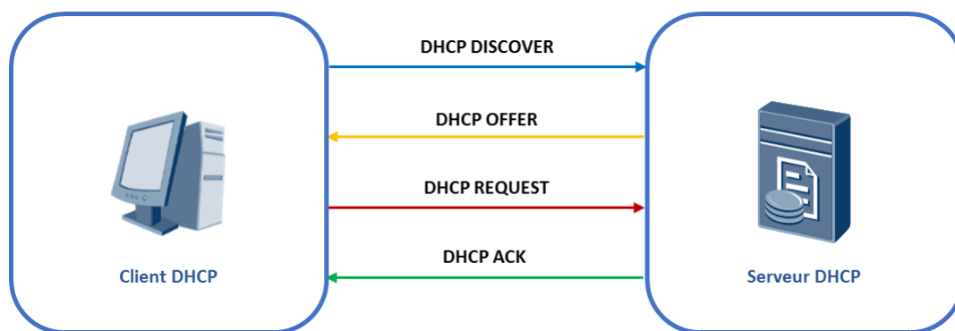
Figure 63: Processus d'affectation d'adresses IP en utilisant DHCP.
