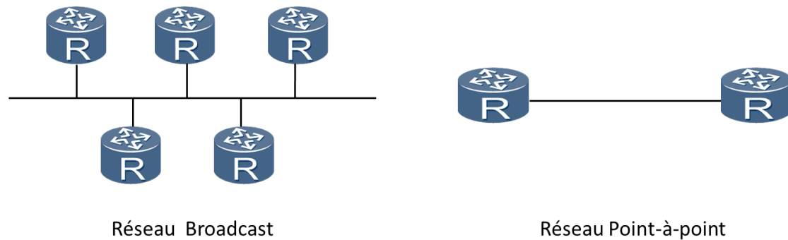
Figure 68: Types des réseaux IS-IS.
