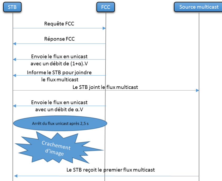
Figure 53: Mécanisme du Zapping.
