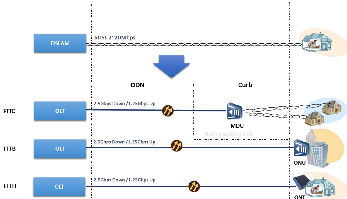
Figure 92: Passage d'une architecture d'accès xDSL aux architectures optiques FTTx. [18]
