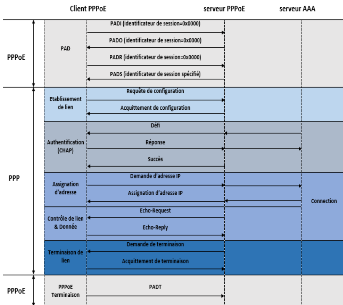
Figure 60: Cycle de vie d'une session PPPoE. [5]
