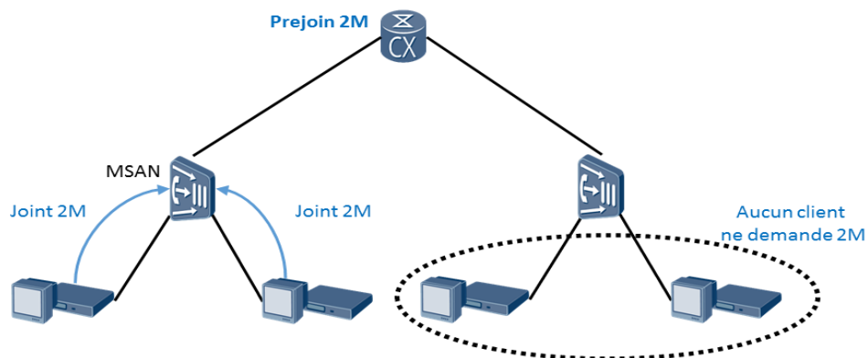
Figure 54: Demande d'une chaîne par MSAN.
