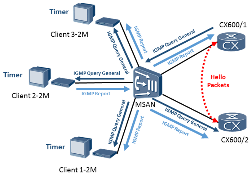
Figure 50: Principe de fonctionnement du protocole IGMP.
