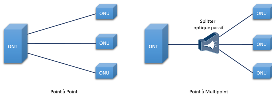
Figure 93: Architecture point à point et architecture point à multipoint.
