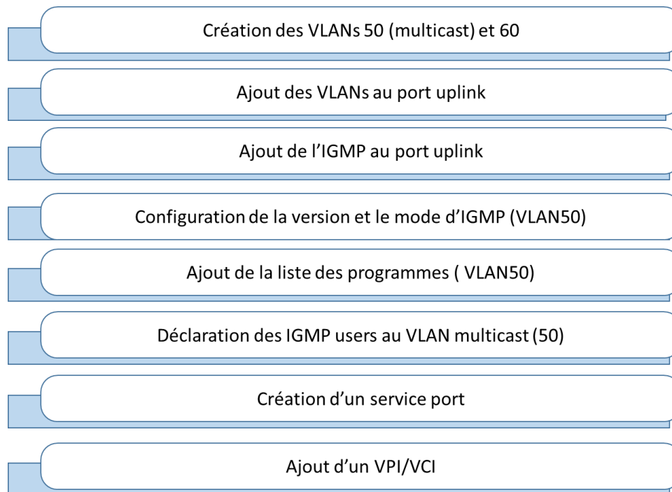
Figure 37: Etapes de configuration du VLAN de multicast au niveau du MSAN.
