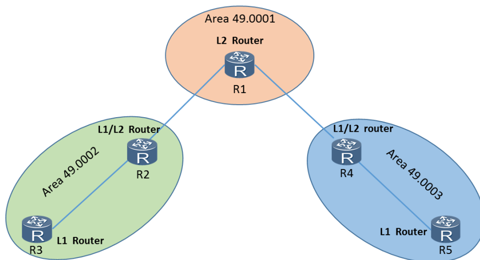
Figure 66: Exemple d'une architecture ISIS sur GNS3.
