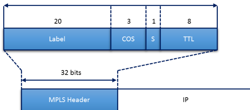
Figure 77: Format de l'entête MPLS. [15]
