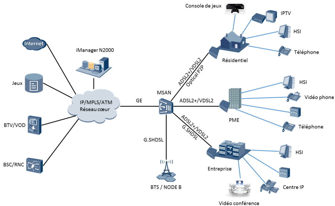
Figure 33: Services supportés par le MSAN.
