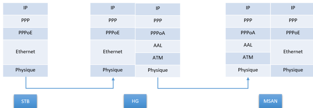
Figure 34: Processus d'encapsulation sur ATM.
