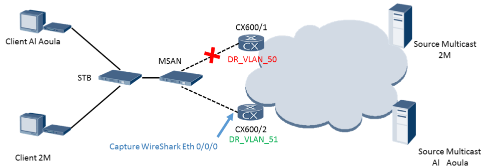
Figure 48: Simulation du basculement vers le nouveau DR.
