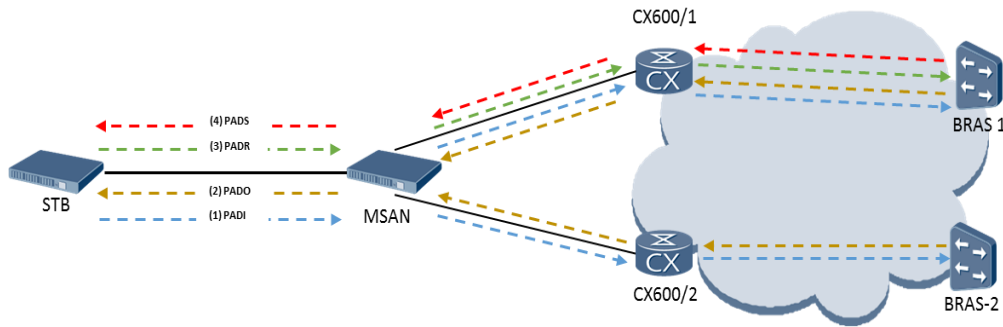
Figure 31: Messages d'établissement de la session PPPOE.
