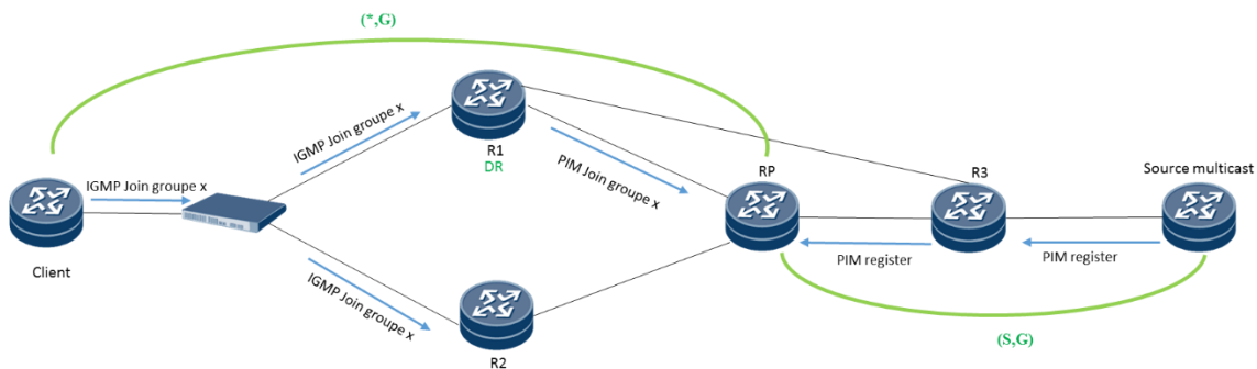
Figure 26: Fonctionnement du PIM-SM.
