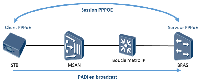
Figure 30: Session PPPOE entre le STB et le BRAS.
