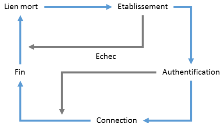
Figure 58: Diagramme d'états de la session PPP. [16]
