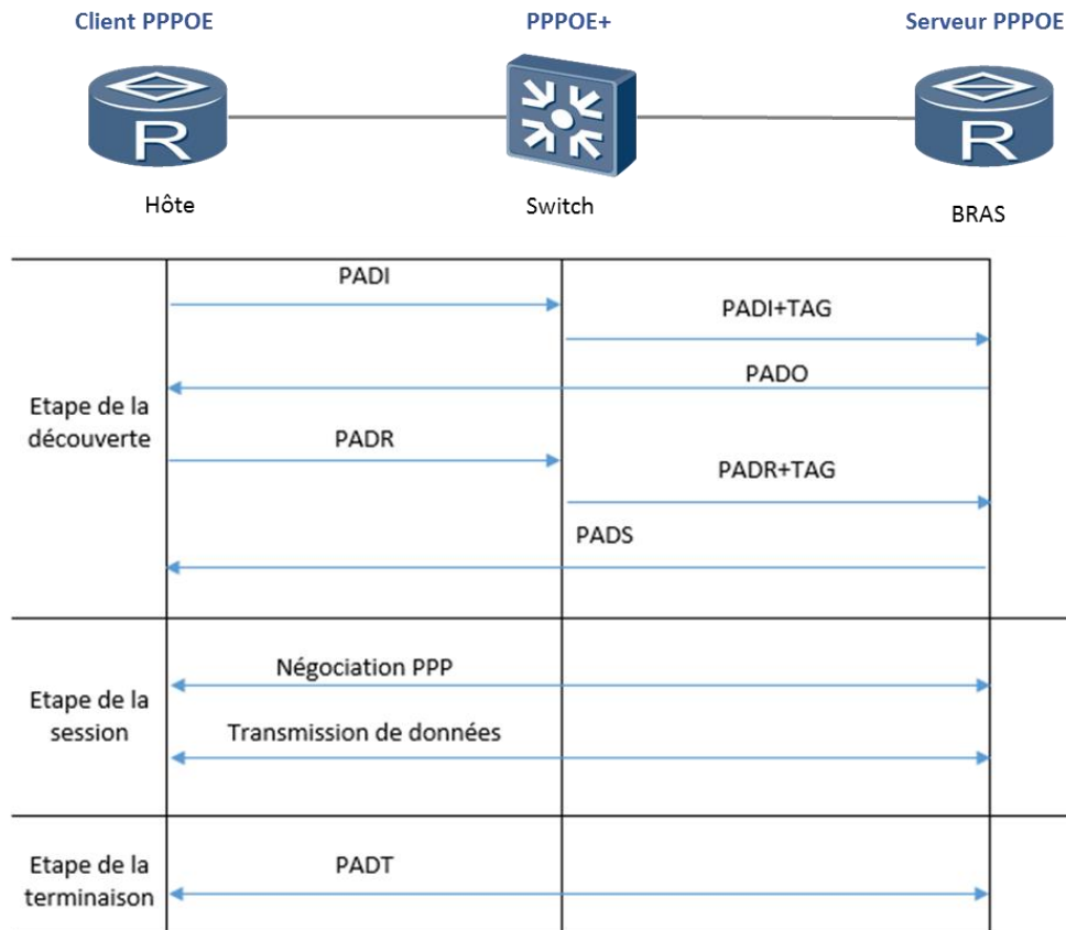
Figure 62: Le processus de fonctionnement du PPPoE+.
