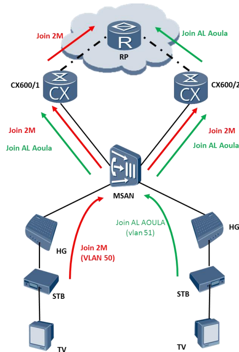
Figure 43: Description de la solution de partage de charge.
