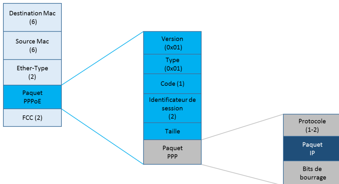
Figure 59: Forme du paquet PPPoE. [5]
