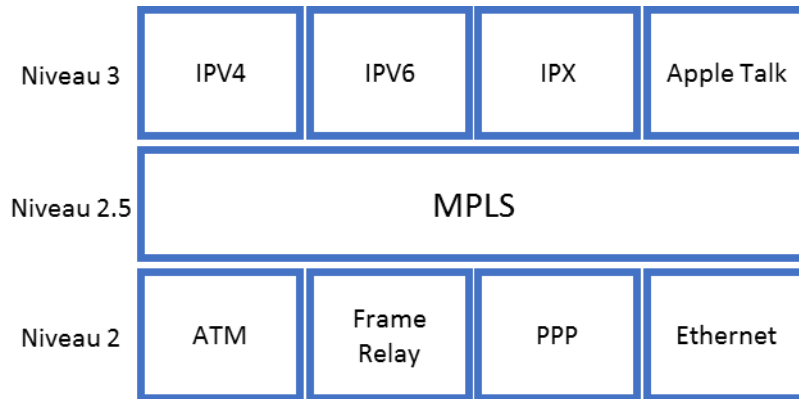
Figure 76: MPLS dans la pile TCP/IP. [15]
