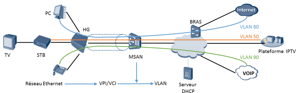
Figure 35: Mapping entre VPI/VCI et VLAN.
