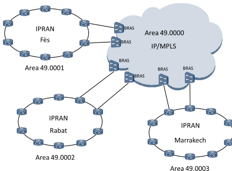
Figure 28: Implémentation du protocole IS-IS.
