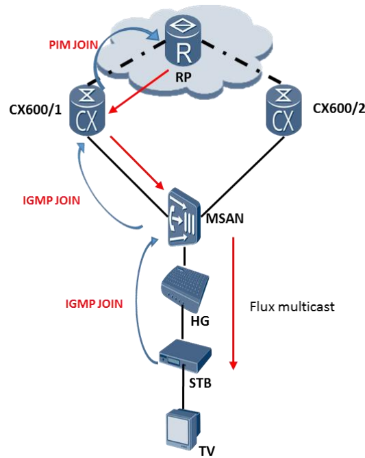
Figure 42: Passage du flux après élection du DR.
