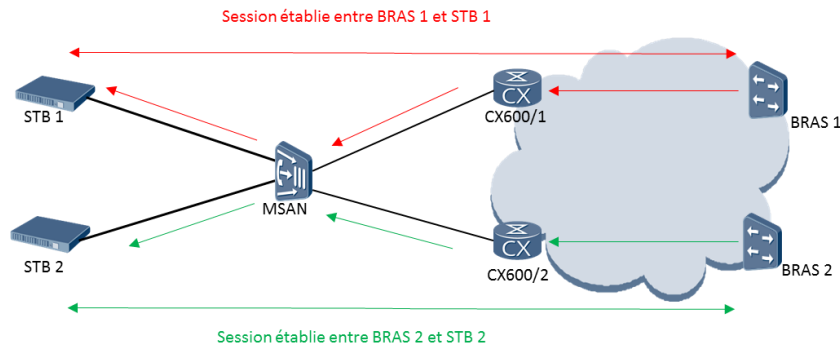
Figure 32: Partage du flux Unicast entre les routeurs CX600/1 et CX600/2.
