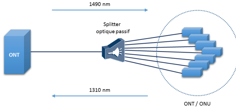
Figure 94: Multiplexage WDM en GPON.
