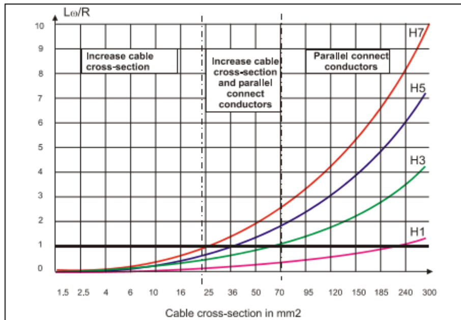
FIG. 3.12. EFFET DE LA SECTION DU CABLE SUR LQ/R
