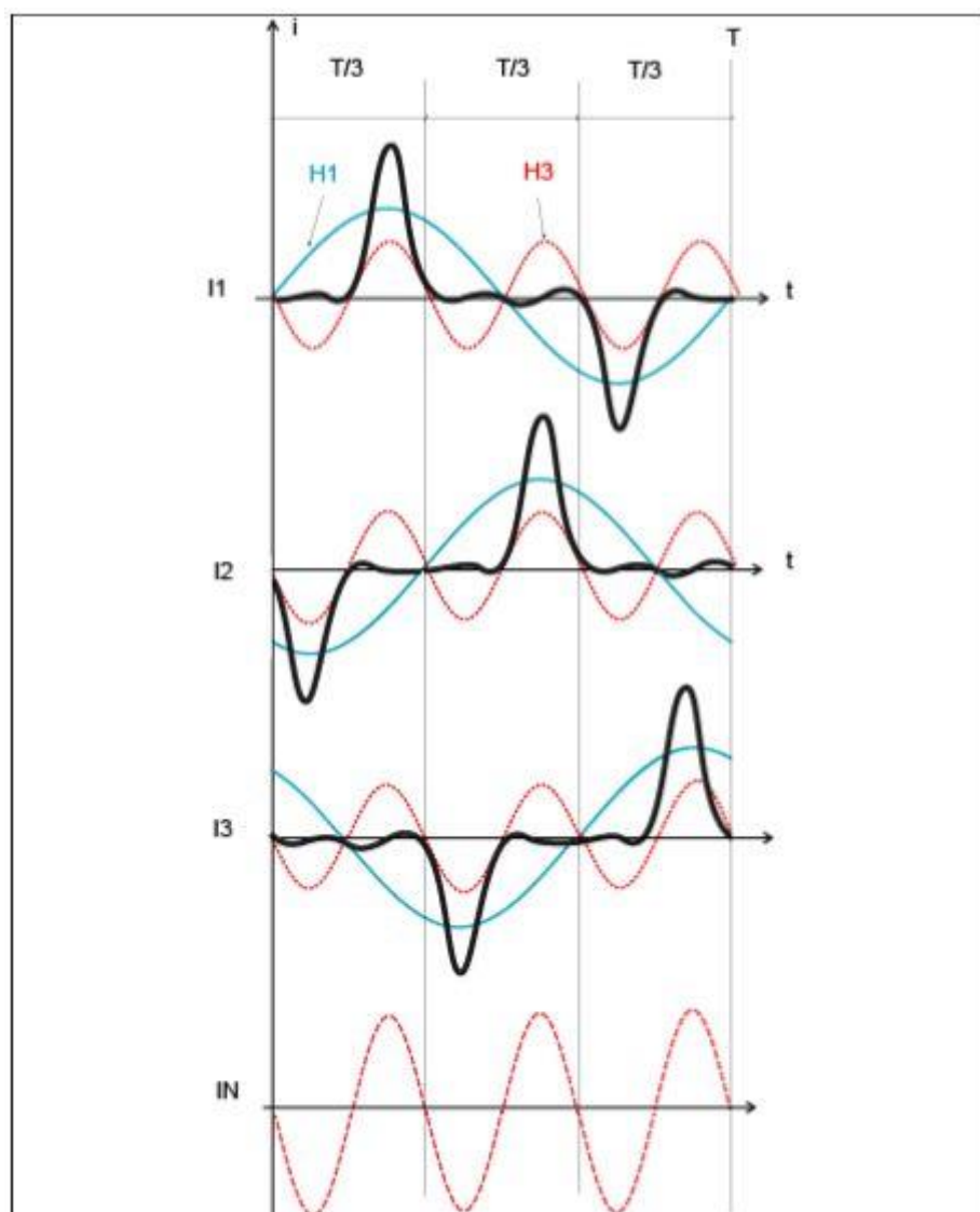
FIGURE 3.5 : LES HARMONIQUES DE RANG 3 ET LEURS MULTIPLES S'ADDITIONNENT DANS LE CONDUCTEUR NEUTRE.
