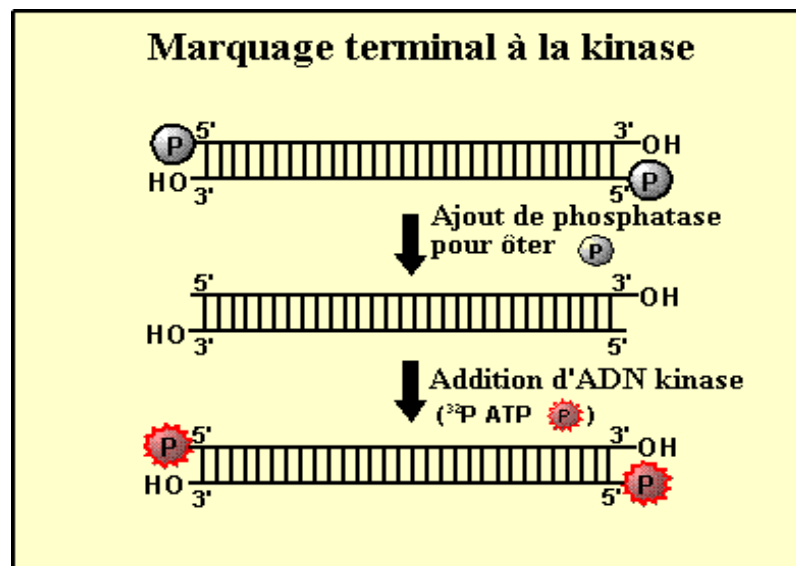
Figure 4 : Marquage en 5' (13).
