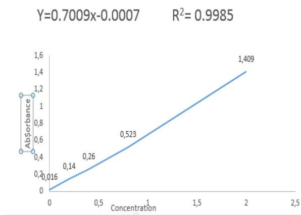
Figure 1 : Courbe d'étalonnage des nitrates
