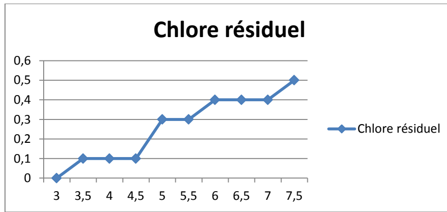
Figure 3 : Courbe du chlore résiduel
