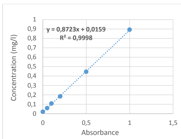
Figure 2 : Courbe d'étalonnage d'ammonium
