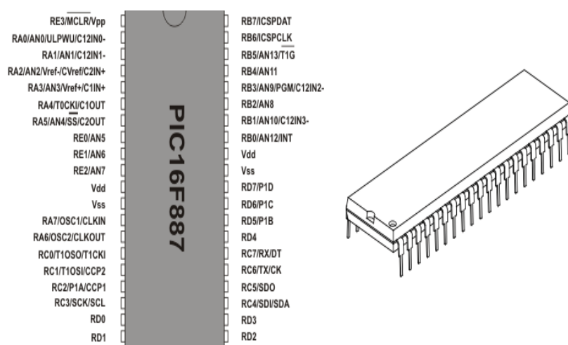
Figure 30 : Le microcontrôleur PIC167887
