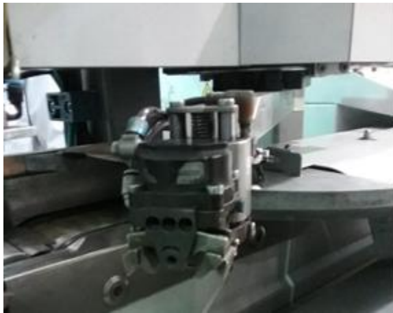
Figure 21 : Unité de pivotement et d'extraction et pince cotée 2
