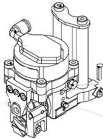
Figure 21 : Unité de pivotement et d'extraction et pince cotée 2
