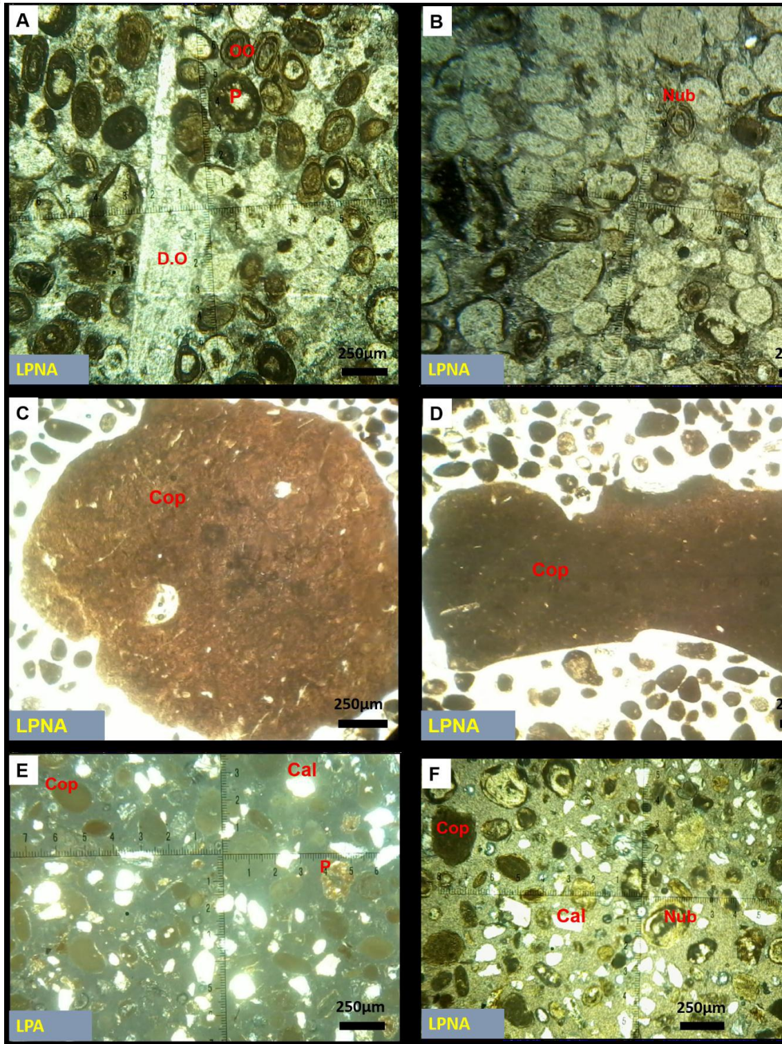
Figure .III.1 : Vue microscopique des quatre principaux composants phosphatés des niveaux étudiés. (OO : oolithes ; P : Pellets ; D.O : Débris Osseux ; Nub. : Nubéculaires ; Cop : Coprolithes ; Cal. : Calcite) (ANAJJAR Ahmed (2005)).
