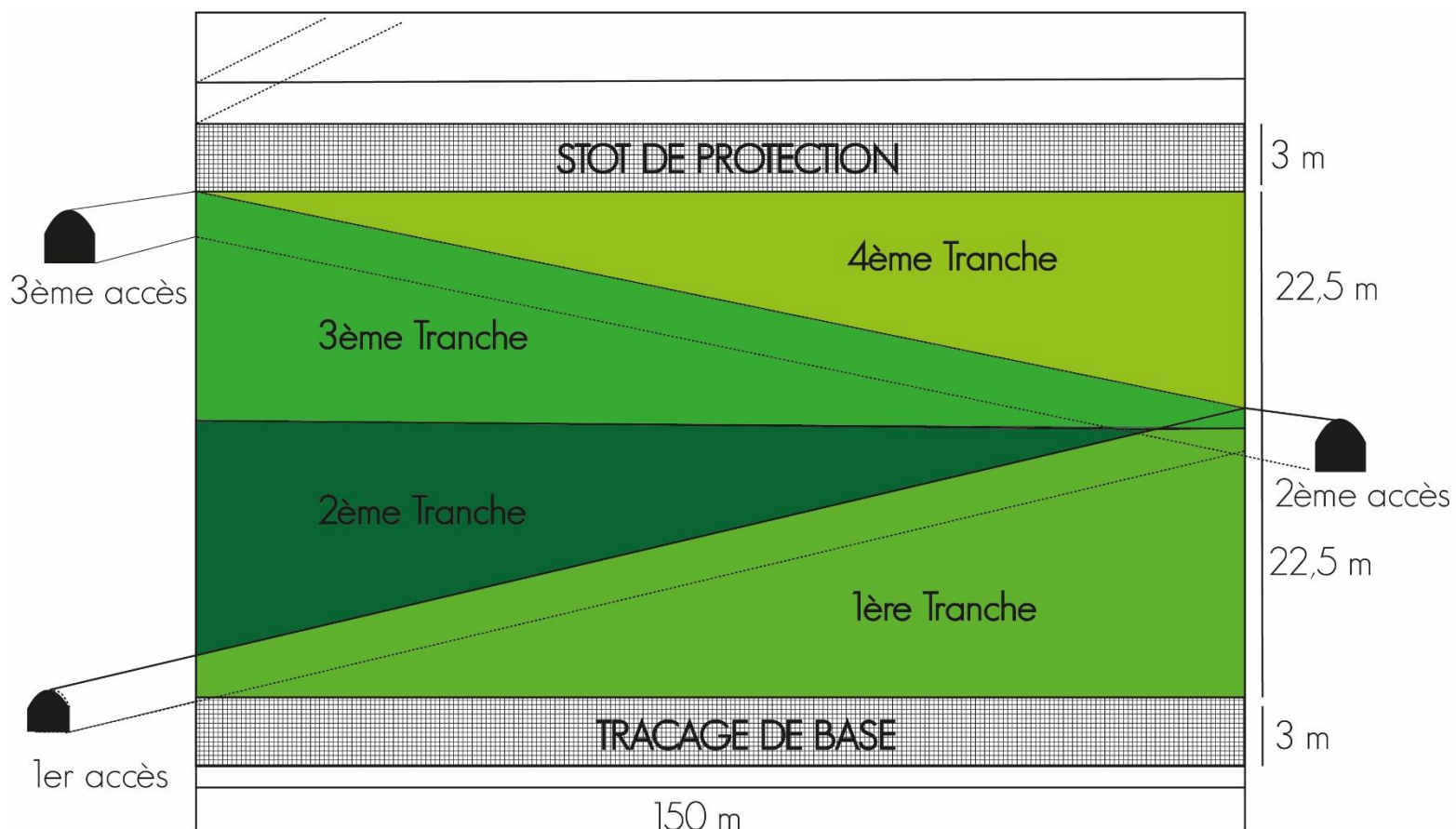
Figure 10 : Exploitation du panneau minéralisé par la méthode TMR
