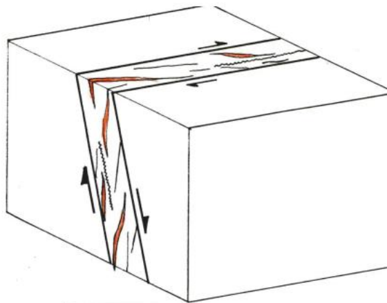
Figure 24 :Schéma du modèle structural d'ouverture des structures étudiées
