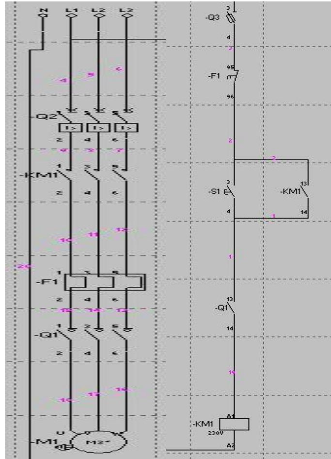
Figure 28 :schéma de puissance et de commande d'un seul ventilateur
