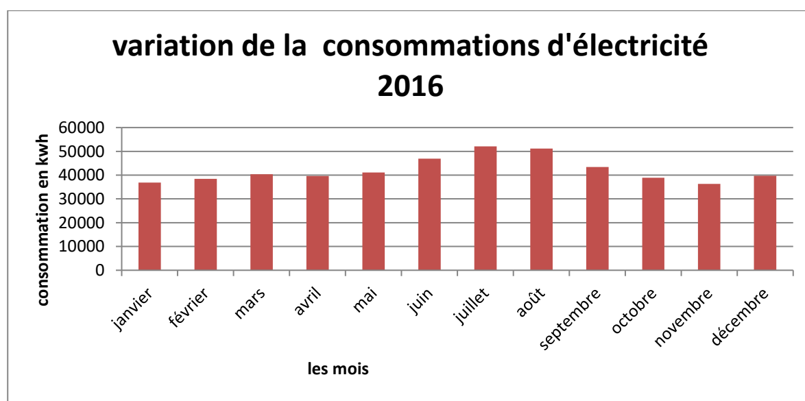
Figure 16 : Répartition de la consommation en fonction des mois 2016
