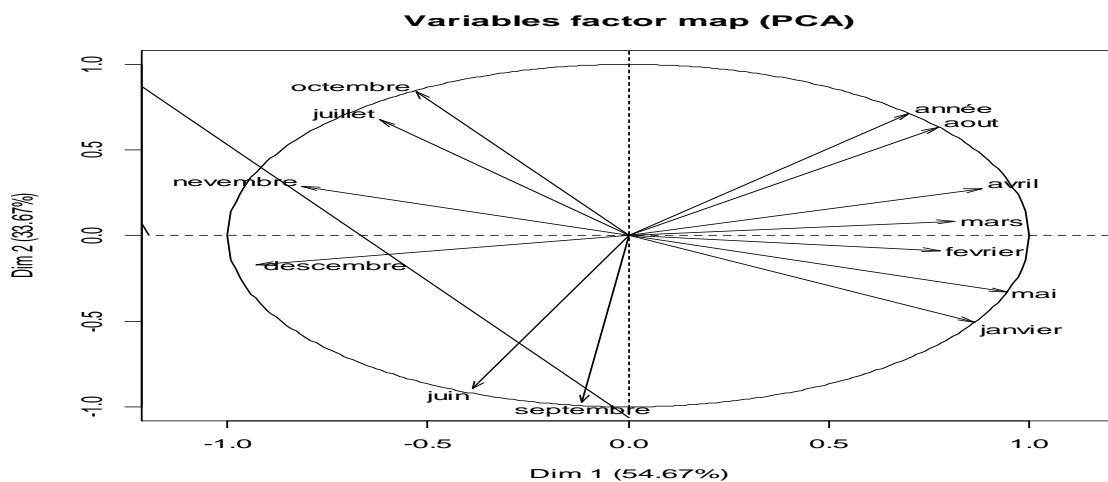
Figure 23 : Cercle de corrélation de l'ACP pour les industriels
