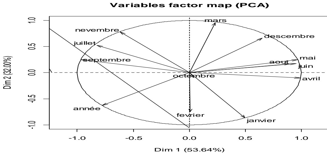
Figure 22 : Cercle de corrélation de l'ACP pour les ADM
