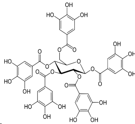
Figure (3) : esters D-glucose et de l'acide gallique
