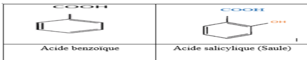
Types des acides benzoïques.
