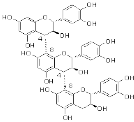
Figure (4) : polymère de tanins condensés.
