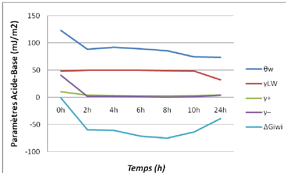
Graph 3 : évolution des paramètres physico-chimiques de la surface du bois de cèdre et de celle des Spores de P. chrytosum
