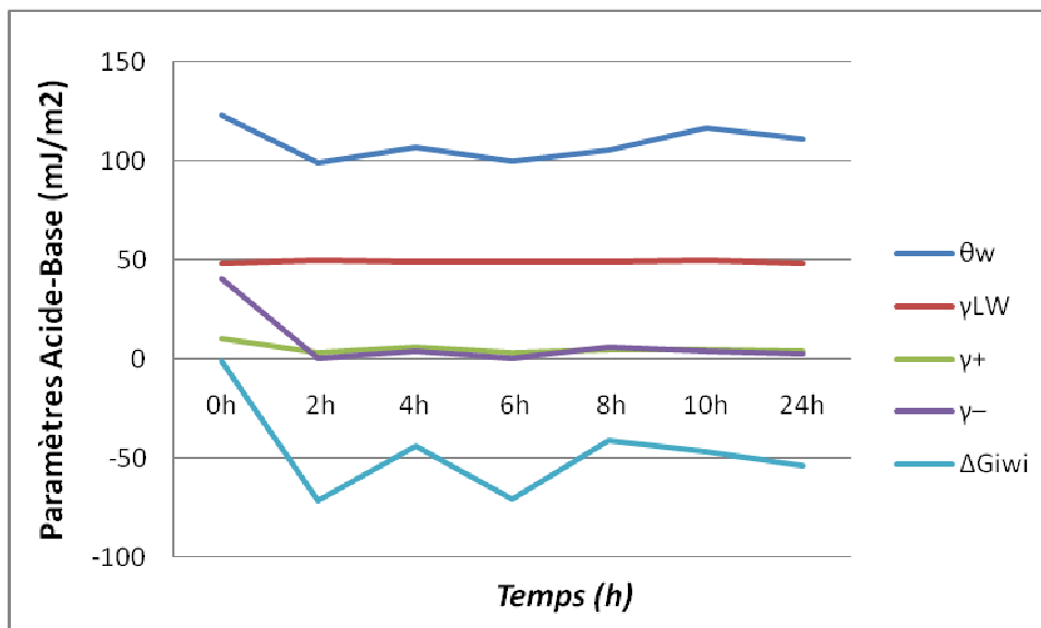
Graph 4 : évolution des paramètres physico-chimiques de la surface du bois de cèdre avec les Spores de P. commun
