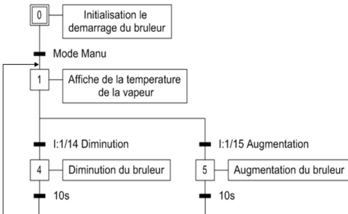
Figure 34 : Grafct de la régulation manuel
