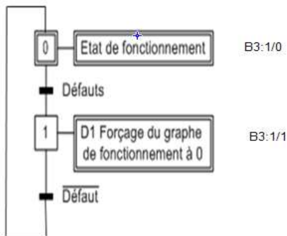
Figure 29 : Grafcet d'arrêt
