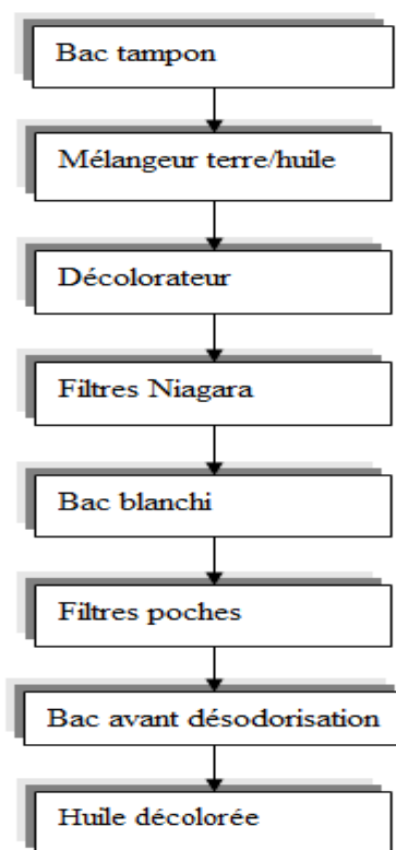
Figure 3 : diagramme de décoloration de : l'huile de soja
