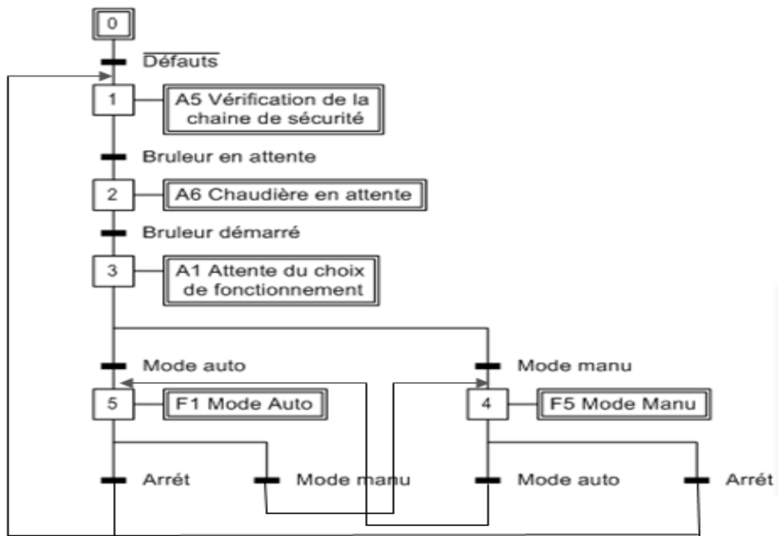
Figure 9 : Grafctet de mode de marche
