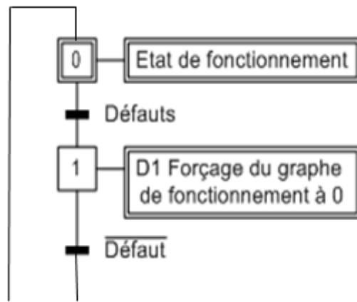
Figure 10 : Grafcet de mode d'arrêt
