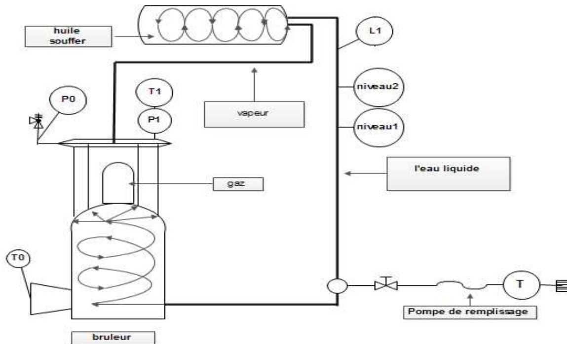
Figure 7 : Schémas de la station
