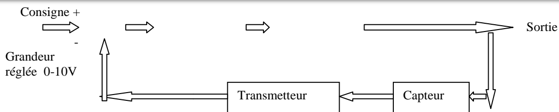
Figure 33 : Boucle de régulation industrielle
