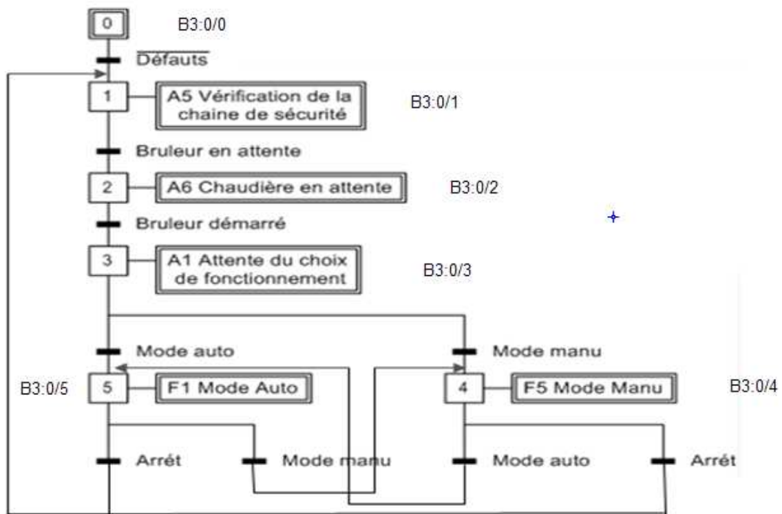
Figure 28 : Grafcet de fonctionnement
