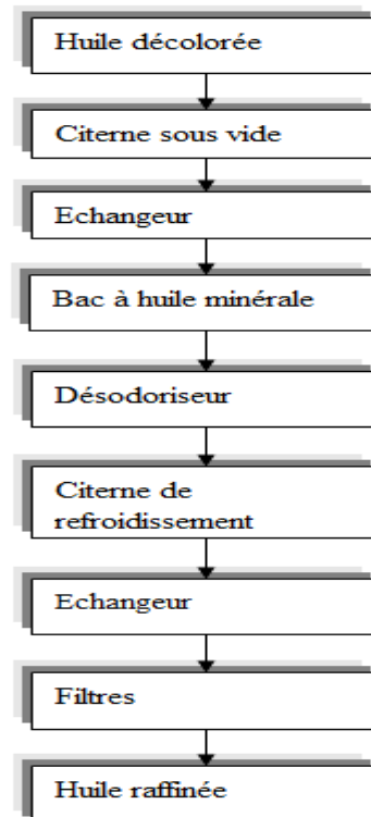
Figure 4 : diagramme de désodorisation de l'huile de soja
