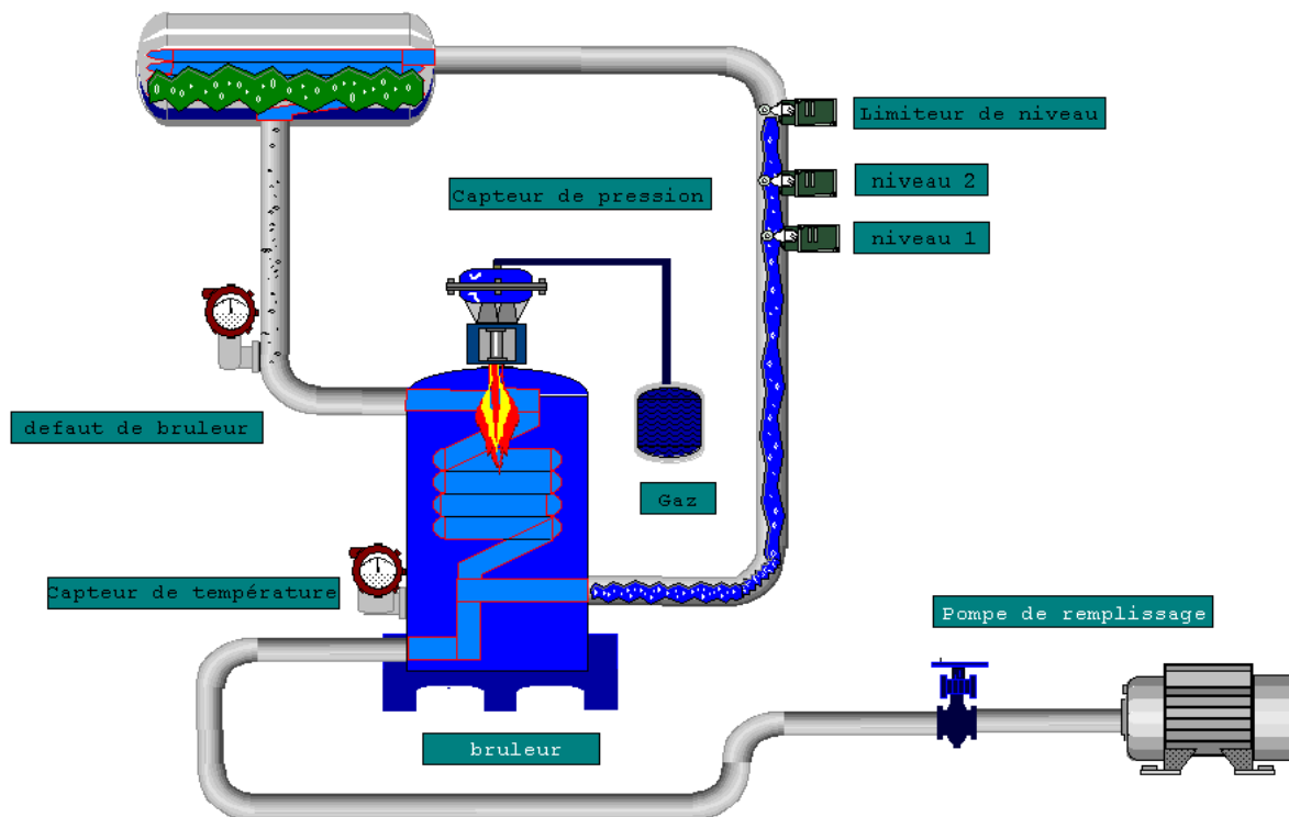
Figure 6 : Schémas de la station
