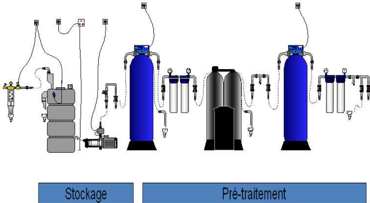
Figure 5 : La chaîne de traitement d'eau
