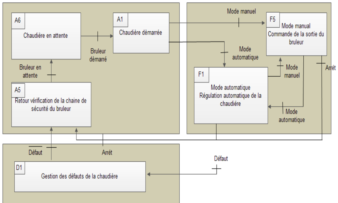
Figure 8 : GEMMA de la chaudière
