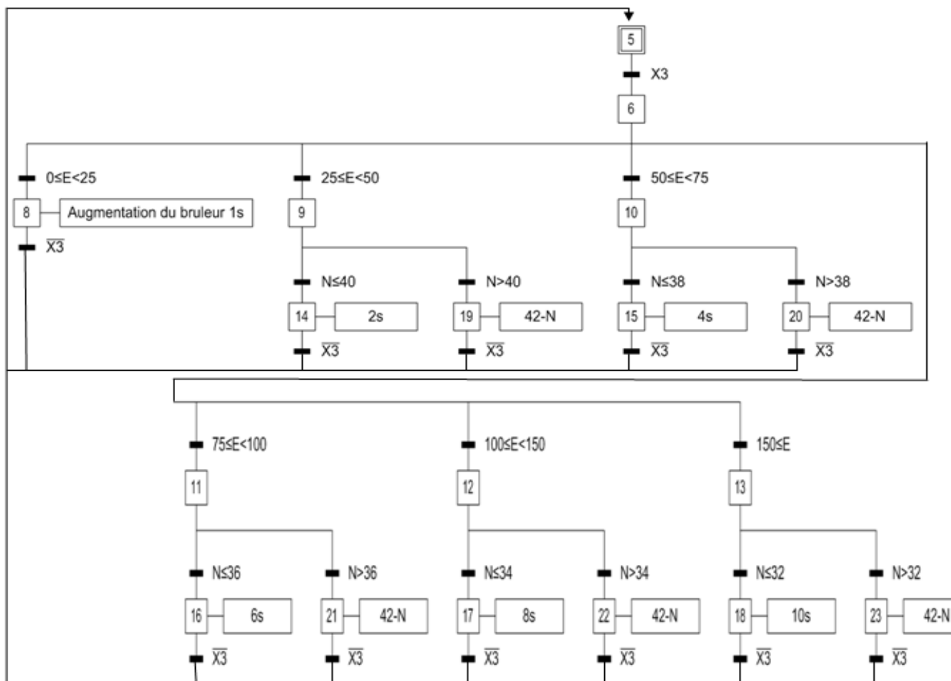
Figure 37 : Grafcet de la régulation automatique en augmentation
