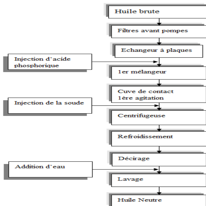
Figure 2 : diagramme de démucilagination et neutralisation de l'huile de soja
