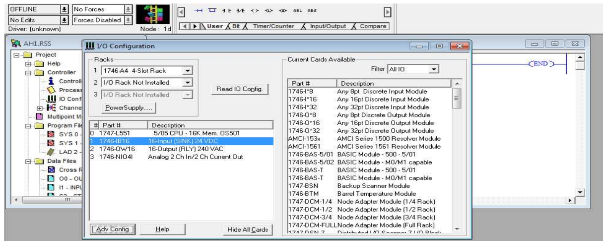
Figure 20 : configuration des E/S
